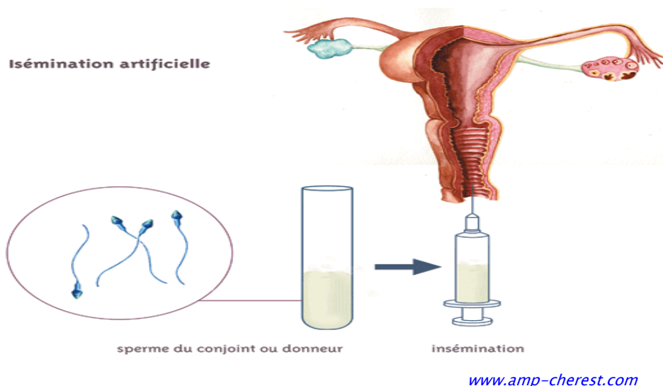
Figure 1 : L'insémination artificielle
