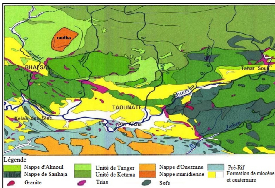
Figure 04 : Schéma structural du sud du Rif central
