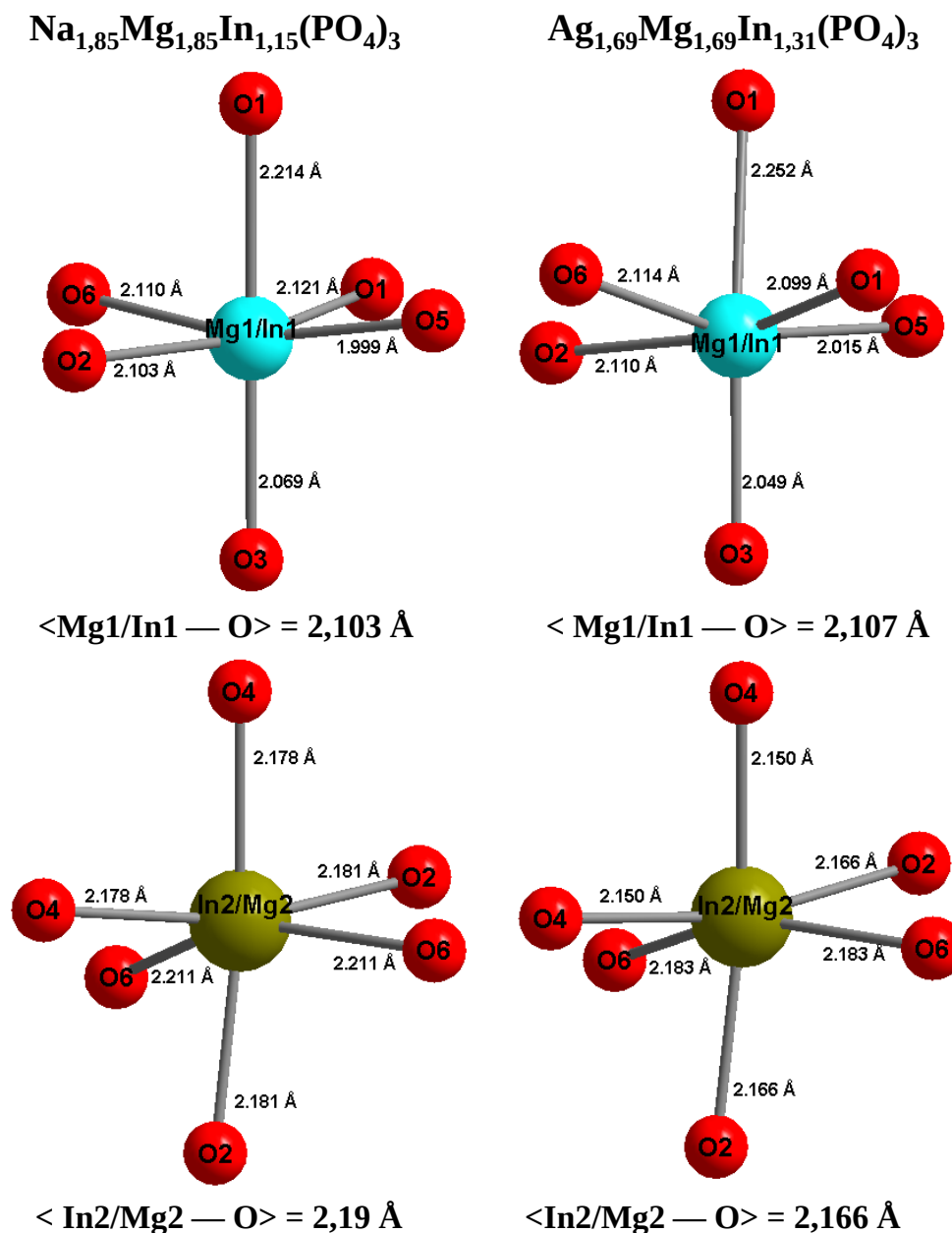
Figure V-23 : Environnement des ions Mg 2+ et In 3+ dans les sites Mg1/In1 et In2/Mg2 dans Na 1,85 Mg 1,85 In 1,15 (PO 4 ) 3 et Ag 1,69 Mg 1,69 In 1,31 (PO 4 ) 3
