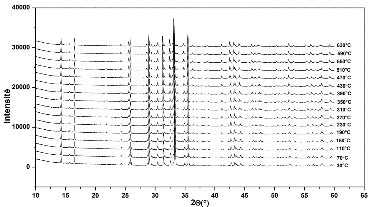
Figure V-16 : Diffractogrammes obtenus sur poudre en fonction de la température de \text{Na}_2\text{Mg}_2\text{Fe}(\text{PO}_4)_3
