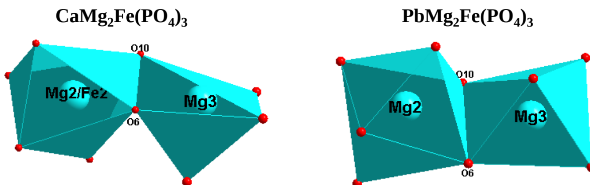
Figure III-16 : Entités \text{Mg}_2\text{Mg}_3\text{O}_9 et (\text{Mg}_2/\text{Fe}_2)\text{Mg}_3\text{O}_9 pour \text{MMg}_2\text{Fe}(\text{PO}_4)_3 (M = Ca, Pb)
