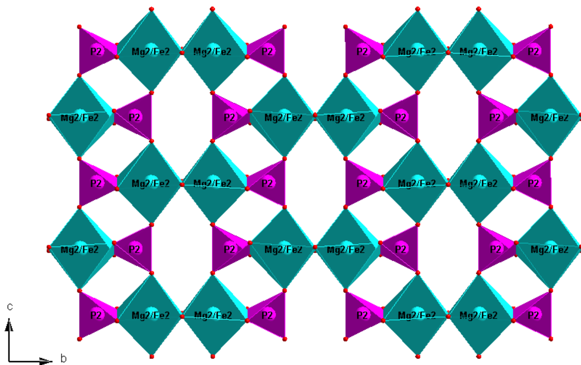
Figure III-7 : Feuillet (\text{Mg}_2/\text{Fe}_2)_4\text{P}_4\text{O}_{26} parallèle au plan (\vec{b}, \vec{c}) pour les composés \text{MMg}_2\text{Fe}(\text{PO}_4)_3 ( \text{M} = \text{Sr}, \text{Ba} )
