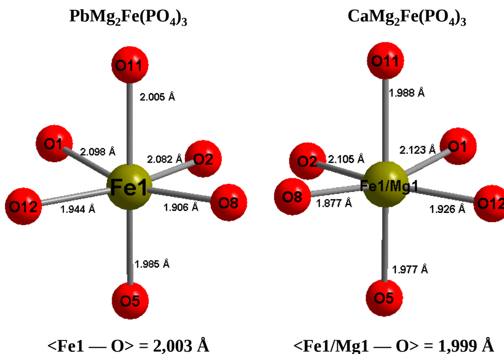
Figure III-13 : Environnement de l'ion \text{Fe}^{3+} dans les sites Fe1 et Fe1/Mg1 pour les composés \text{MMg}_2\text{Fe}(\text{PO}_4)_3 (M = Ca, Pb)
