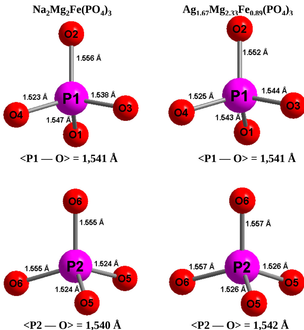
Figure V-1 : Environnement des ions \text{P}^{5+} dans les sites P1 et P2 pour \text{Na}_2\text{Mg}_2\text{Fe}(\text{PO}_4)_3 et \text{Ag}_{1,67}\text{Mg}_{2,33}\text{Fe}_{0,89}(\text{PO}_4)_3
