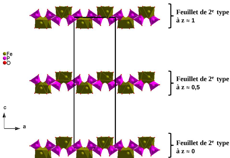
Figure III-35 : Projection des feuillets de 2 ème type dans le plan (\vec{a}, \vec{c}) pour \text{Ca}_2\text{MgFe}_2(\text{PO}_4)_4
