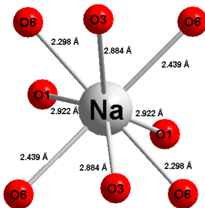
Figure IV-3 : Environnement de \text{Na}^+ dans le site Na pour \text{NaMg}_3(\text{HPO}_4)_2(\text{PO}_4)
