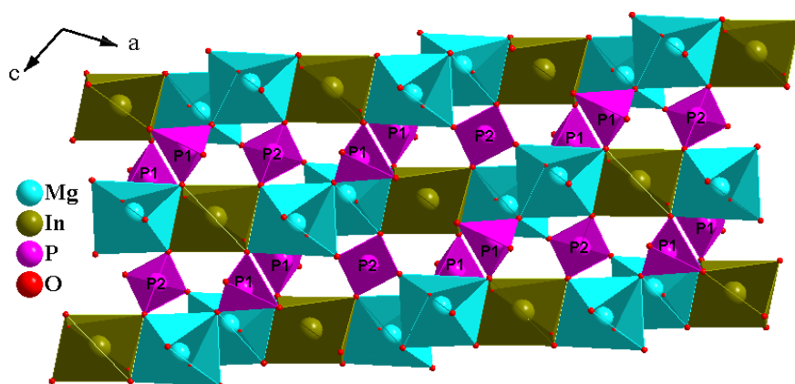
Figure V-26 : Feuillet parallèle au plan (\vec{a}, \vec{c}) pour \text{Na}_{1,85}\text{Mg}_{1,85}\text{In}_{1,15}(\text{PO}_4)_3 et \text{Ag}_{1,69}\text{Mg}_{1,69}\text{In}_{1,31}(\text{PO}_4)_3
