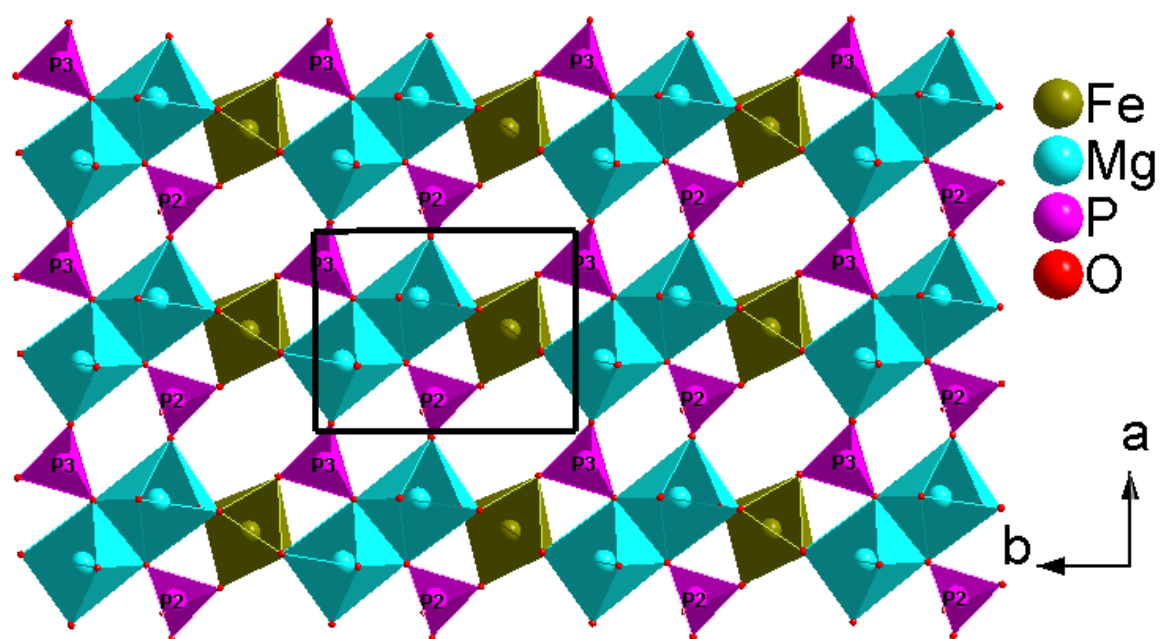
Figure III-19 : Projection des feuillets à z = 0,35 et à z = 0 dans le plan (\vec{a}, \vec{b}) pour \text{MMg}_2\text{Fe}(\text{PO}_4)_3 ( M = \text{Ca}, \text{Pb} )
