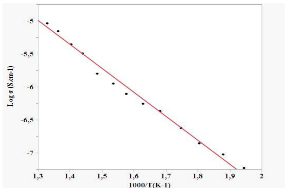
Figure V-21 : Evolution de la conductivité en fonction de la température pour \text{Na}_2\text{Mg}_2\text{Fe}(\text{PO}_4)_3
