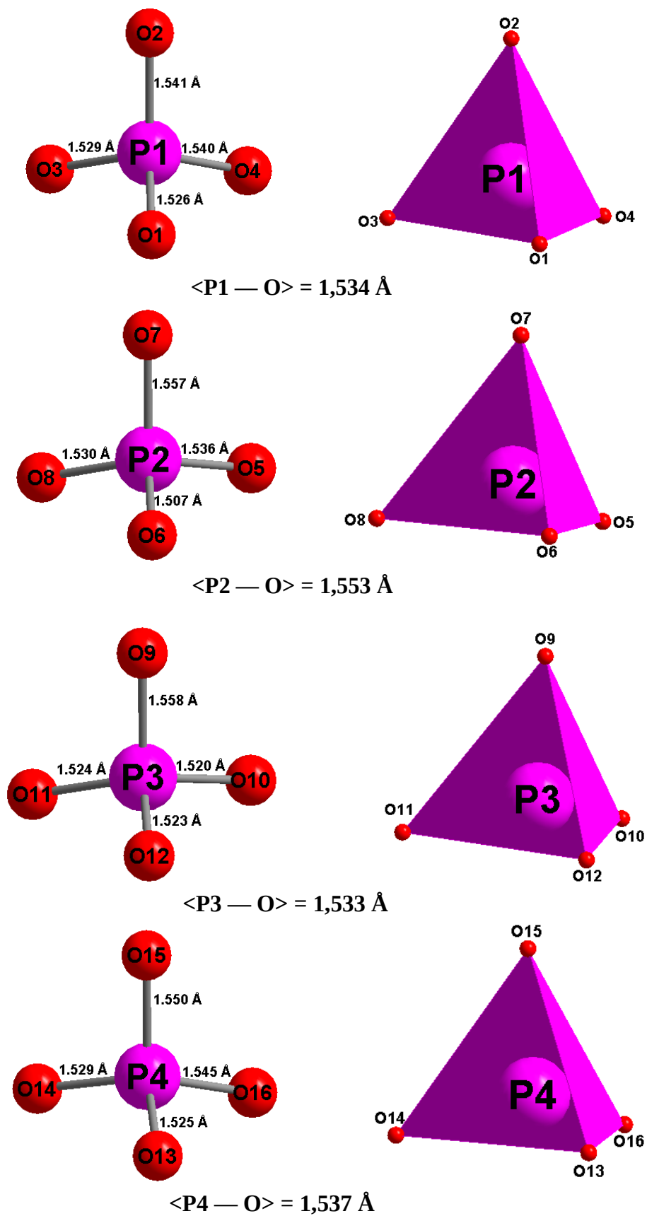
Figure III-25 : Environnement de l'ion P^{5+} dans les sites P1, P2, P3 et P4 pour Ca_2MgFe_2(PO_4)_4
