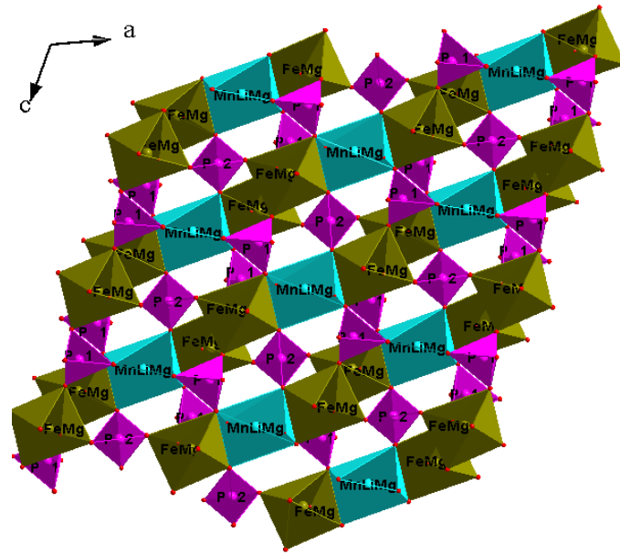
Figure I-12 : Feuille parallèle au plan (\vec{a}, \vec{c})
