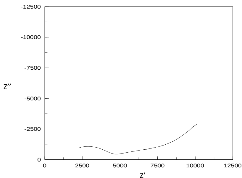
Figure V-18 : Impédance complexe de Ag_2Mg_2Fe(PO_4)_3
