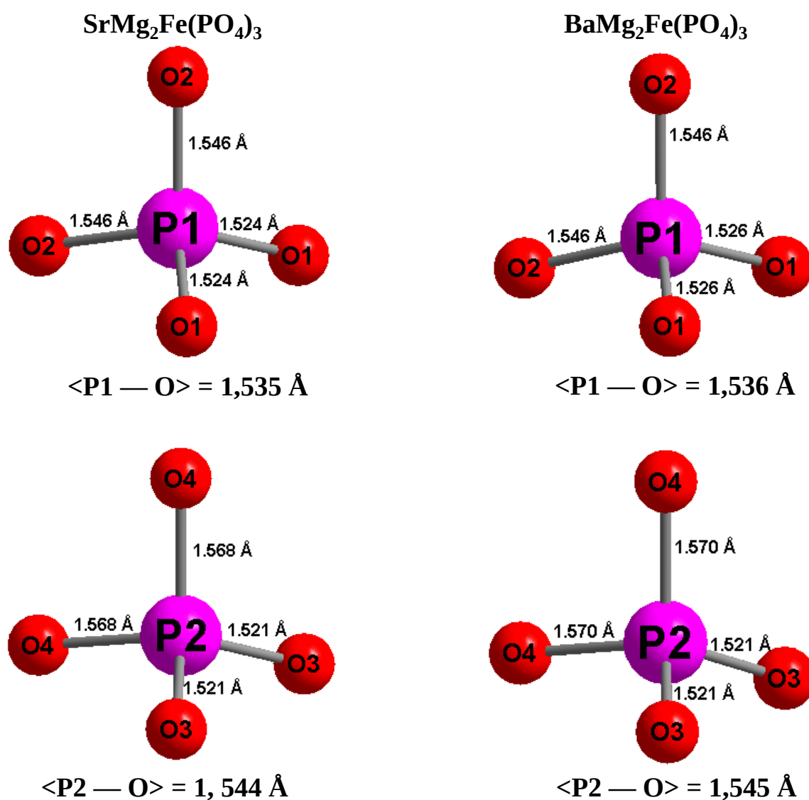
Figure III-1 : Environnement des ions \text{P}^{5+} dans les sites P1 et P2 dans les composés \text{MMg}_2\text{Fe}(\text{PO}_4)_3 ( \text{M} = \text{Sr}, \text{Ba} )
