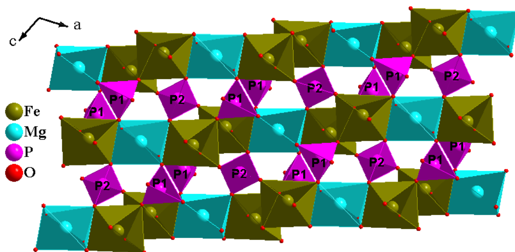
Figure V-8 : Feuillet parallèle au plan (\vec{a}, \vec{c}) pour \text{Na}_2\text{Mg}_2\text{Fe}(\text{PO}_4)_3 et \text{Ag}_{1,67}\text{Mg}_{2,33}\text{Fe}_{0,89}(\text{PO}_4)_3
