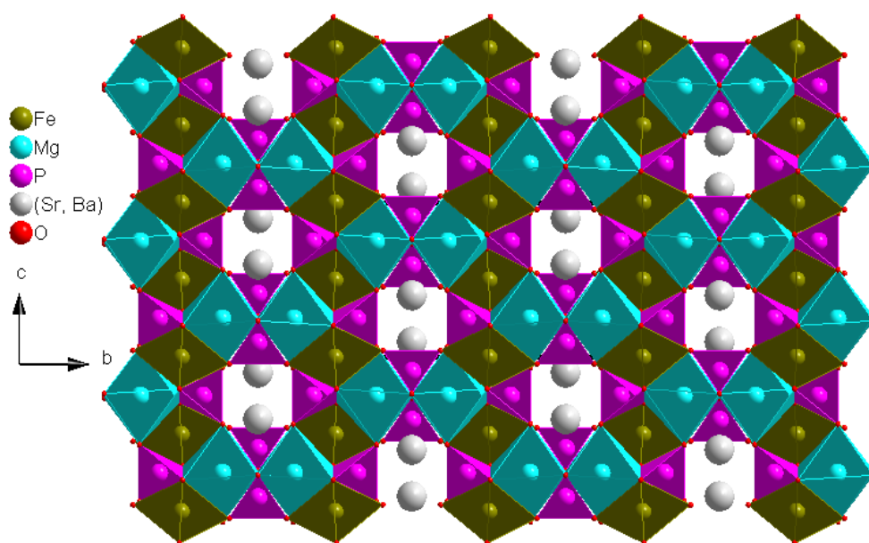
Figure III-11 : Projection de la structure MMg_2Fe(PO_4)_3 ( M = Sr, Ba ) dans le plan (\vec{b}, \vec{c})
