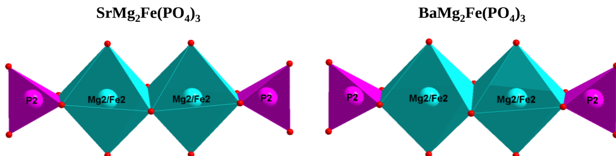
Figure III-6 : Entité (\text{Mg}_2/\text{Fe}_2)_2\text{P}_2\text{O}_{14} pour les composés \text{MMg}_2\text{Fe}(\text{PO}_4)_3 ( \text{M} = \text{Sr}, \text{Ba} )
