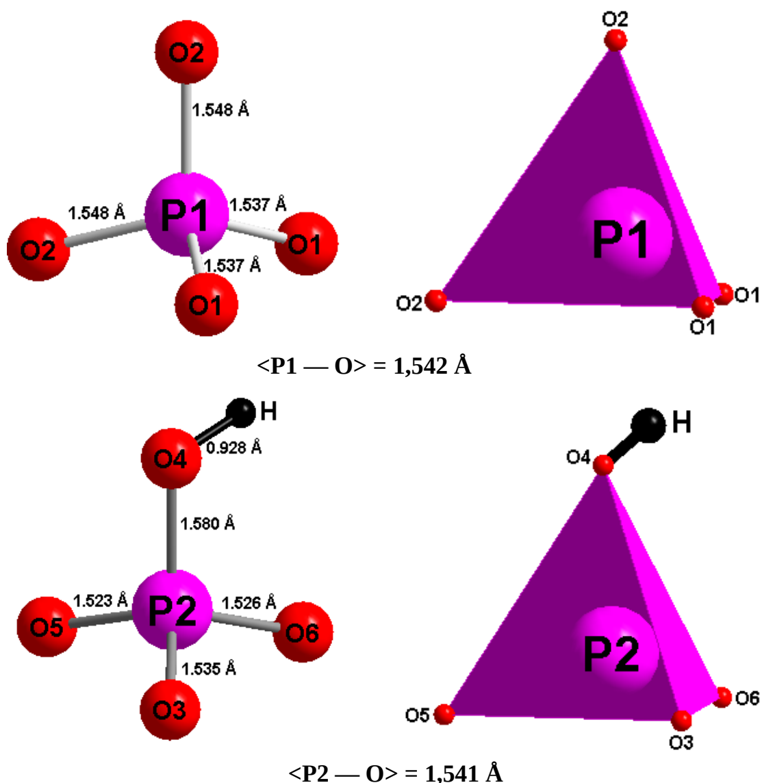
Figure IV-1 : Environnement des ions P^{5+} dans les sites P1 et P2 pour NaMg_3(HPO_4)_2(PO_4)
