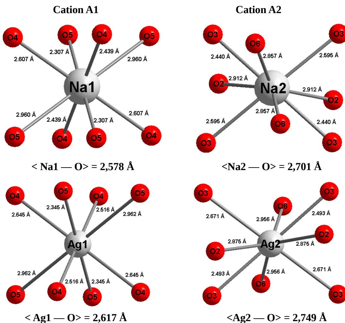
Figure V-24 : Environnement des ions \text{Na}^+ dans les sites Na1 et Na2 et des ions \text{Ag}^+ dans les sites Ag1 et Ag2 dans \text{Na}_{1,85}\text{Mg}_{1,85}\text{In}_{1,15}(\text{PO}_4)_3 et \text{Ag}_{1,69}\text{Mg}_{1,69}\text{In}_{1,31}(\text{PO}_4)_3
