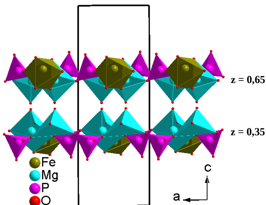
Figure III-21 : Projection des feuillets à z = 0,35 et à z = 0,65 dans le plan (\vec{a}, \vec{c}) pour \text{MMg}_2\text{Fe}(\text{PO}_4)_3 ( M = \text{Ca}, \text{Pb} )
