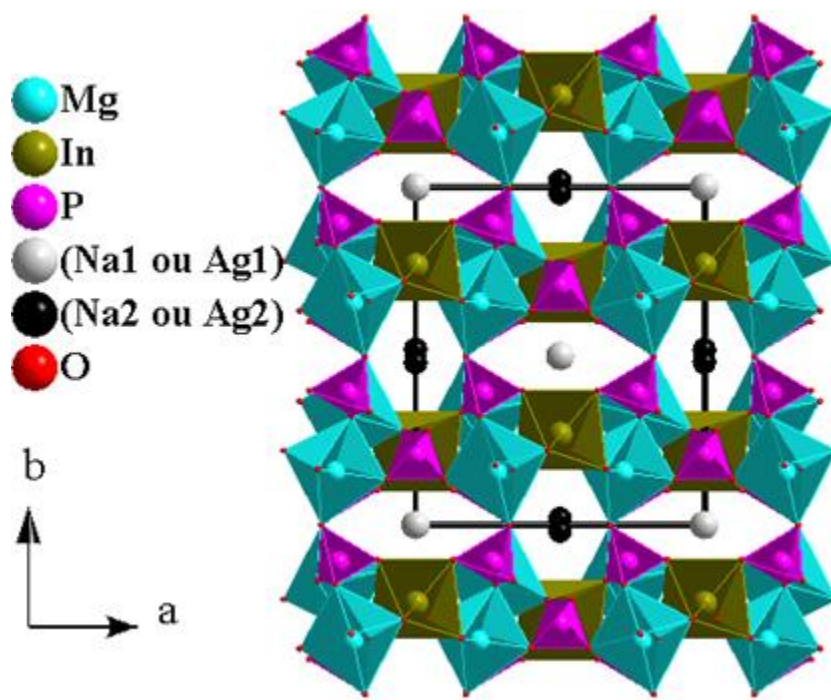
Figure V-27 : Projection de la structure de \text{Na}_{1,85}\text{Mg}_{1,85}\text{In}_{1,15}(\text{PO}_4)_3 et de \text{Ag}_{1,69}\text{Mg}_{1,69}\text{In}_{1,31}(\text{PO}_4)_3 dans le plan (\vec{a}, \vec{b})
