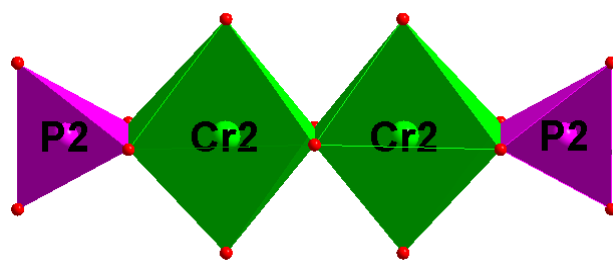
Figure I-8 : Entité \text{Cr}_2\text{P}_2\text{O}_{14}
