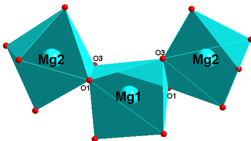
Figure IV-4 : Trimère \text{Mg}(2)_2\text{Mg}(1)\text{O}_{14} pour \text{NaMg}_3(\text{HPO}_4)_2(\text{PO}_4)
