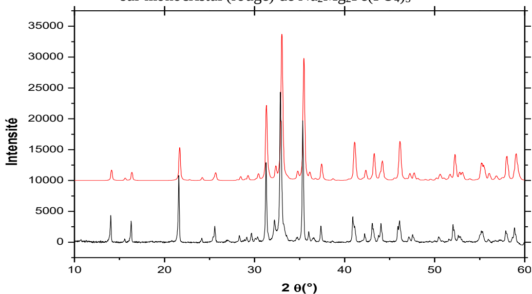
Figure V-11 : Diagramme de diffraction X expérimental (noir) et calculé à partir des données sur monocristal (rouge) de \text{Ag}_2\text{Mg}_2\text{Fe}(\text{PO}_4)_3
