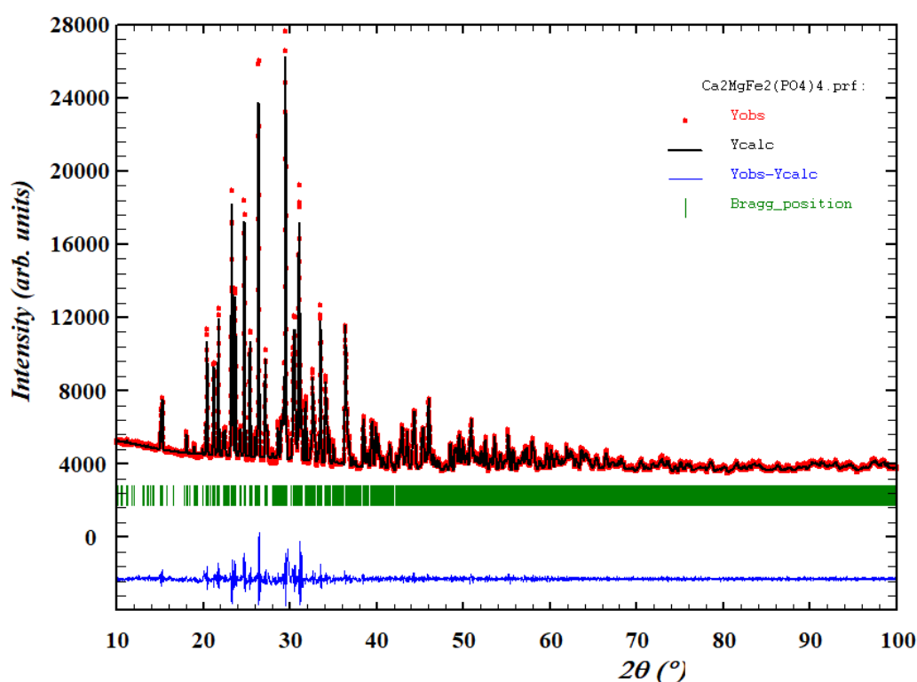
Figure III-37 : Diffractogrammes calculé, observé et différence pour \text{Ca}_2\text{MgFe}_2(\text{PO}_4)_4
