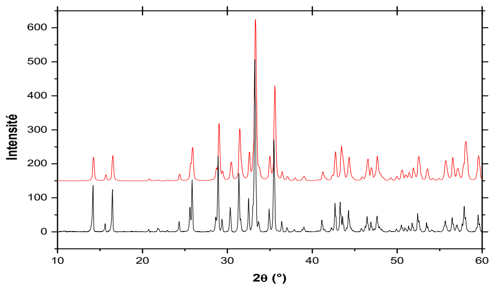
Figure V-10 : Diagrammes de diffraction X expérimental (noir) et calculé à partir des données sur monocristal (rouge) de \text{Na}_2\text{Mg}_2\text{Fe}(\text{PO}_4)_3
