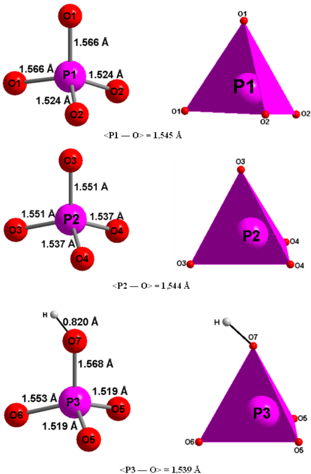
Figure II-1 : Environnement des ions \text{P}^{5+} dans les sites P1, P2 et P3 pour \text{PbMg}_3(\text{HPO}_4)(\text{PO}_4)_2
