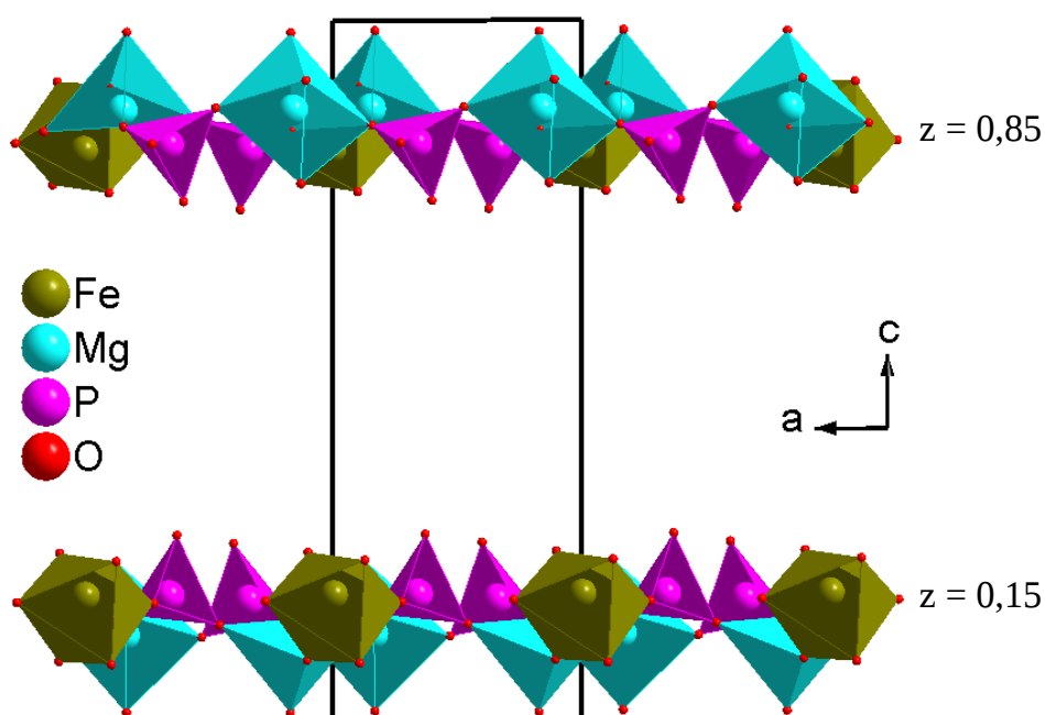
Figure III-20 : Projection des feuillets à z = 0,15 et à z = 0,85 dans le plan (\vec{a}, \vec{c}) pour \text{MMg}_2\text{Fe}(\text{PO}_4)_3 ( M = \text{Ca}, \text{Pb} )
