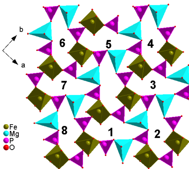
Figure III-30 : Premier type de feuillet dans le plan (\vec{a}, \vec{b}) pour Ca_2MgFe_2(PO_4)_4
