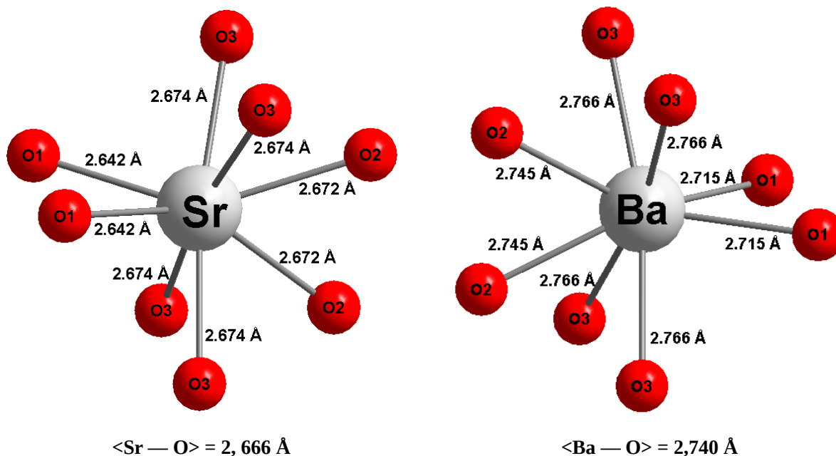
Figure III-4 : Environnement du cation M dans le site Sr/Ba pour les composés \text{MMg}_2\text{Fe}(\text{PO}_4)_3 (M = Sr, Ba)
