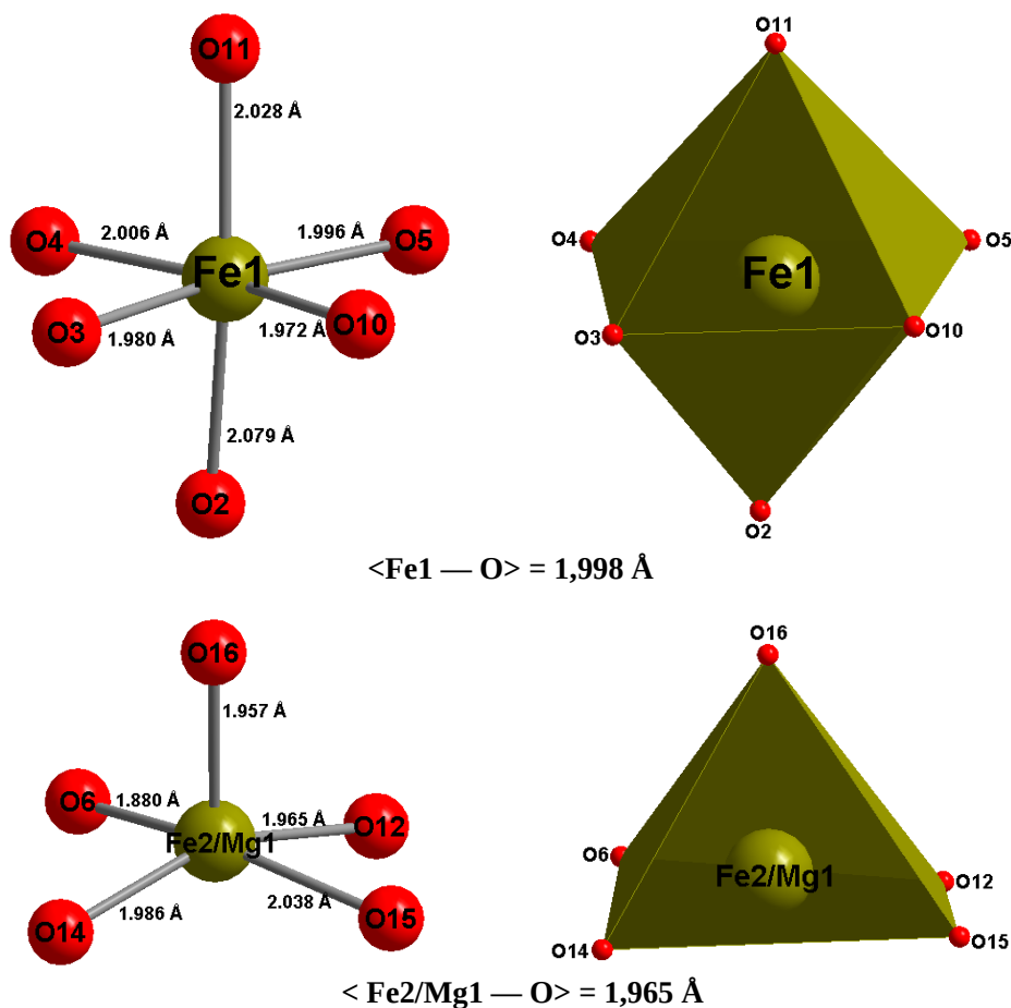
Figure III-26 : Environnement des ions Fe^{3+} et de Mg^{2+} dans les sites Fe1 et Fe2/Mg1 pour Ca_2MgFe_2(PO_4)_4
