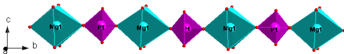
Figure II-6 : Représentation de la chaîne \text{Mg}_1\text{P}_1\text{O}_9 suivant l'axe \vec{b} pour \text{PbMg}_3(\text{HPO}_4)(\text{PO}_4)_2
