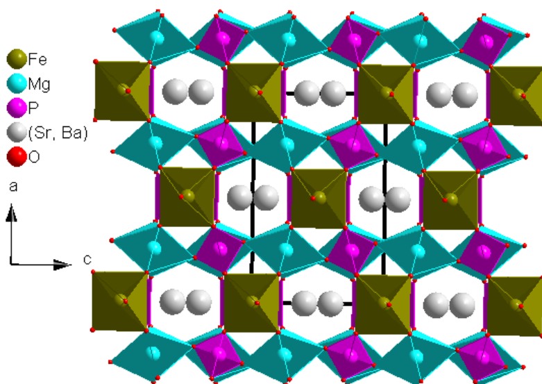
Figure III-10 : Projection de la structure MMg_2Fe(PO_4)_3 ( M = Sr, Ba ) dans le plan (\vec{a}, \vec{c})
