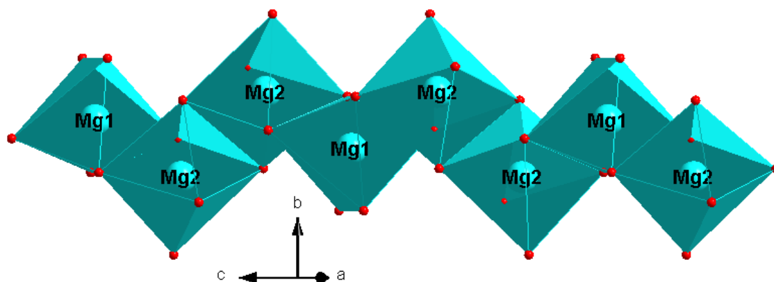
Figure IV-5 : Chaîne infinie (\text{Mg}_2\text{Mg}_1\text{O}_{14})_\infty suivant la rangée [101] pour \text{NaMg}_3(\text{HPO}_4)_2(\text{PO}_4)
