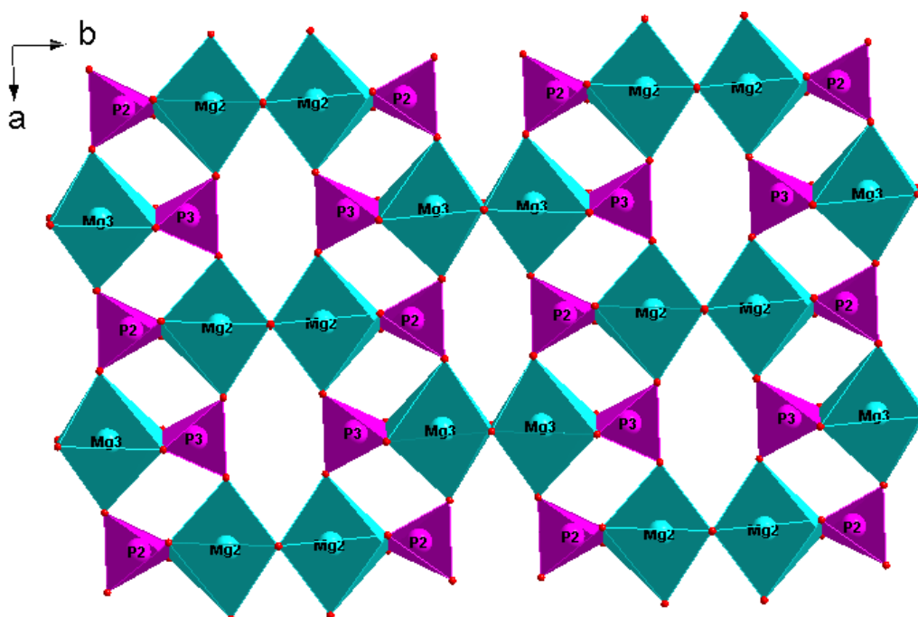
Figure II-5 : Représentation du feuillet \text{Mg}_4\text{P}_4\text{O}_{26} parallèle au plan (\vec{a}, \vec{b}) pour \text{PbMg}_3(\text{HPO}_4)(\text{PO}_4)_2
