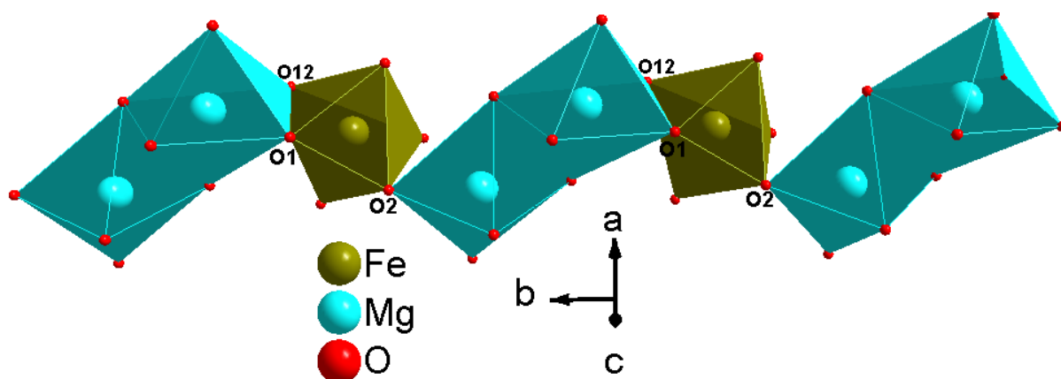
Figure III-17 : Représentation de la chaîne en zigzag suivant [0\ 1\ 0] pour \text{MMg}_2\text{Fe}(\text{PO}_4)_3 ( \text{M} = \text{Ca}, \text{Pb} )
