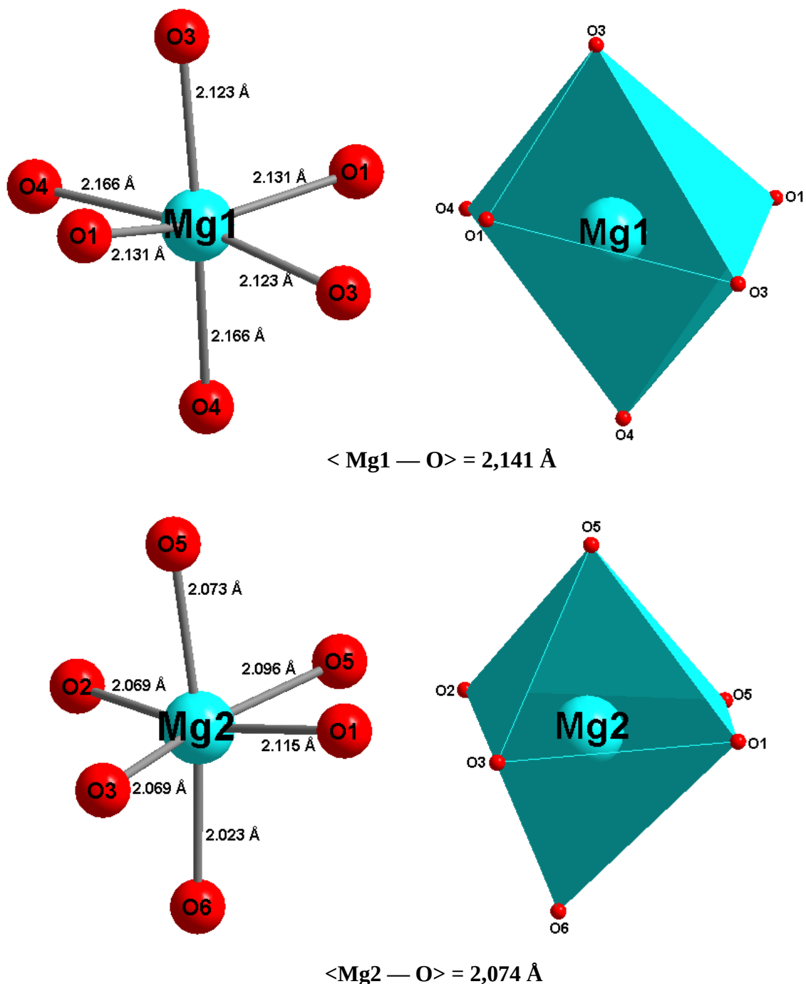
Figure IV-2 : Environnement des ions \text{Mg}^{2+} dans les sites Mg1 et Mg2 pour \text{NaMg}_3(\text{HPO}_4)_2(\text{PO}_4)
