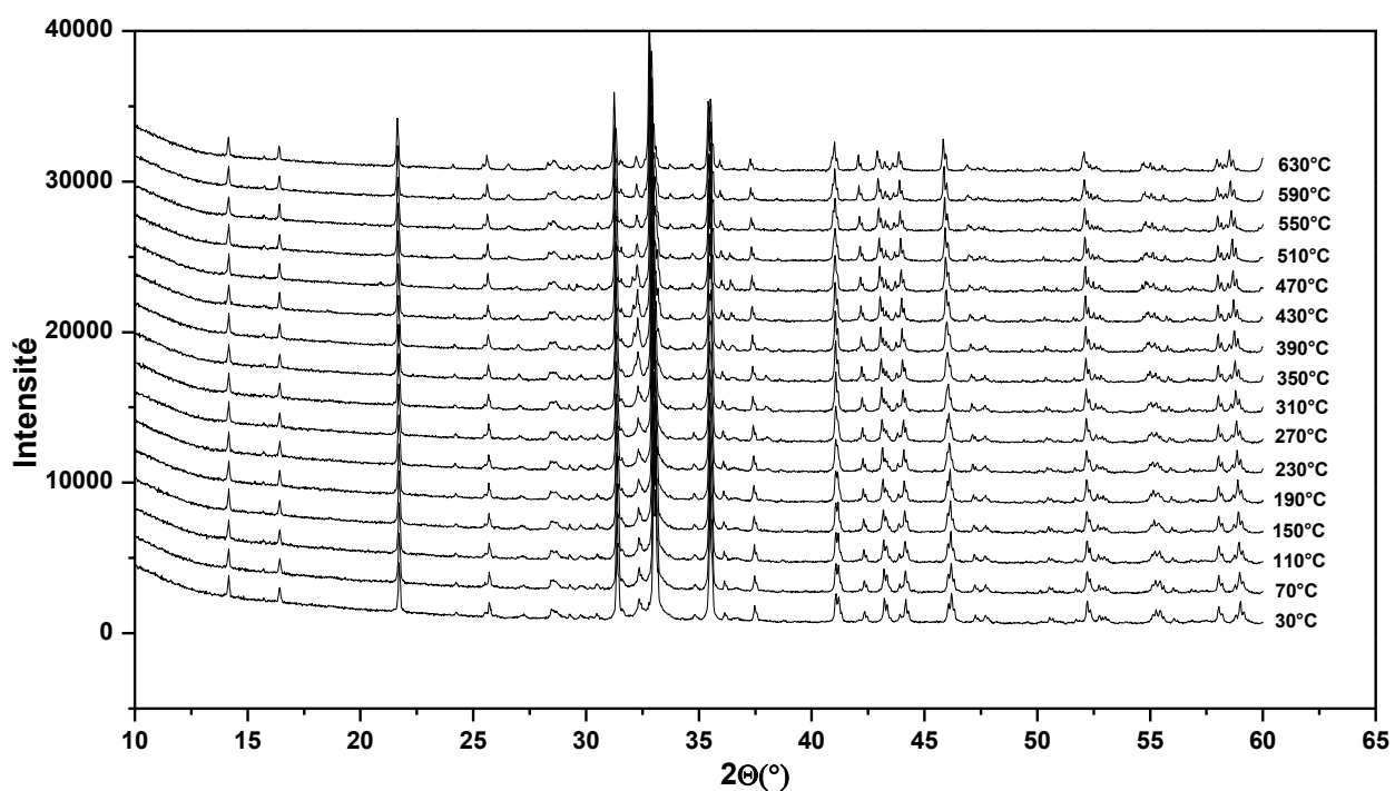
Figure V-17 : Diffractogrammes obtenus sur poudre en fonction de la température de \text{Ag}_2\text{Mg}_2\text{Fe}(\text{PO}_4)_3
