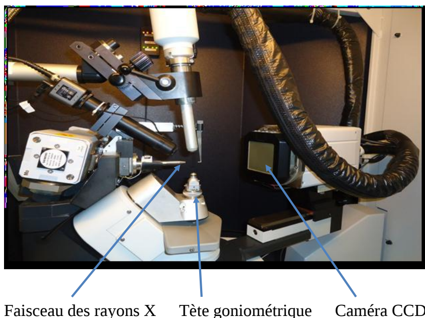
Figure 4 : Diffractomètre automatique à quatre cercles Bruker X8
