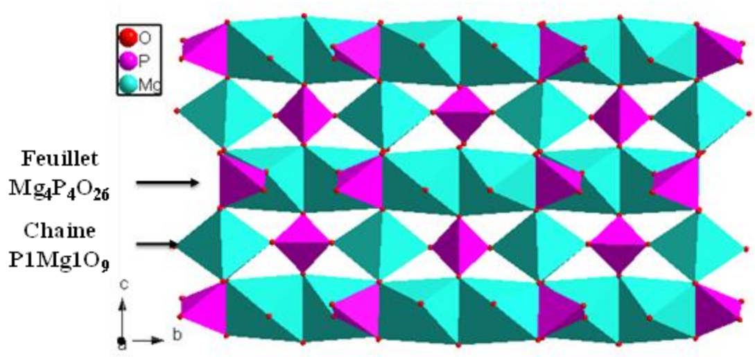
Figure II-7 : Représentation de la jonction entre les chaînes \text{Mg}_1\text{P}_1\text{O}_9 et les feuillets \text{Mg}_4\text{P}_4\text{O}_{26} pour \text{PbMg}_3(\text{HPO}_4)(\text{PO}_4)_2
