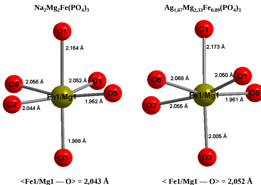
Figure V-2 : Environnement des ions \text{Fe}^{3+} et \text{Mg}^{2+} dans le site Fe1/Mg1 pour \text{Na}_2\text{Mg}_2\text{Fe}(\text{PO}_4)_3 et \text{Ag}_{1,67}\text{Mg}_{2,33}\text{Fe}_{0,89}(\text{PO}_4)_3
