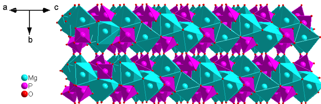
Figure IV-7 : Connexion des feuillets via les sommets de P_2O_4 et de Mg_2O_6 pour NaMg_3(HPO_4)_2(PO_4)
