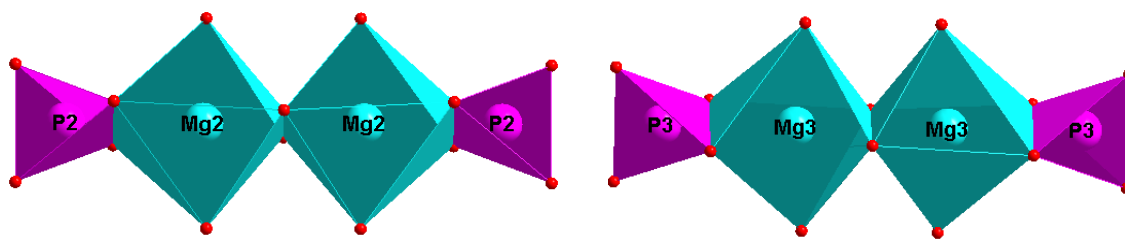
Figure II-4 : Représentation des entités \text{Mg}_2\text{P}_2\text{O}_{14} et \text{Mg}_3\text{P}_3\text{O}_{14} pour \text{PbMg}_3(\text{HPO}_4)(\text{PO}_4)_2
