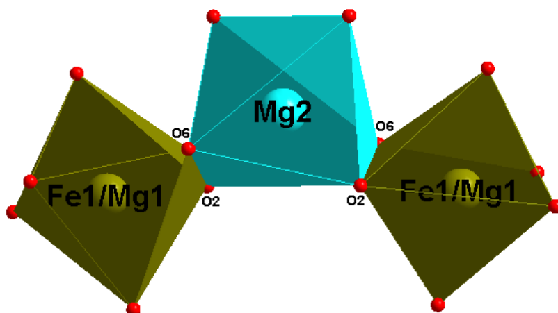
Figure V-6 : Entité (\text{Fe1/Mg1})_2\text{Mg2O}_{14} pour \text{Na}_2\text{Mg}_2\text{Fe}(\text{PO}_4)_3 et \text{Ag}_{1,67}\text{Mg}_{2,33}\text{Fe}_{0,89}(\text{PO}_4)_3
