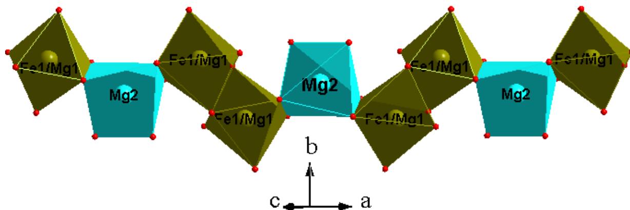
Figure V-7 : Chaîne infinie [(\text{Fe1/Mg1})_2\text{Mg2O}_{14}]_\infty suivant la rangée [101] pour \text{Na}_2\text{Mg}_2\text{Fe}(\text{PO}_4)_3 et \text{Ag}_{1,67}\text{Mg}_{2,33}\text{Fe}_{0,89}(\text{PO}_4)_3
