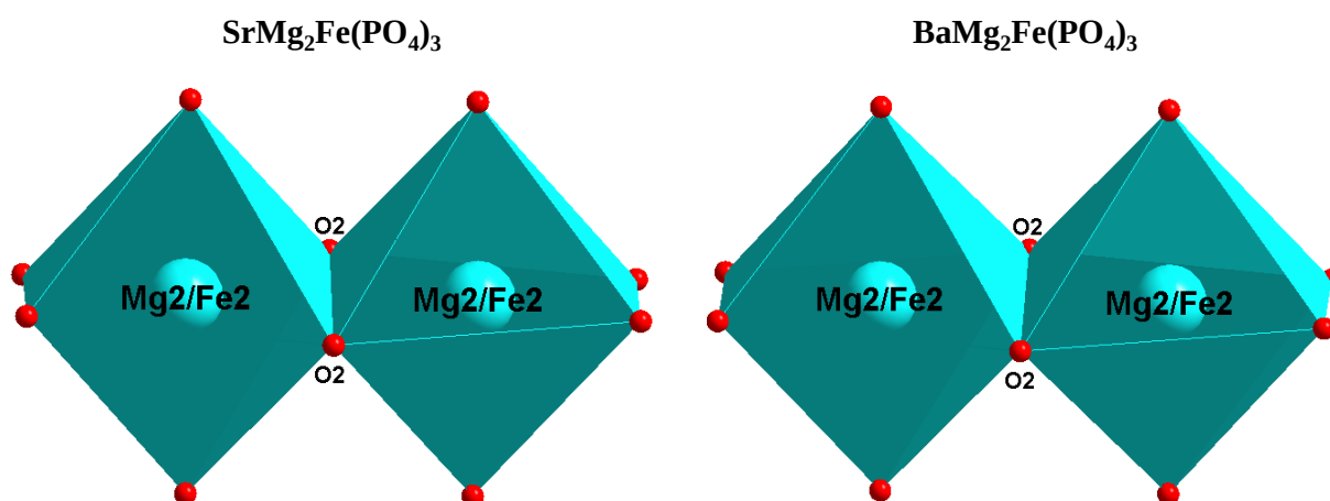
Figure III-5 : Dimères (\text{Mg}_2/\text{Fe}_2)_2\text{O}_{10} pour les composés \text{MMg}_2\text{Fe}(\text{PO}_4)_3 (M = Sr, Ba)
