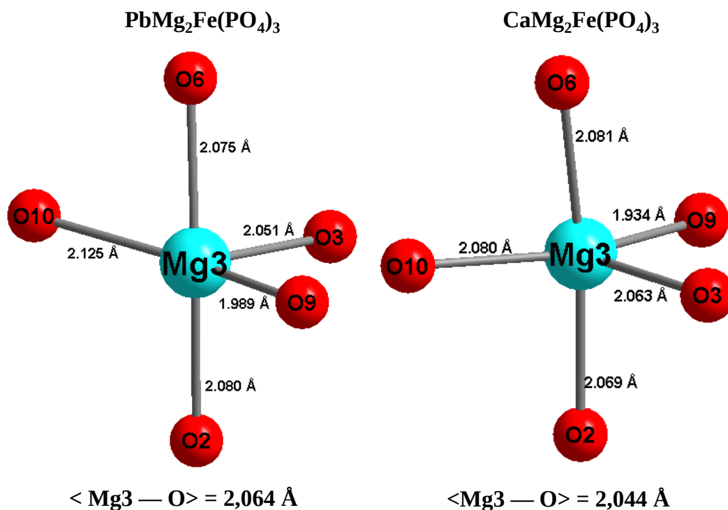
Figure III-15 : Environnement des ions \text{Mg}^{2+} dans le site Mg3 pour les composés \text{MMg}_2\text{Fe}(\text{PO}_4)_3 (M = Ca, Pb)
