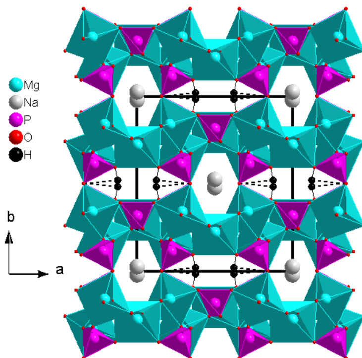
Figure IV-8 : Projection de la structure de NaMg_3(HPO_4)_2(PO_4) dans le plan (\vec{a}, \vec{b})
