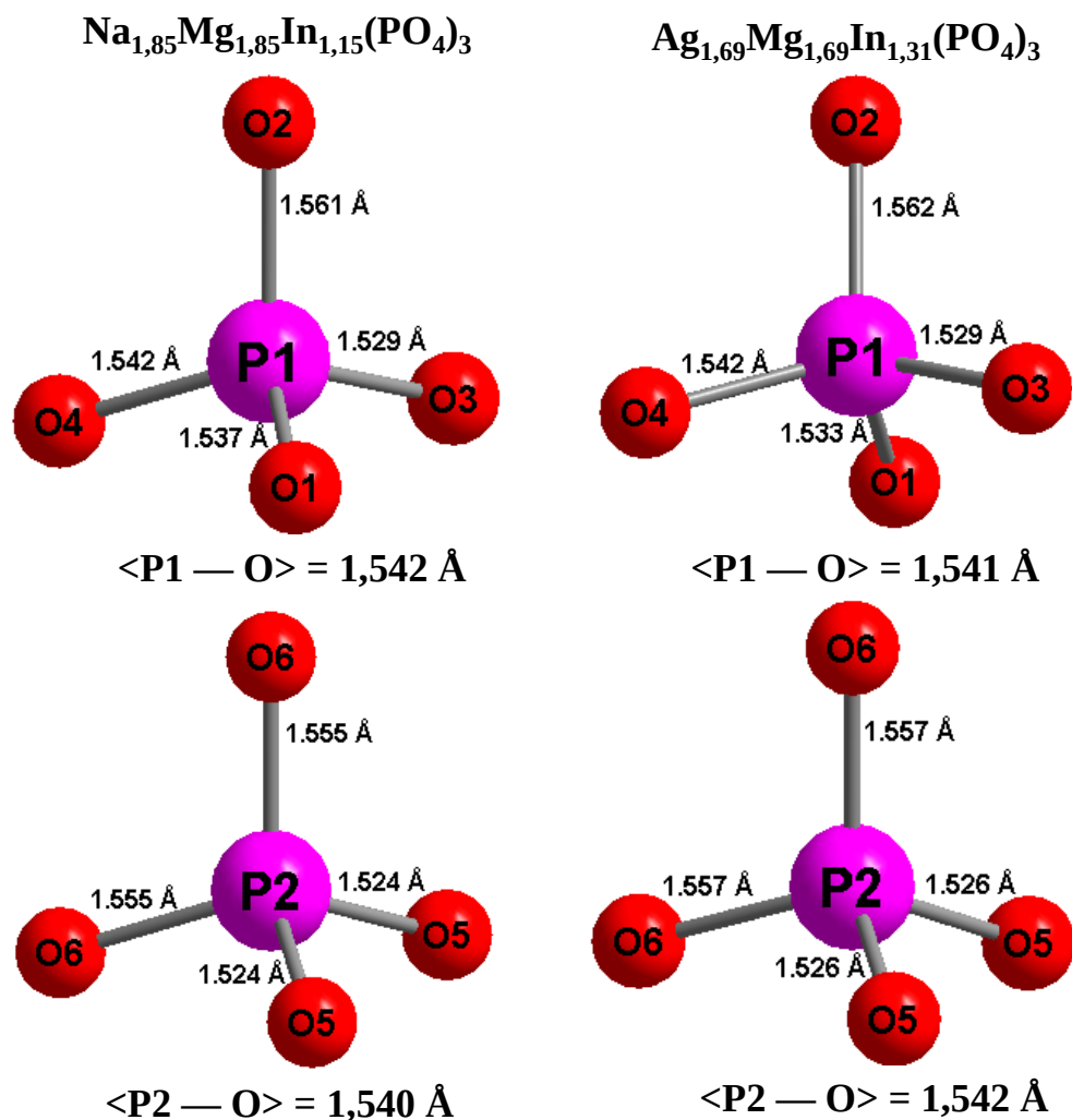
Figure V-22 : Environnement de l'ion P 5+ dans les sites P1 et P2 pour Na 1,85 Mg 1,85 In 1,15 (PO 4 ) 3 et Ag 1,69 Mg 1,69 In 1,31 (PO 4 ) 3
