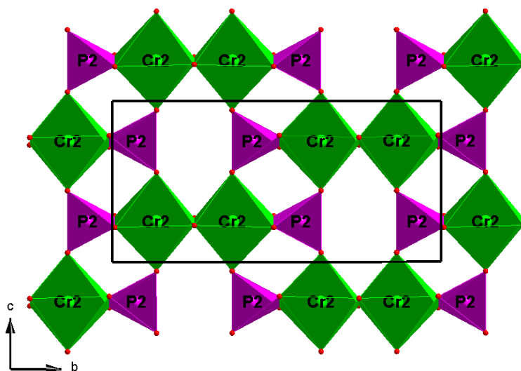
Figure I-9 : Feuillet \text{Cr}_2\text{P}_2\text{O}_{14} dans le plan (\vec{b}, \vec{c})
