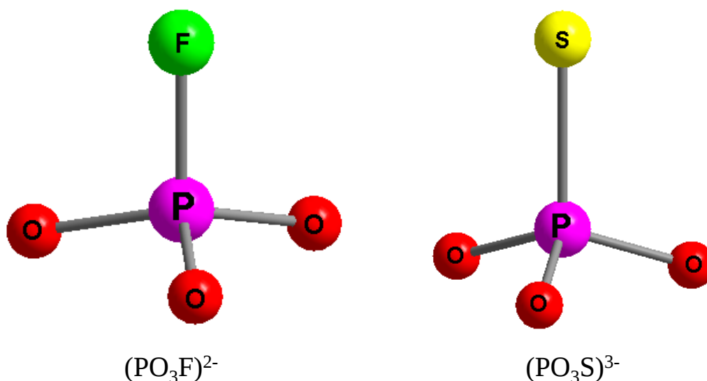
Figure I-2 : Monophosphates d'anions substitués \text{Ag}_2\text{PO}_3\text{F} [26] et \text{NaSr}[\text{PO}_3\text{S}], 9\text{H}_2\text{O} [27]
