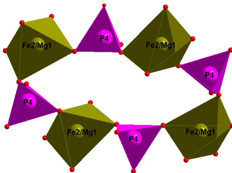
Figure III-31 : Deuxième type d'anneau formé par les polyèdres P_4O_4-(Fe_2/Mg_1)O_6 pour Ca_2MgFe_2(PO_4)_4
