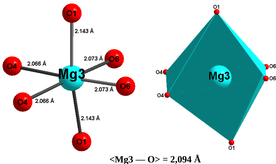
Figure II-2 : Environnement des ions \text{Mg}^{2+} dans les sites Mg1, Mg2 et Mg3 pour \text{PbMg}_3(\text{HPO}_4)(\text{PO}_4)_2
