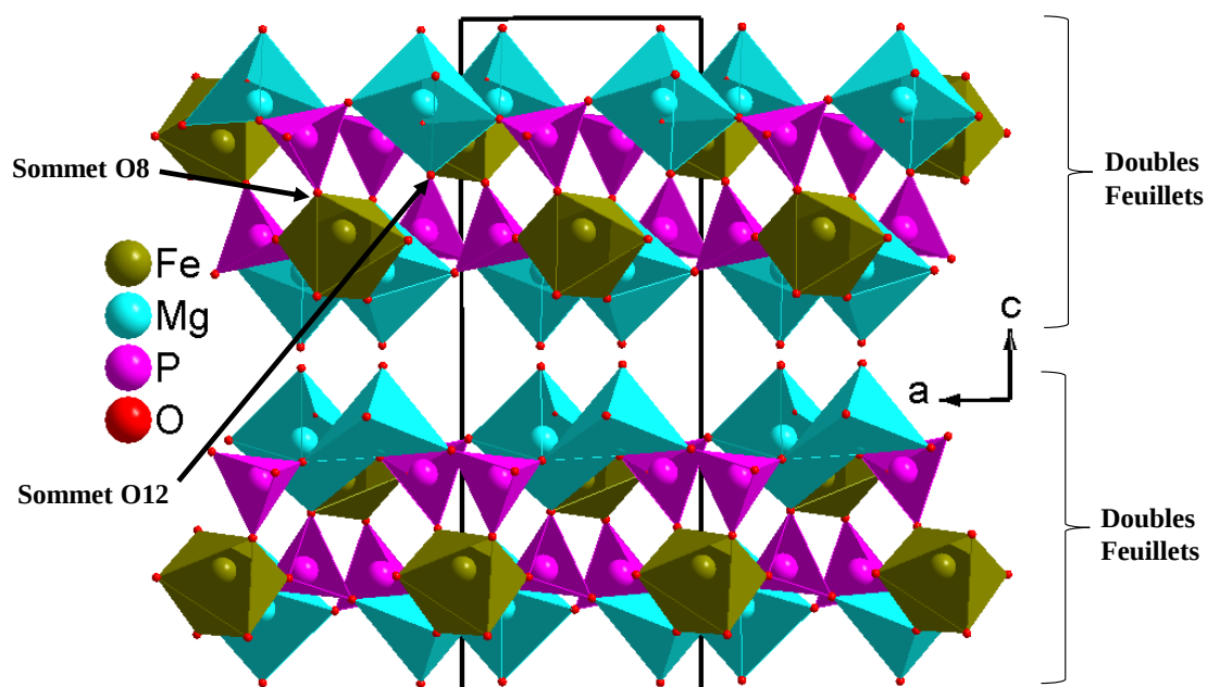
Figure III-22 : Projection des doubles feuillets dans le plan (\vec{a}, \vec{c}) pour \text{MMg}_2\text{Fe}(\text{PO}_4)_3 ( M = \text{Ca}, \text{Pb} )
