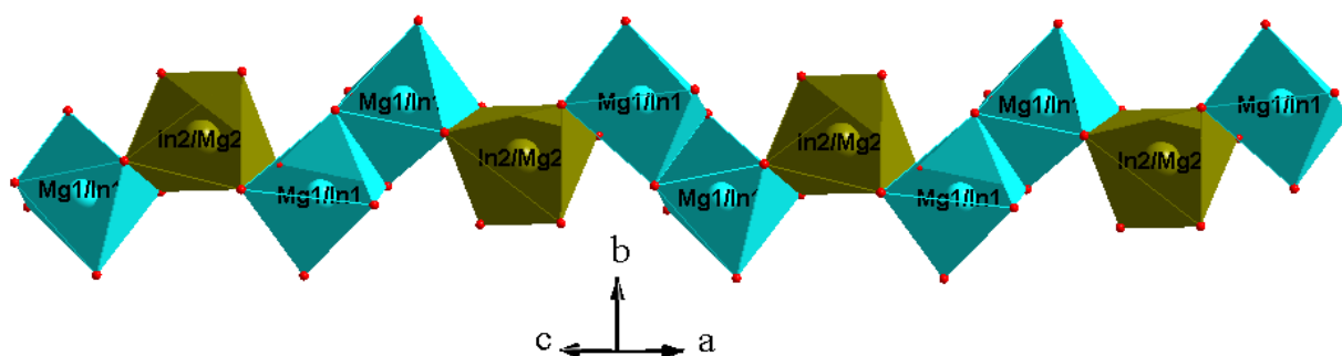
Figure V-25 : Chaînes infinie suivant [101] pour \text{Na}_{1,85}\text{Mg}_{1,85}\text{In}_{1,15}(\text{PO}_4)_3 et \text{Ag}_{1,69}\text{Mg}_{1,69}\text{In}_{1,31}(\text{PO}_4)_3
