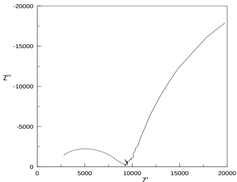
Figure V-20 : Impédance complexe de \text{Na}_2\text{Mg}_2\text{Fe}(\text{PO}_4)_3
