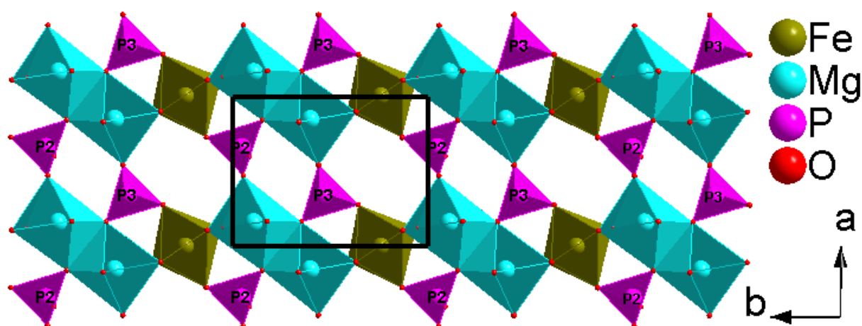
Figure III-18 : Projection des feuillets à z = 0,15 et à z = 0,85 dans le plan (\vec{a}, \vec{b}) pour \text{MMg}_2\text{Fe}(\text{PO}_4)_3 ( \text{M} = \text{Ca}, \text{Pb} )
