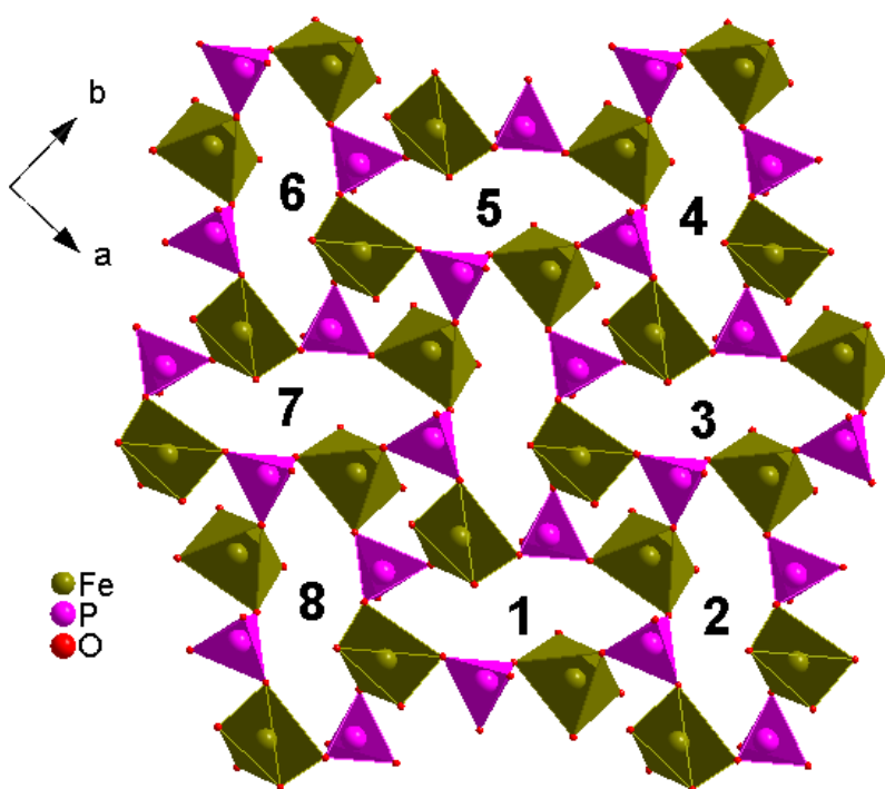
Figure III-32 : Deuxième type de feuillet dans le plan (\vec{a}, \vec{b}) pour Ca_2MgFe_2(PO_4)_4
