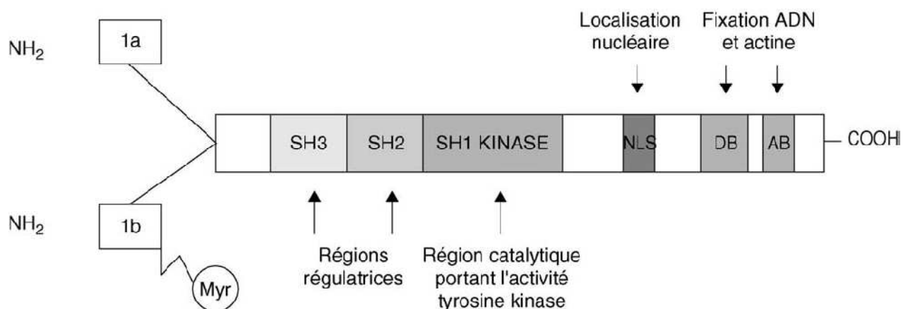
Figure 8 : représentation schématique de la protéine Abl [16]
