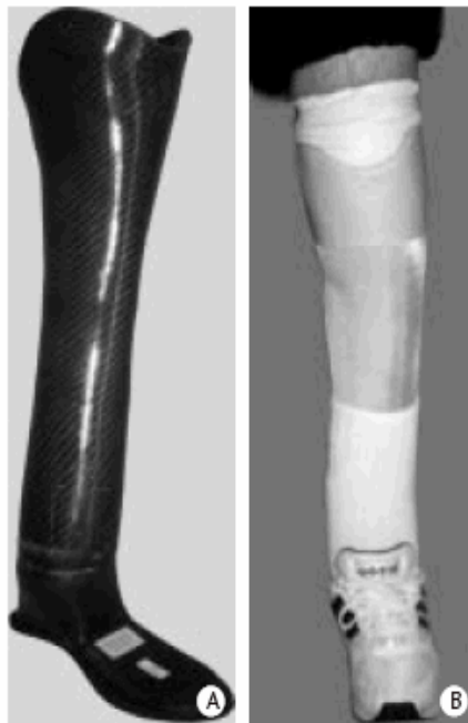
Figure. 44: prothèse de type Syme
