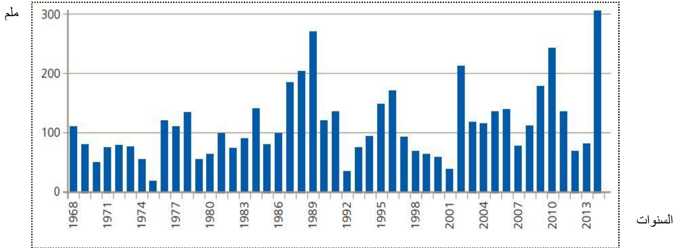
شكل رقم 9: توزيع التساقطات المطرية بمدينة كلميم ما بين سنتي 1968 و 2014 بالملم
