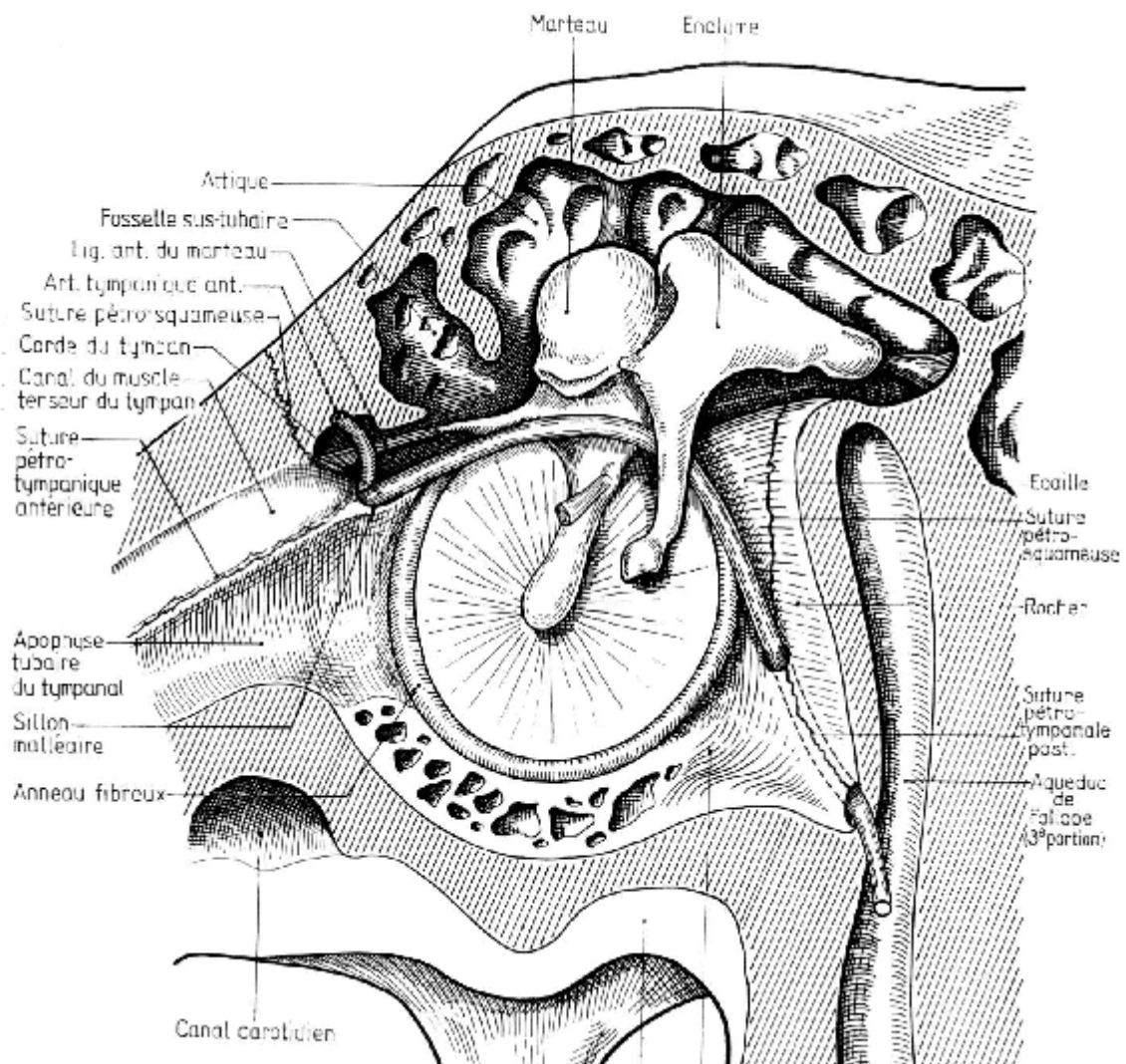
Figure 3: Paroi membraneuse ou latérale de la caisse. [55]
