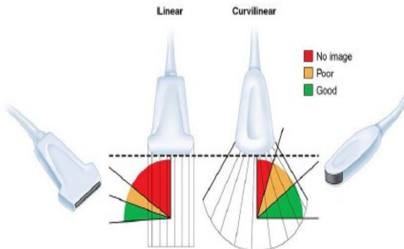
Figure 24 : Une sonde linéaire offre une résolution plus élevée avec une pénétration moindre. Une sonde curviligne permet une meilleure pénétration avec une résolution inférieure.
