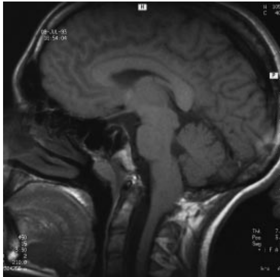
Fig.19 : Gliome de la jonction bulbomédullaire chez un garçon de 16 ans. Imagerie par résonance magnétique, séquence pondérée T1 : Déformation postérieure du bulbe et de la portion initiale de la moelle [2]
