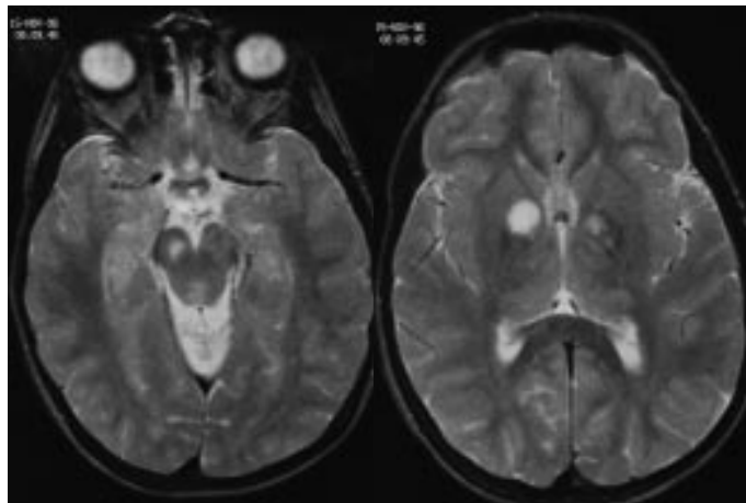
Fig.20 : Lésions hamartomateuses chez une fille de 10 ans. Imagerie par résonance magnétique, séquence pondérée T2 : A. Hypersignal du pédoncule cérébral droit. B. Hypersignal asymétrique des deux pallidums [2]
