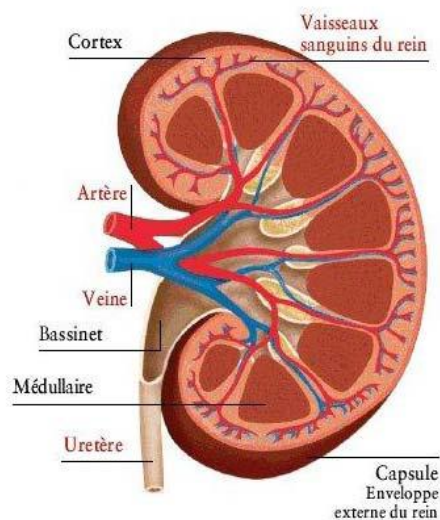
Figure 8 : Vascularisation rénale
