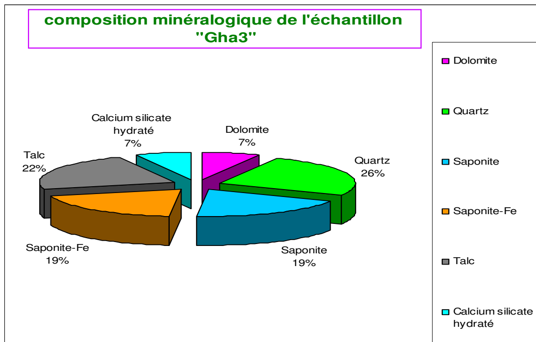
Figures 12 ; 12 bis : Diffractogramme de l'échantillon « Gha3 » et diagramme représentant sa composition minéralogique [7]
