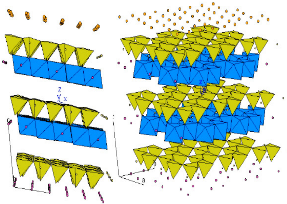
Assemblage d'une couche octaédrique et d'une couche tétraédrique pour une argile de type TO
