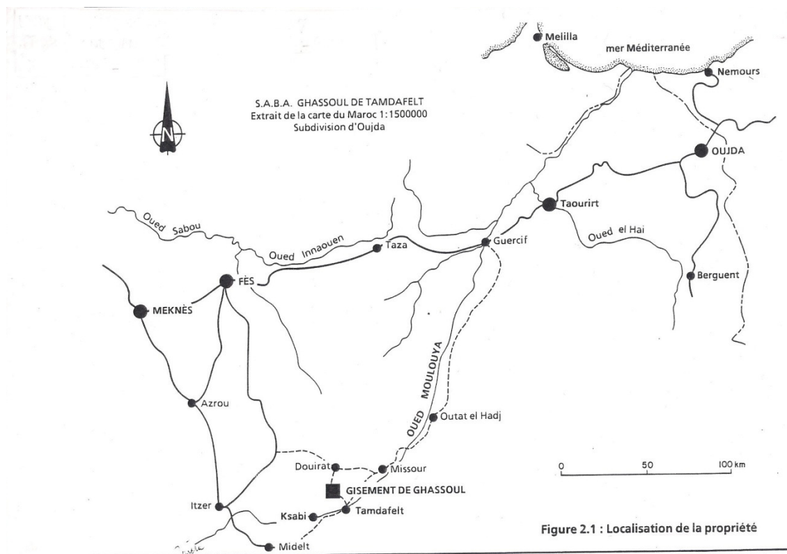
Figure 1: Localisation du gisement de Ghassoul [9 ; 20]
