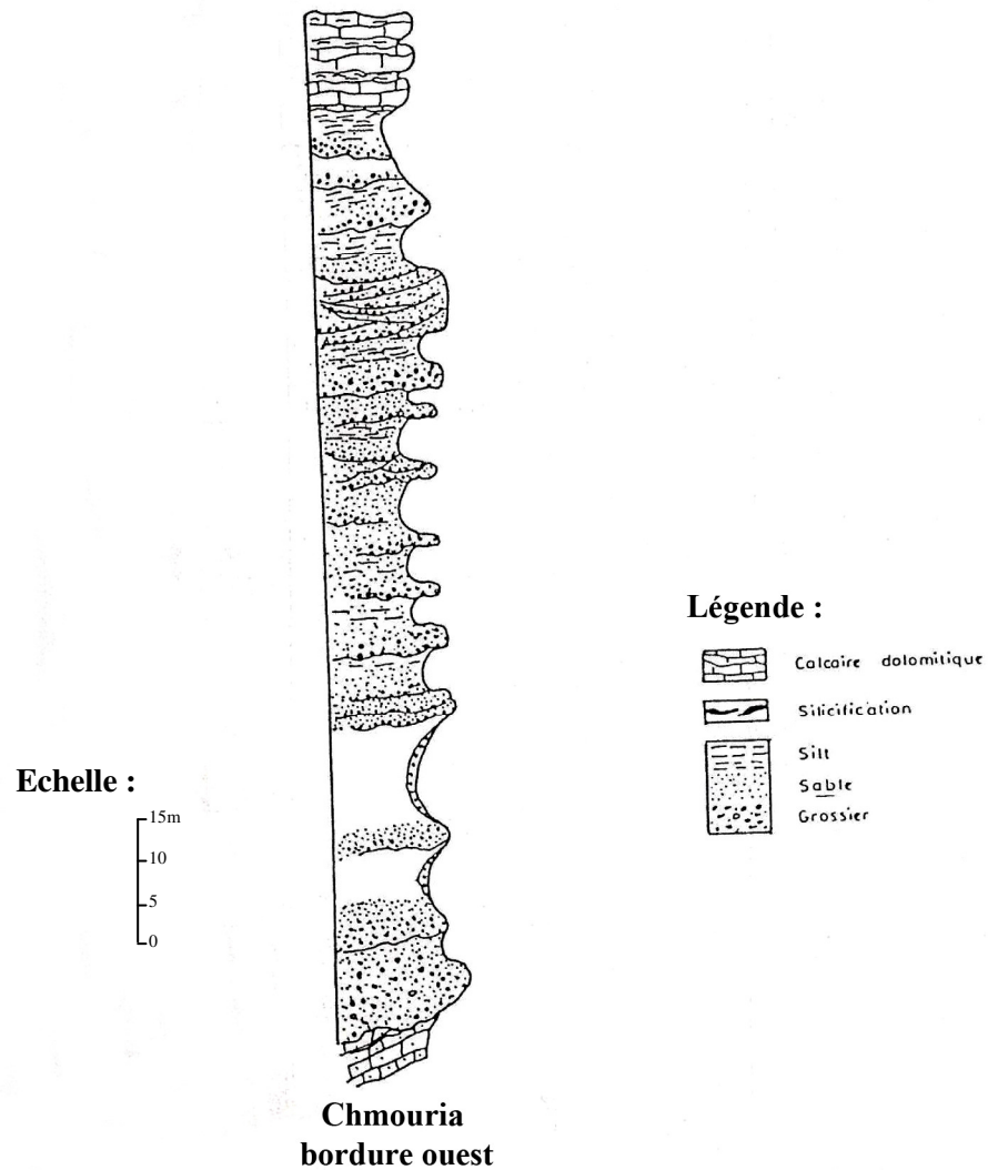
Figure 2: Coupe géologique du gisement de Ghassoul [9 ; 20]
