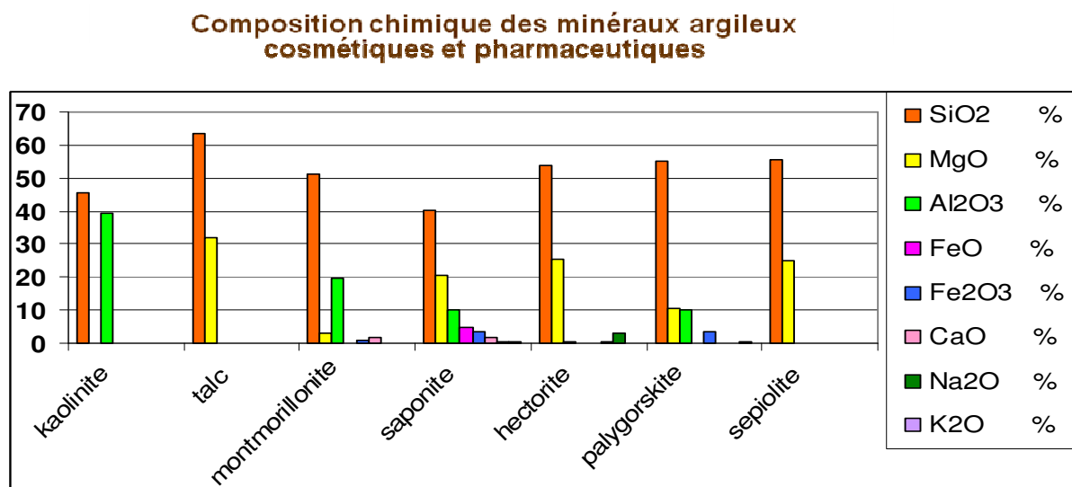
Figure 5 : Histogramme représentant la composition chimique des minéraux argileux cosmétiques et pharmaceutiques [7]
