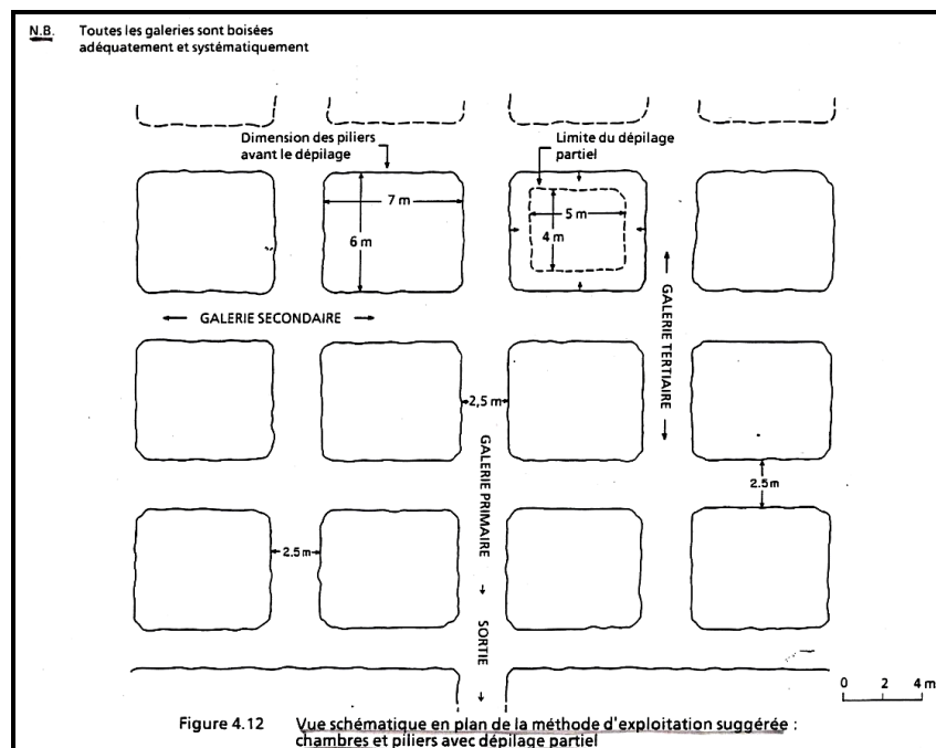
Figure 13 : Schéma de la méthode «Traçage-Dépilage» utilisée pour l'exploitation du ghassoul dans les galeries [10 ; 20]
