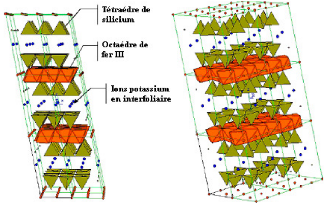
Représentation schématique d'un feuillet de phyllosilicate 2:1
