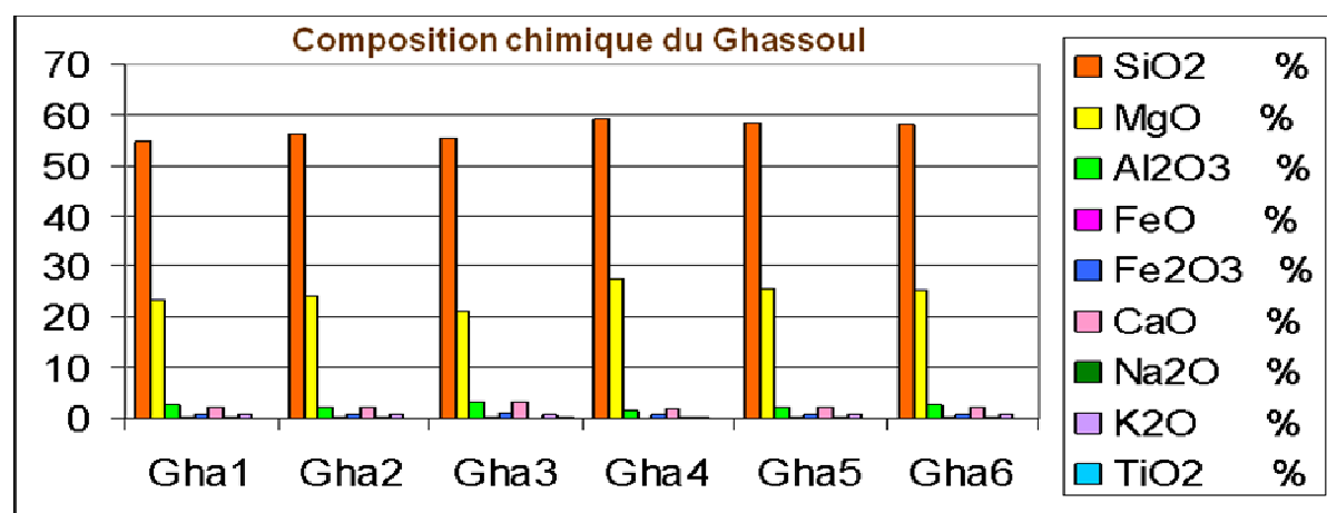
Figure 6 : Histogramme représentant la composition chimique du ghassoul pour les six échantillons [7]
