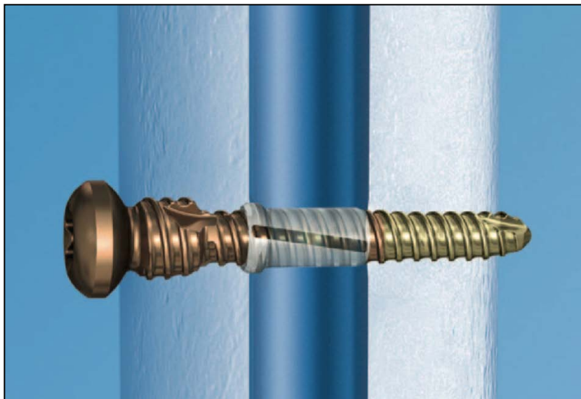
Figure n°45 : Schéma représentant une vis de verrouillage insérée dans le tibia et le clou distal
