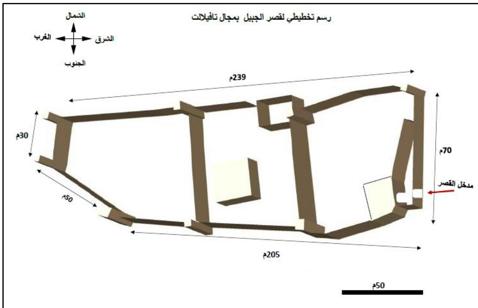
الشكل رقم 14: تخطيط قصر الجبيل بمجال تافيلالت
