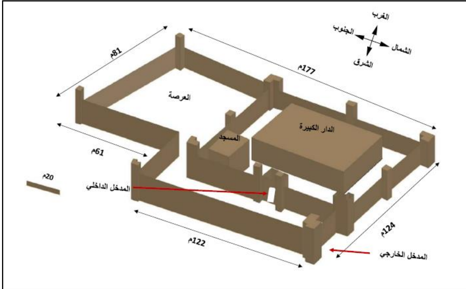
الشكل رقم 12 : تخطيط وأبعاد قصر أولاد عبد الحليم ومكوناته المعمارية
