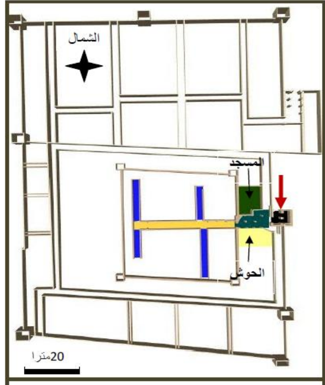
الشكل رقم 6 : تصميم قصر اللهاين بتيزيمي
