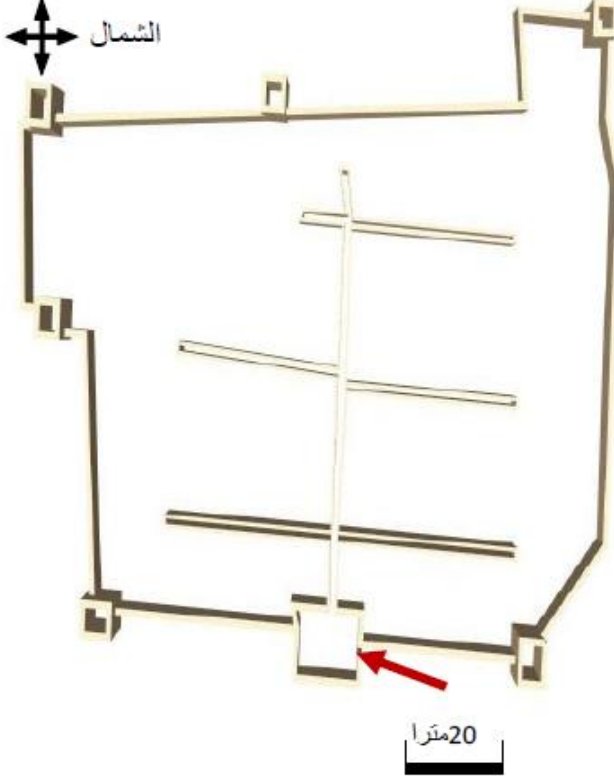
الشكل رقم 11 : تصميم قصر مولاي ابراهيم بتيزيمي
