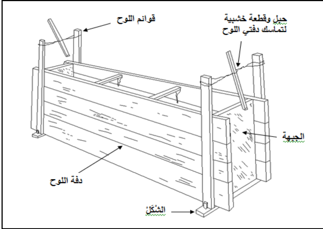
الشكل رقم 23 : رسم اللوح لبناء جدار الطابية
