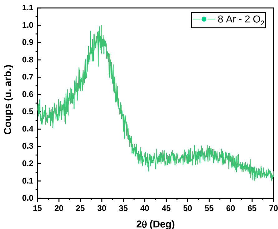
Figure 40 : Diffractogrammes du film de \text{SnO}_2 obtenus pour un débit de \text{O}_2 de 2 \text{ cm}^3/\text{min}
