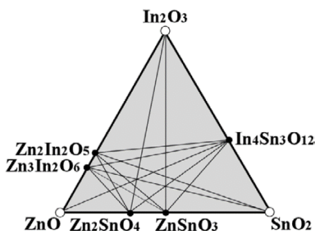
Figure 4 : Multi composés de ZnO, \text{In}_2\text{O}_3 et \text{SnO}_2 [3].
