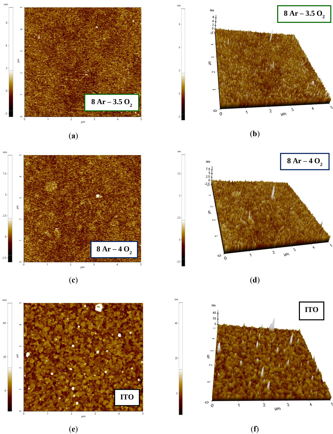
Figure 45 : Images AFM (a-d) des films de SnO 2 obtenus pour un débit de O 2 variable et (e-f) pour un substrat commercial d'ITO.
