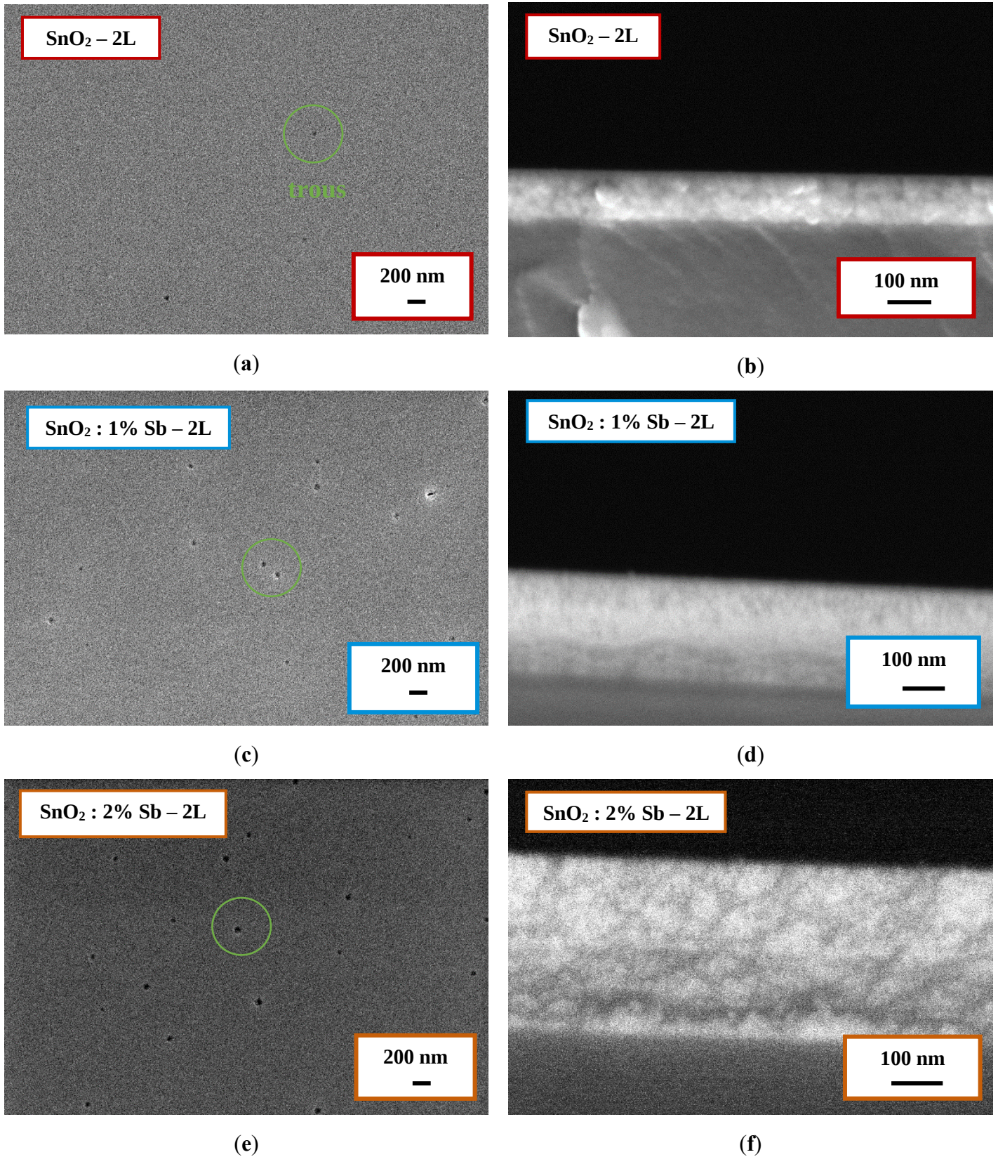
Figure 78 : Images MEB en surface et en coupe des films bicouches de \text{SnO}_2 dopé à l'antimoine ( \text{SnO}_2 : \text{Sb} ) élaborés à partir des solutions de concentration 0.75 mol/L.
