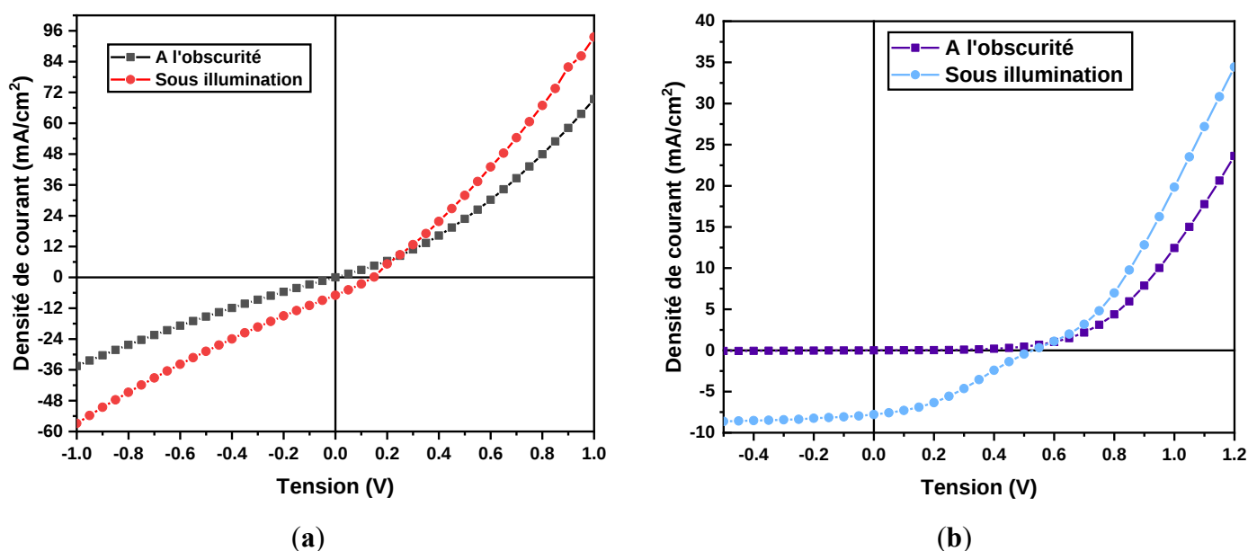
Figure 109 : Caractéristique densité de courant-tension J(V) des cellules OPV à base de P3HT : PC 60 BM ayant pour ETL des films monocouches a) de SnO 2 et b) SnO 2 : 5% Ge.
