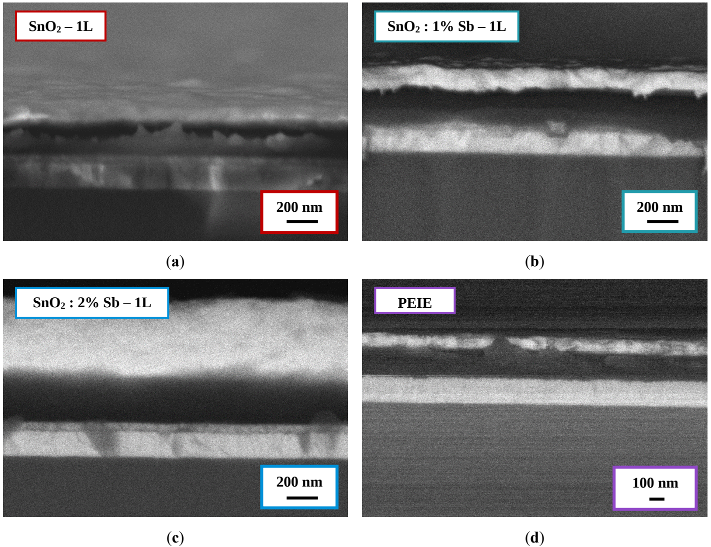
Figure 98 : Images MEB en coupe des cellules OPV à base de P3HT : \text{PC}_{60}\text{BM} ayant pour ETL (a – c) des films monocouches de \text{SnO}_2 dopé à l'antimoine ( \text{SnO}_2 : Sb) et d) une couche de PEIE.
