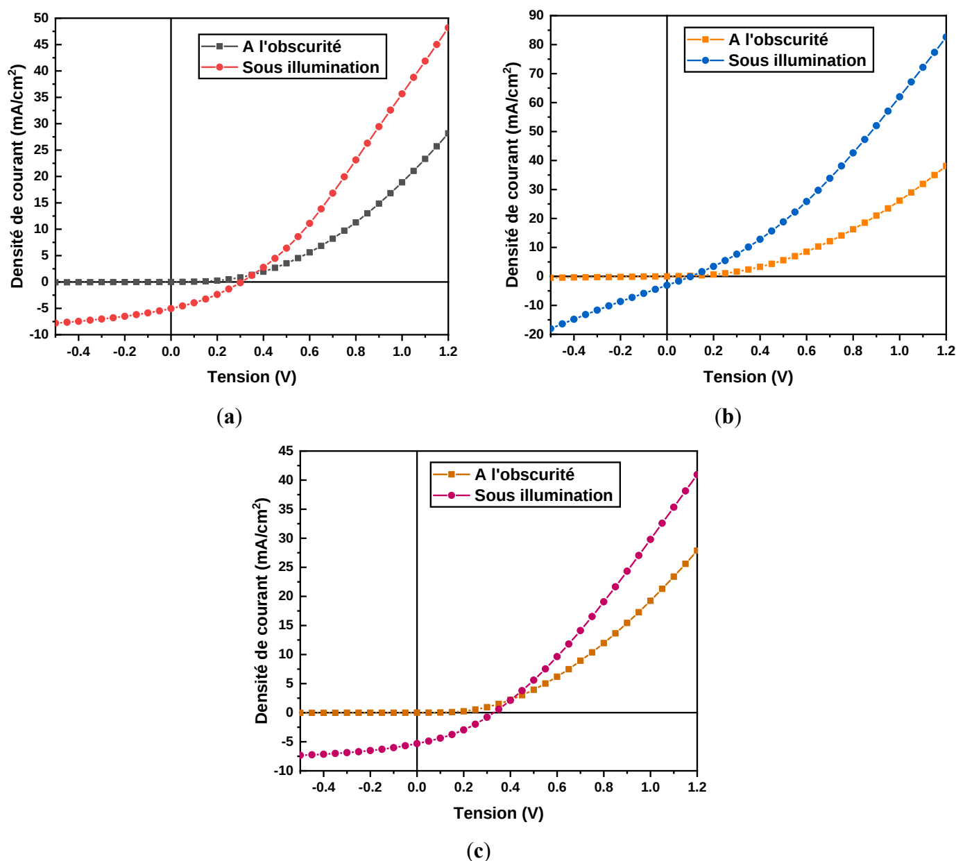
Figure 101 : Caractéristique densité de courant-tension J(V) des cellules OPV à base de P3HT : PC 60 BM ayant pour ETL des films monocouches a) de \text{SnO}_2 ; b) \text{SnO}_2 : 1% Sb et c) \text{SnO}_2 : 2% Sb.
