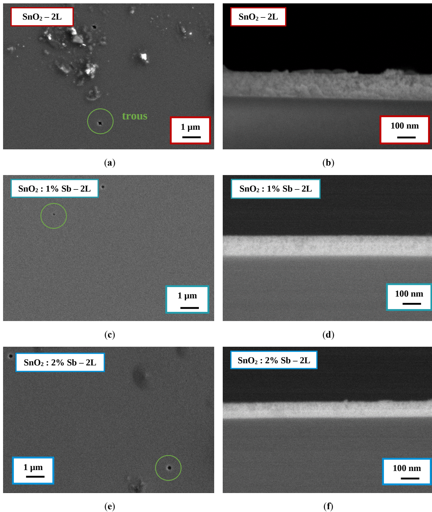
Figure 76 : Images MEB en surface et en coupe des films bicouches de SnO 2 dopé à l'antimoine (SnO 2 : Sb) élaborés à partir des solutions de concentration 0.50 mol/L.
