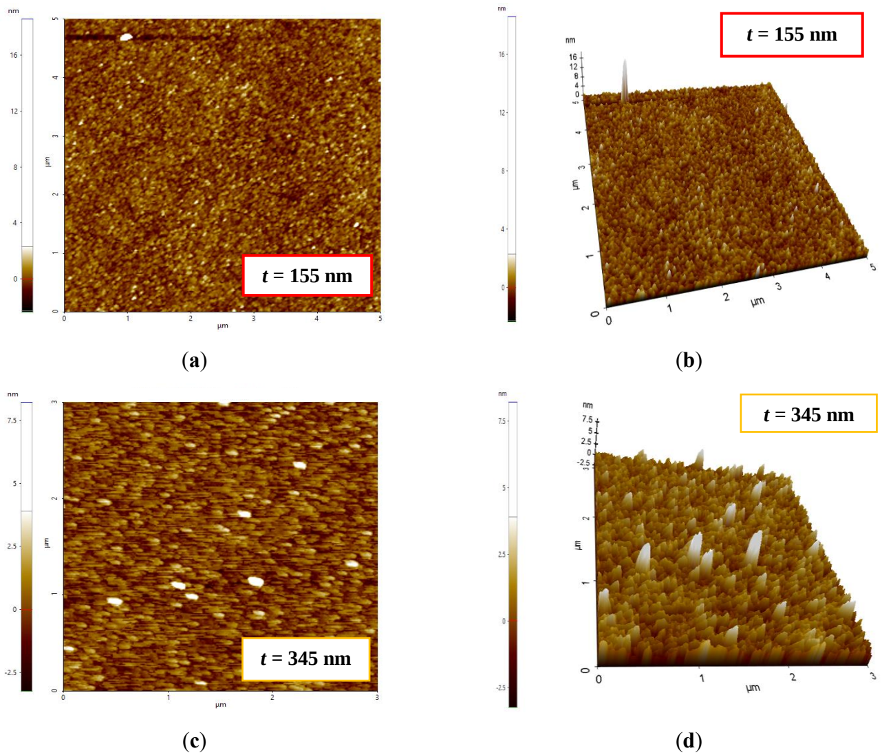
Figure 61 : Images AFM des films de SnO 2 obtenus pour différentes épaisseurs.
