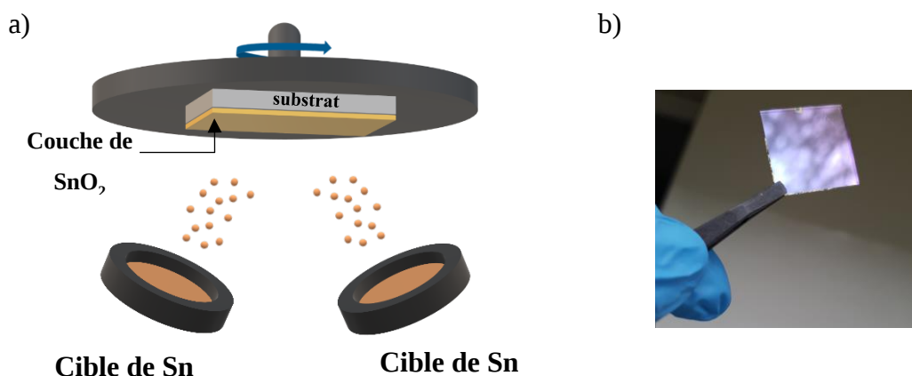
Figure 30 : a) Représentation du principe de pulvérisation cathodique et b) d'un film de \text{SnO}_2 déposé sur verre.
