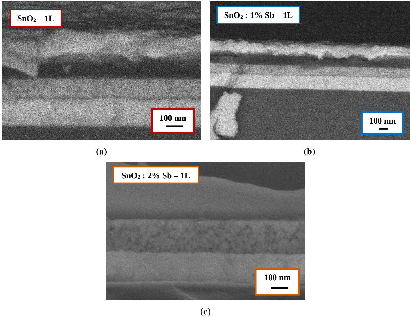
Figure 102 : Images MEB en coupe des cellules OPV à base de P3HT : \text{PC}_{60}\text{BM} ayant pour ETL (a – c) des films monocouches de \text{SnO}_2 dopé à l'antimoine ( \text{SnO}_2 : \text{Sb} ).
