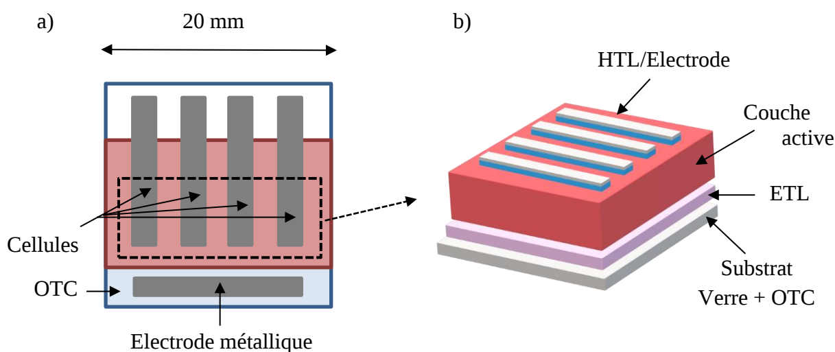
Figure 36 : a) Disposition des cellules organiques élaborées et b) description des différentes couches.
