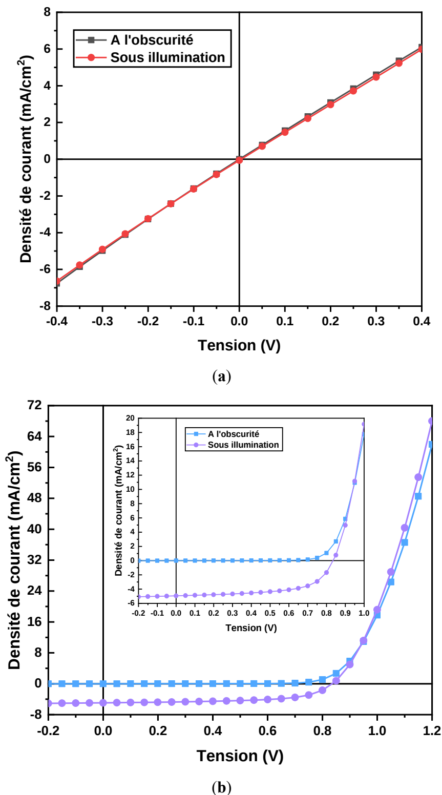
Figure 71 : Caractéristiques densité de courant-tension J(V) des cellules OPV à base de P3HT : ICBA ( C = 40 \text{ mg/mL} ) intégrant une électrode a) de \text{SnO}_2 et b) d'ITO.
