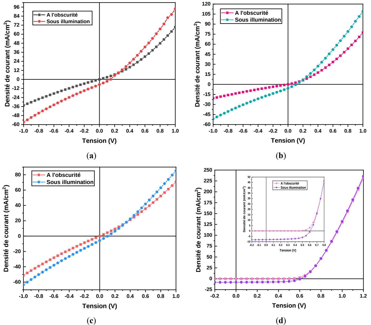
Figure 97 : Caractéristique densité de courant-tension J(V) des cellules OPV à base de P3HT : PC 60 BM ayant pour ETL des films monocouches a) de SnO 2 ; b) SnO 2 : 1% Sb, c) SnO 2 : 2% Sb et d) une couche de PEIE.
