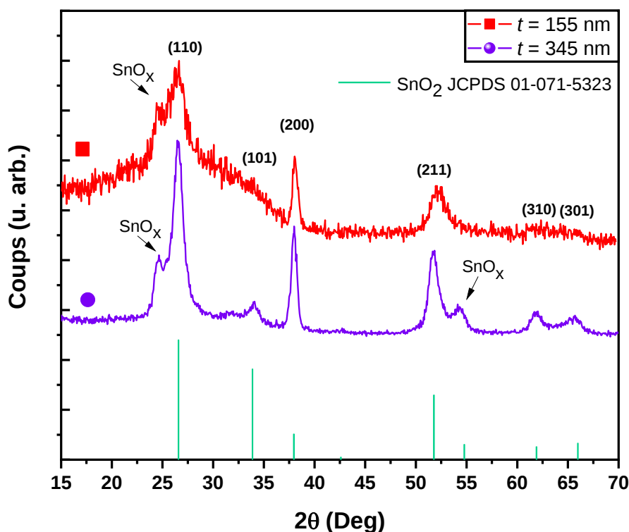
Figure 59 : Diffractogrammes des films de \text{SnO}_2 obtenus pour différentes épaisseurs. Les courbes ont été traduites pour une meilleure visibilité.
