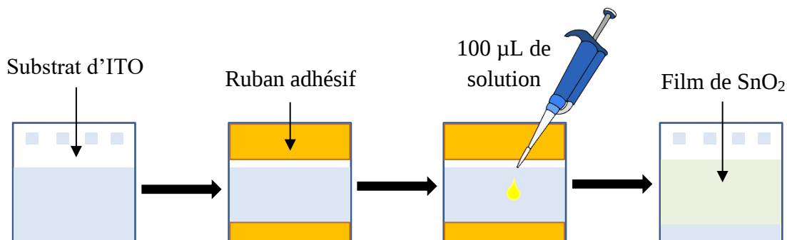
Figure 35 : Représentation du procédé de réalisation par voie sol-gel des films de \text{SnO}_2 non dopé et dopé sur des substrats d'ITO gravés pour l'élaboration de cellules organiques.
