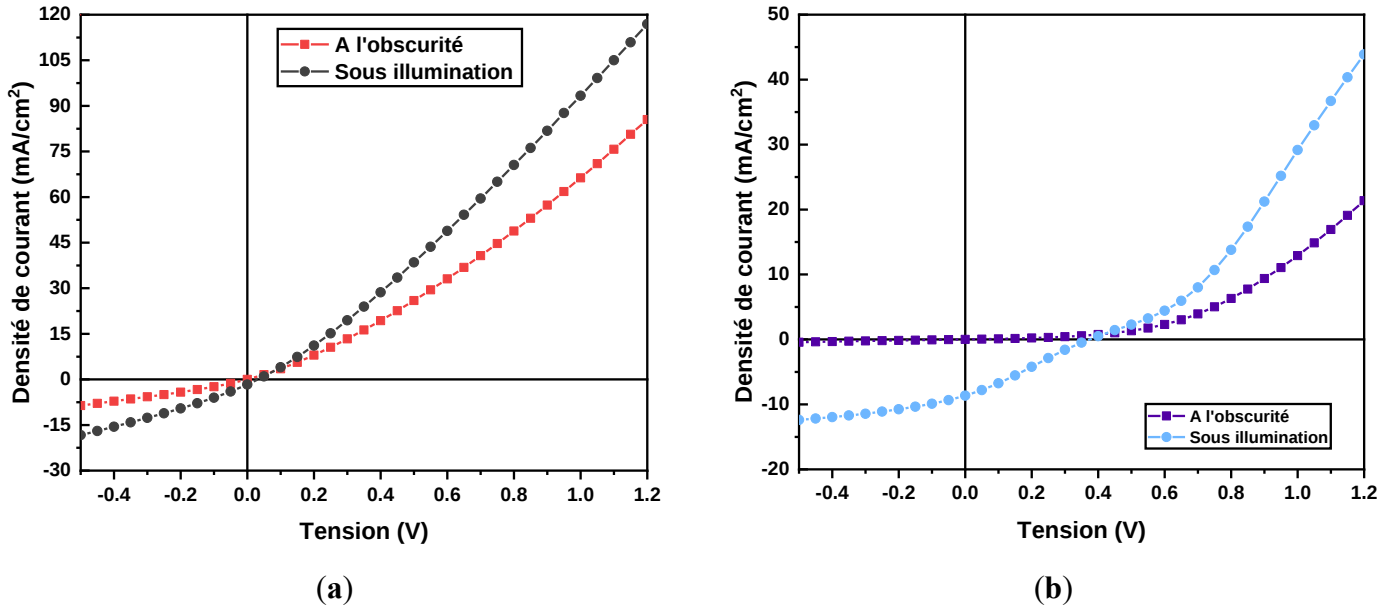
Figure 111 : Caractéristique densité de courant-tension J(V) des cellules OPV à base de P3HT : PC 60 BM ayant pour ETL des films bicouches dopé au germanium ( \text{SnO}_2 : Ge).
