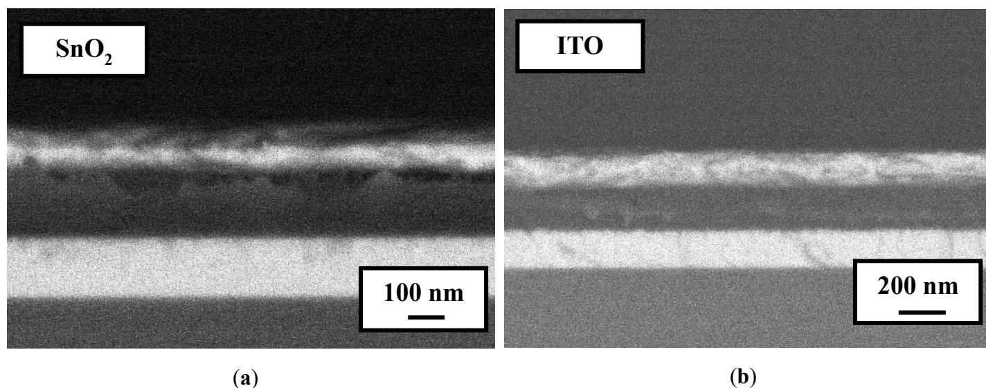
Figure 68 : Images MEB en coupe des cellules OPV à base de P3HT : PC 60 BM ( C = 40 mg/mL) intégrant une électrode a) de \text{SnO}_2 et b) d'ITO.
