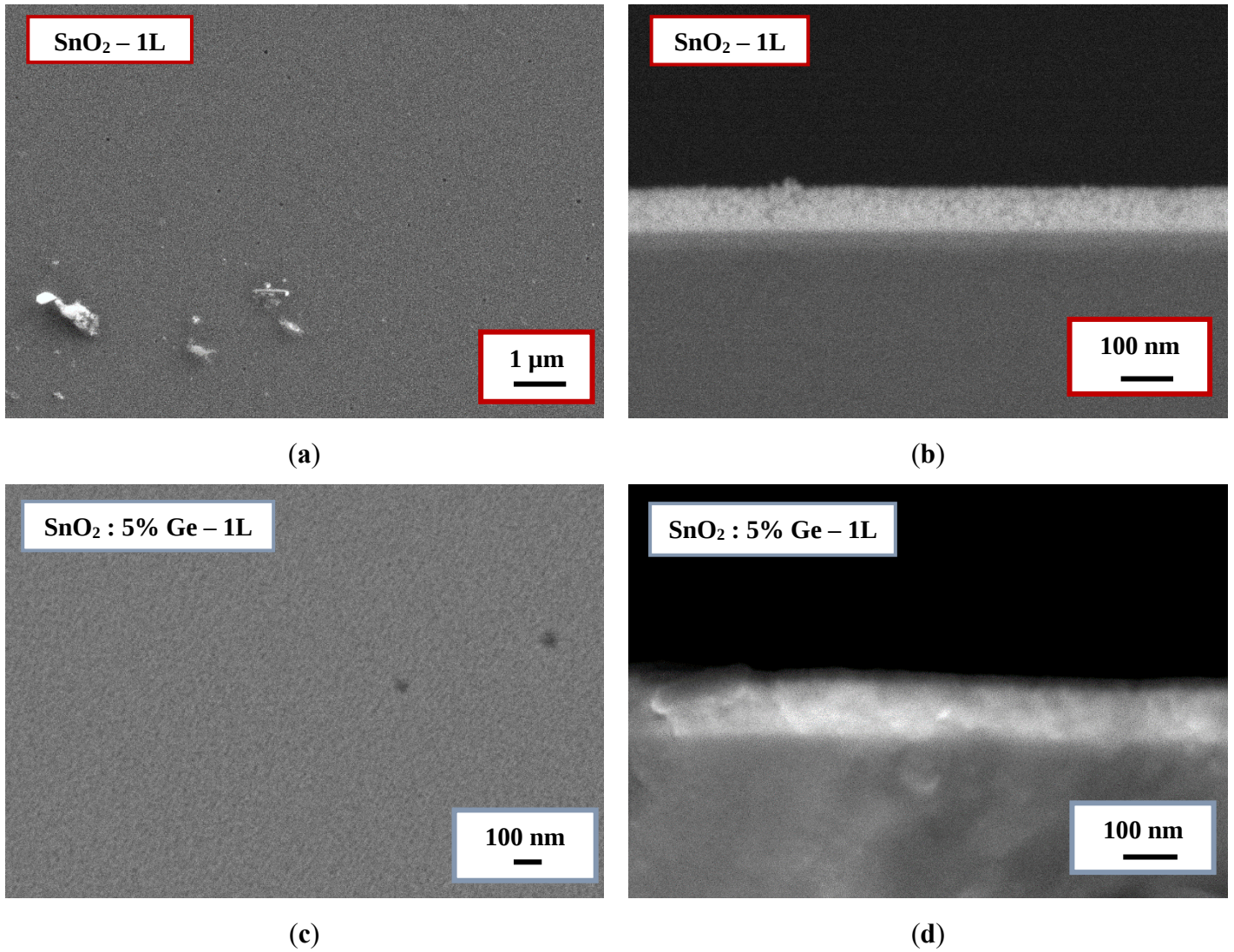
Figure 92 : Images MEB en surface et en coupe des films monocouches de \text{SnO}_2 dopé au germanium ( \text{SnO}_2 : \text{Ge} ).
