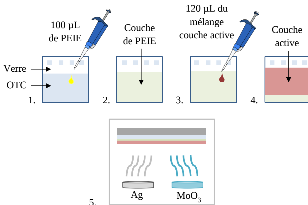
Figure 38 : Procédé d'élaboration d'une cellule organique avec ITO ou SnO 2 en tant que OTC.
