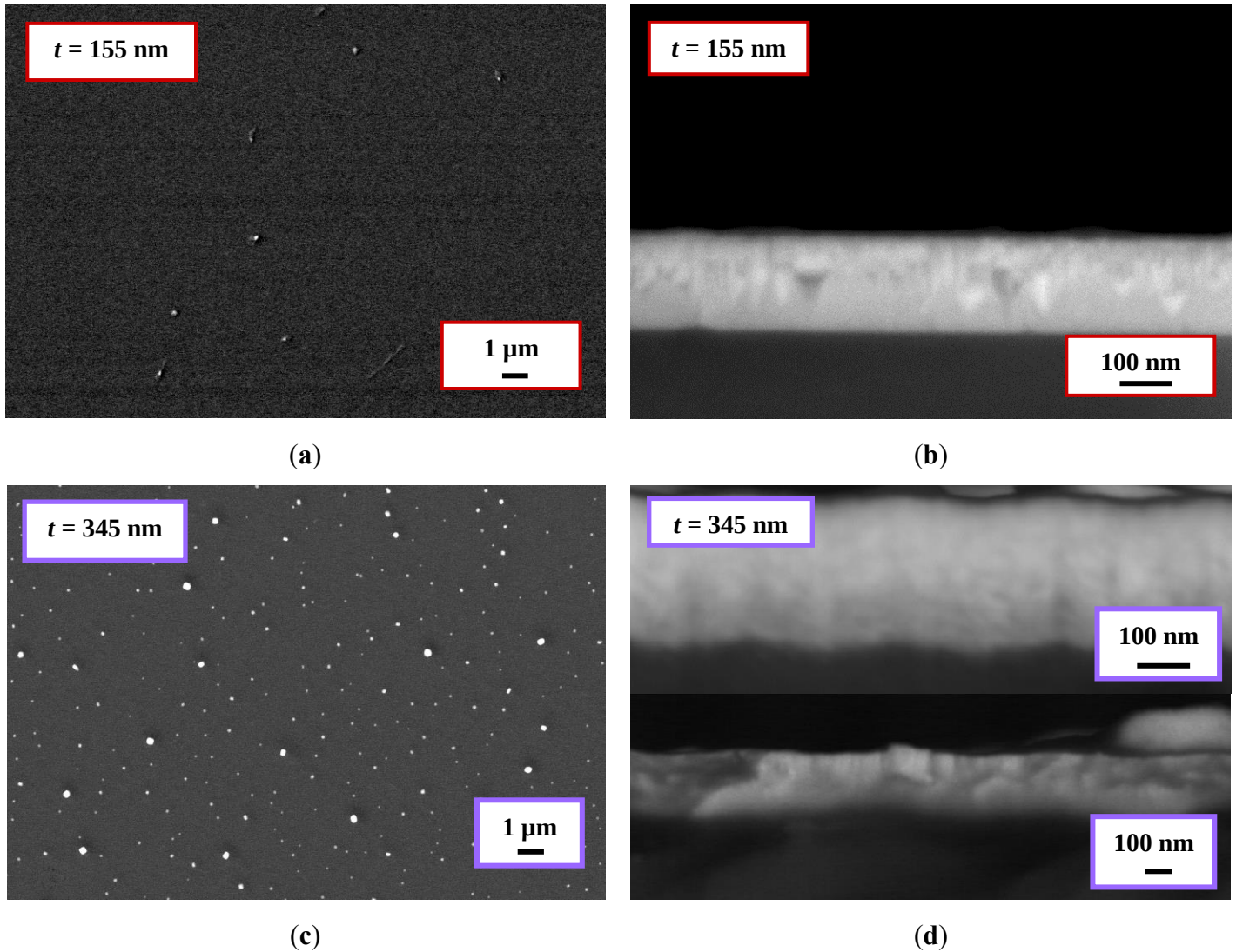
Figure 60 : Images MEB en surface et en coupe des films de SnO 2 obtenus pour différentes épaisseurs.
