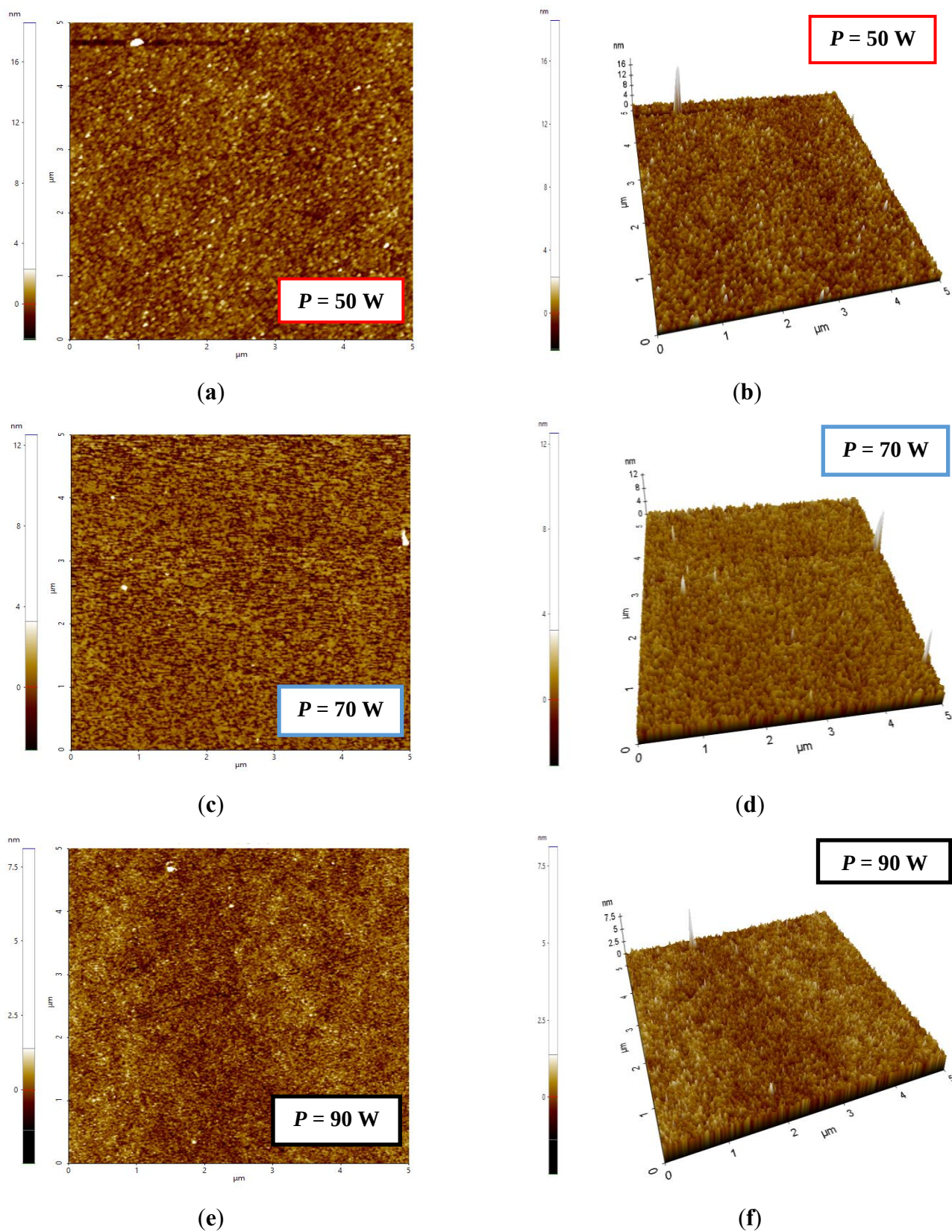
Figure 56 : Images AFM des films de \text{SnO}_2 obtenus pour différentes puissances.
