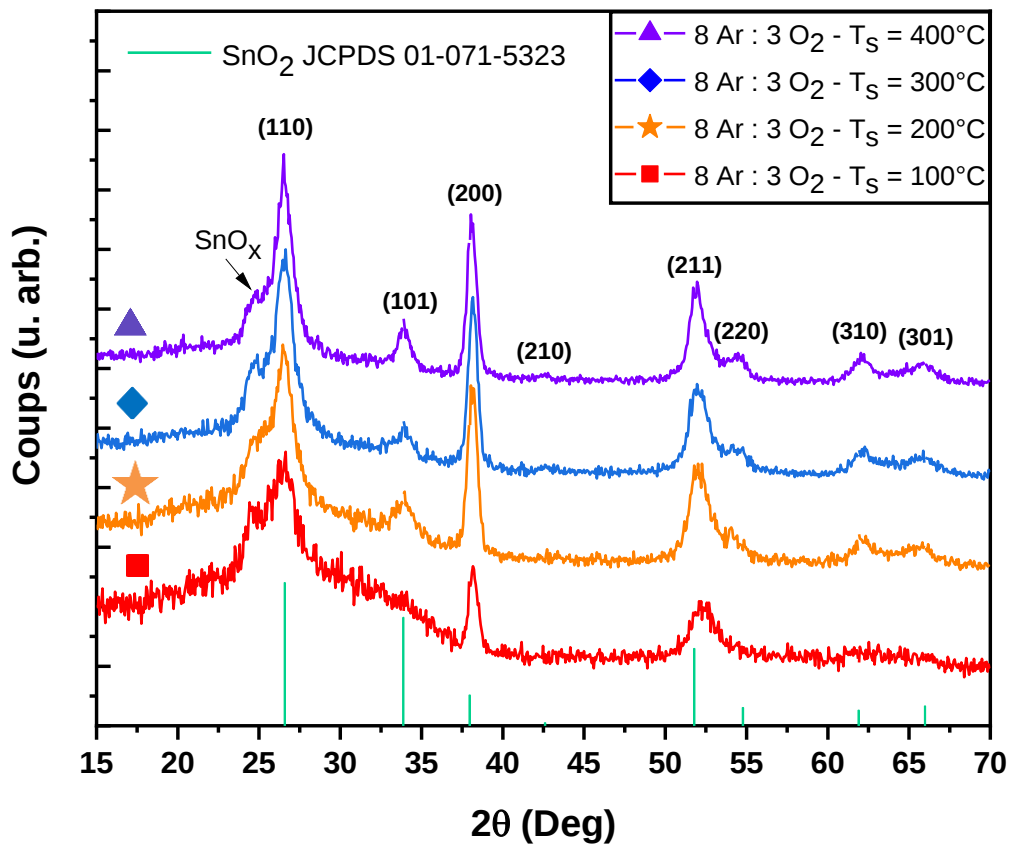
Figure 49 : Diffractogrammes des films de \text{SnO}_2 obtenus pour une température de substrat T_S variable. Les courbes ont été translattées pour une meilleure visibilité.
