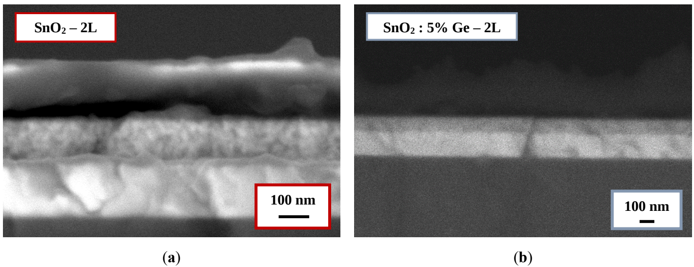
Figure 112 : Images MEB en coupe des cellules OPV à base de P3HT : PC 60 BM ayant pour ETL (a – c) des films bicouches de \text{SnO}_2 dopé au germanium ( \text{SnO}_2 : Ge).
