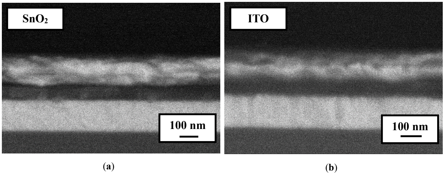
Figure 66 : Images MEB en coupe des cellules OPV à base de P3HT : \text{PC}_{60}\text{BM} ( C = 20 mg/mL) intégrant une électrode a) de \text{SnO}_2 et b) d'ITO.
