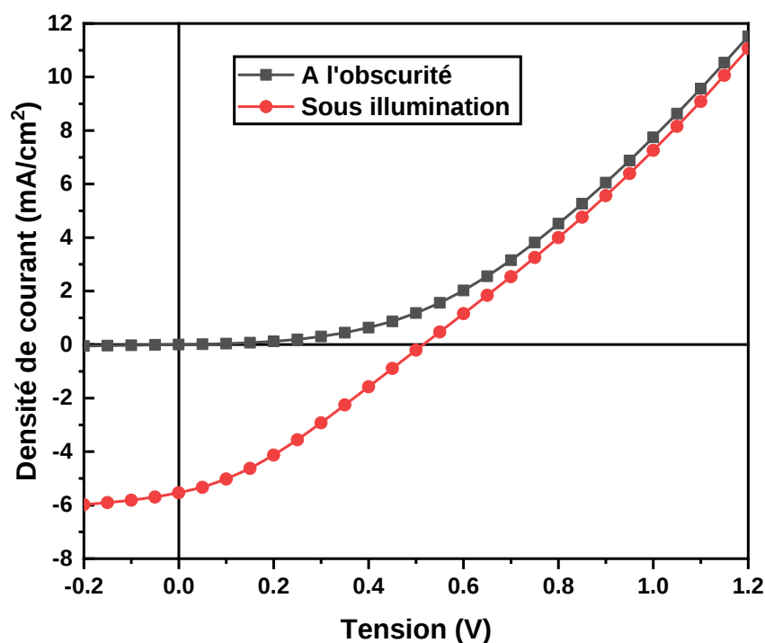
Figure 64 : Caractéristiques densité de courant-tension J(V) des cellules OPV à base de P3HT : \text{PC}_{60}\text{BM} ( C = 20 \text{ mg/mL} ) intégrant une électrode de \text{SnO}_2 .
