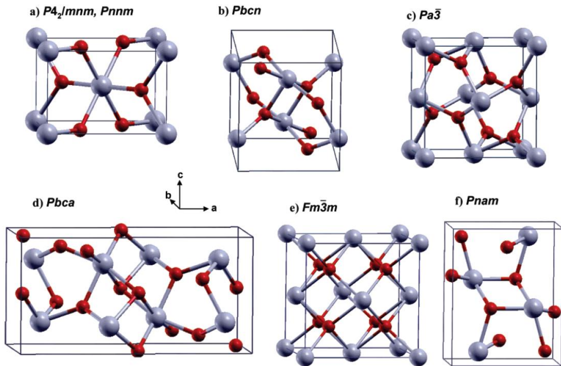
Figure 12 : Structures cristallographiques des différentes phases de \text{SnO}_2 (en gris les atomes Sn et rouge les atomes O). (a) Rutile ( P4_2/mnm ) et type \text{CaCl}_2 ( Pnnm ), (b) type \alpha\text{-PbO}_2 ( Pbcn ), (c) type pyrite ( Pa\bar{3} ), (d) type \text{ZrO}_2 ( Pbca ), (e) type fluorite ( Fm\bar{3}m ), and (f) type cotunnite ( Pnam ) [105].
