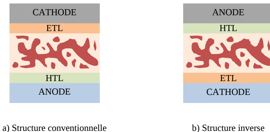
Figure 26 : Architectures des cellules solaires organiques.
