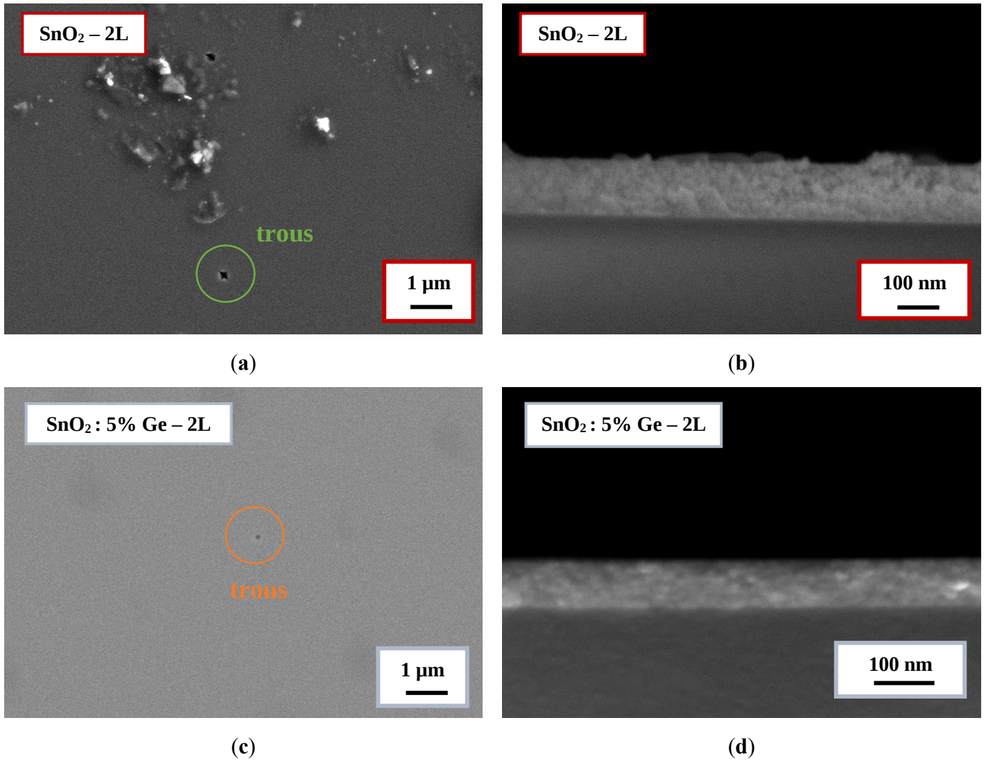
Figure 93 : Images MEB en surface et en coupe des films bicouches de \text{SnO}_2 dopé au germanium ( \text{SnO}_2 : \text{Ge} ).
