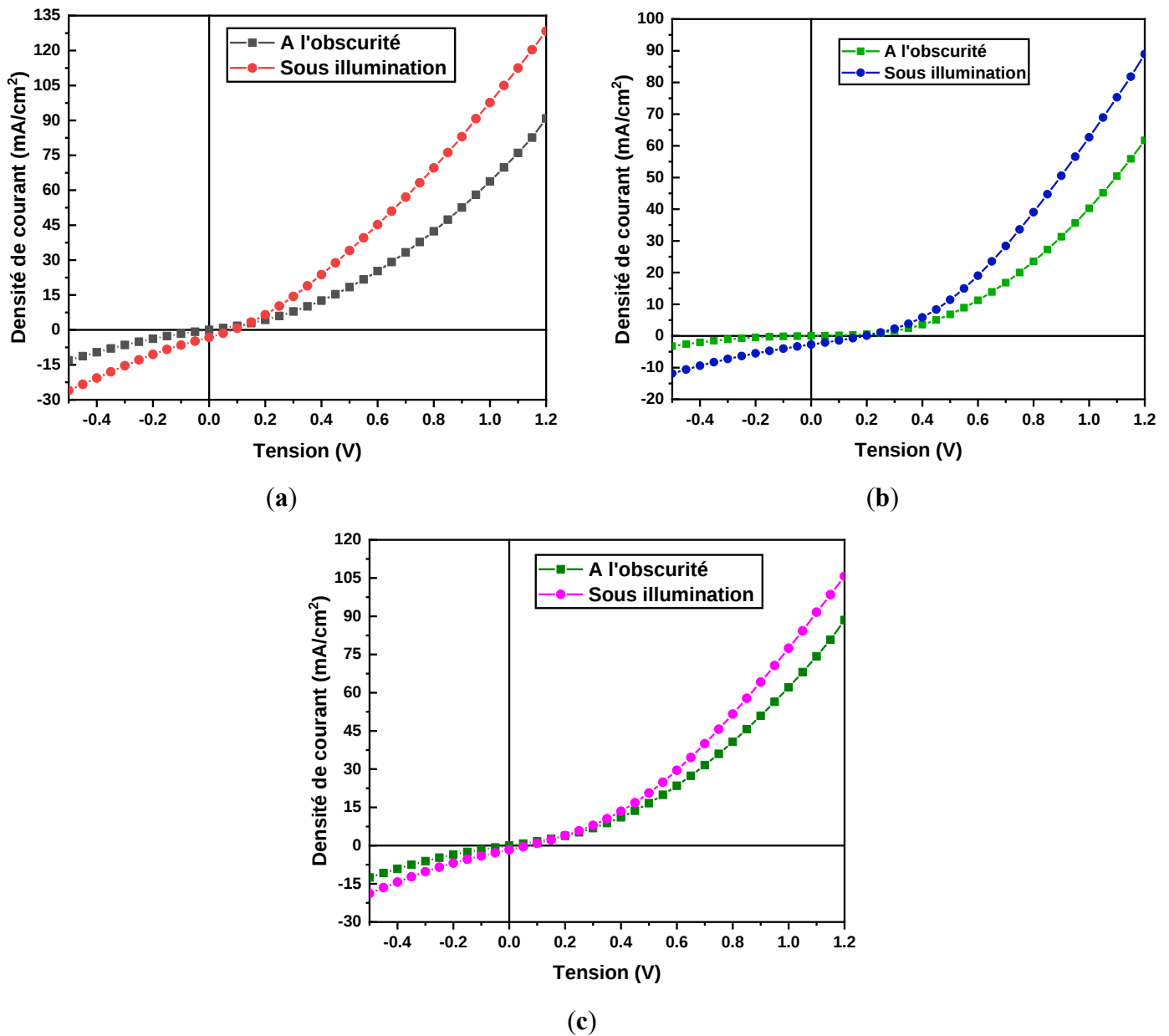
Figure 107 : Caractéristique densité de courant-tension J(V) des cellules OPV à base de P3HT : PC 60 BM ayant pour ETL des films bicouches a) de \text{SnO}_2 ; b) \text{SnO}_2 : 5% In et c) \text{SnO}_2 : 10%.
