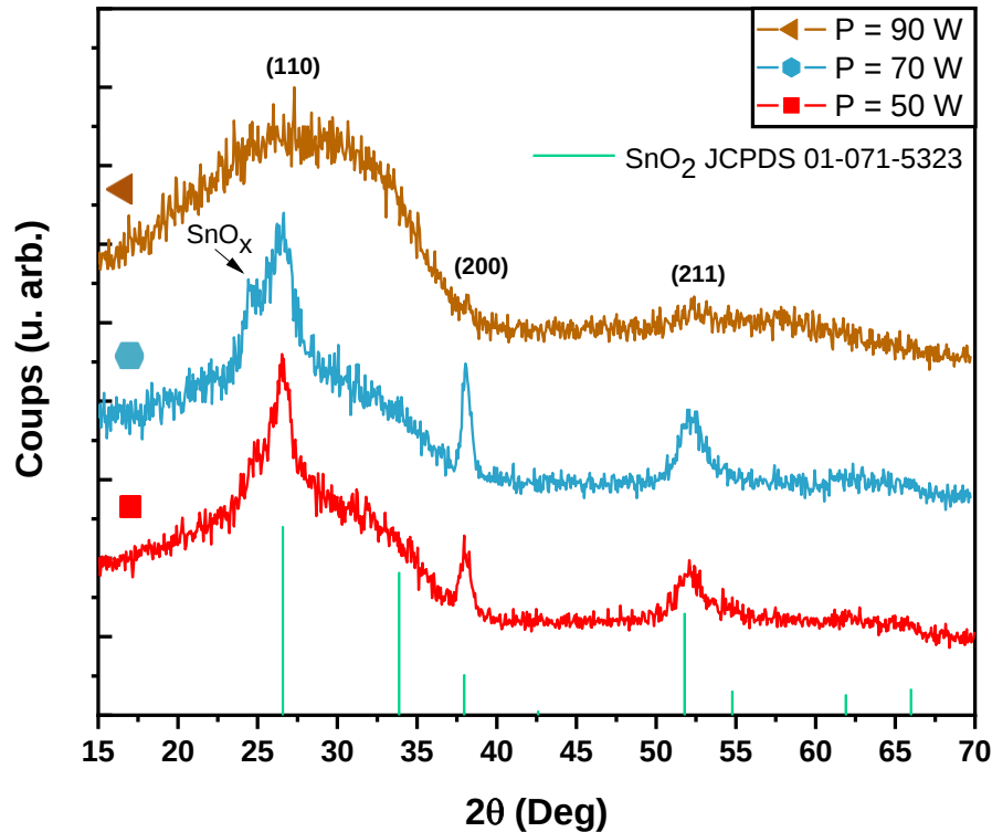
Figure 54 : Diffractogrammes des films de \text{SnO}_2 obtenus pour une puissance variable. Les courbes ont été traduites pour une meilleure visibilité.
