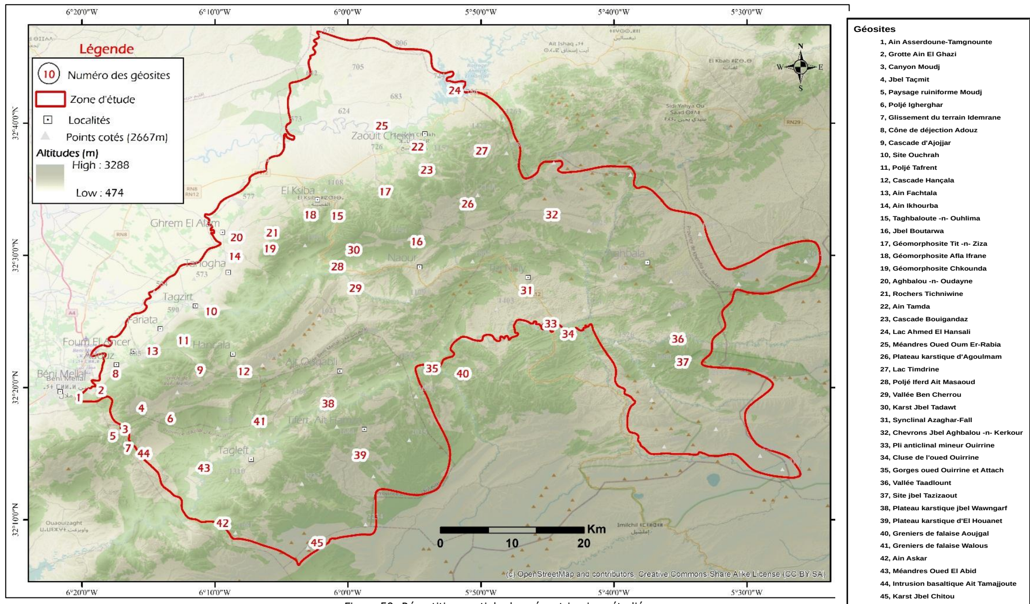
Figure 58: Répartition spatiale des géopatrimoines étudiés
