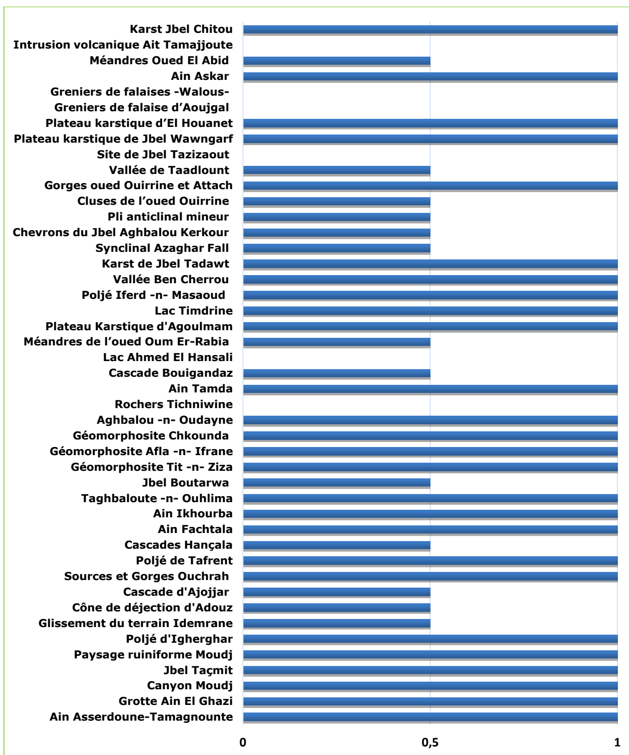
Figure 71: Scores de la représentativité des géopatrinoines étudiés
