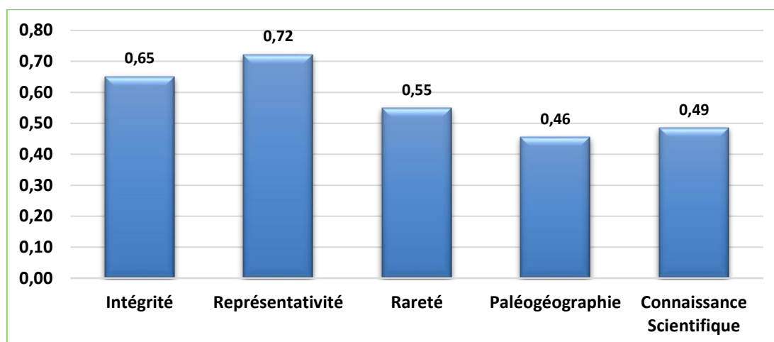
Figure 67: Valeurs des sous-critères de la valeur scientifique
