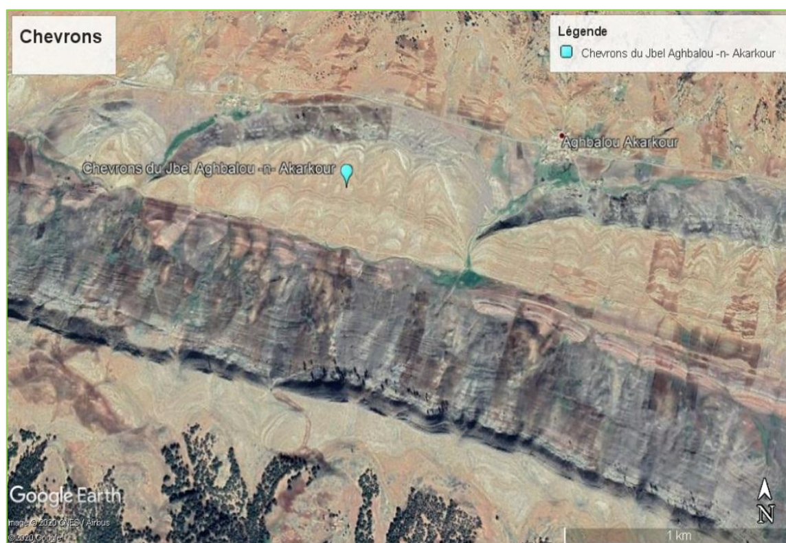
Figure 13: les chevrons du Jbel Aghbalou -n- Kerkour à Tizi Nisly (Google Earth, 2020)
