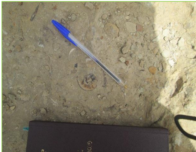
Photo 60: Fossiles sur le plateau d'Agoulmam, Oum El Bakht, (Ait Omar, 2020)
