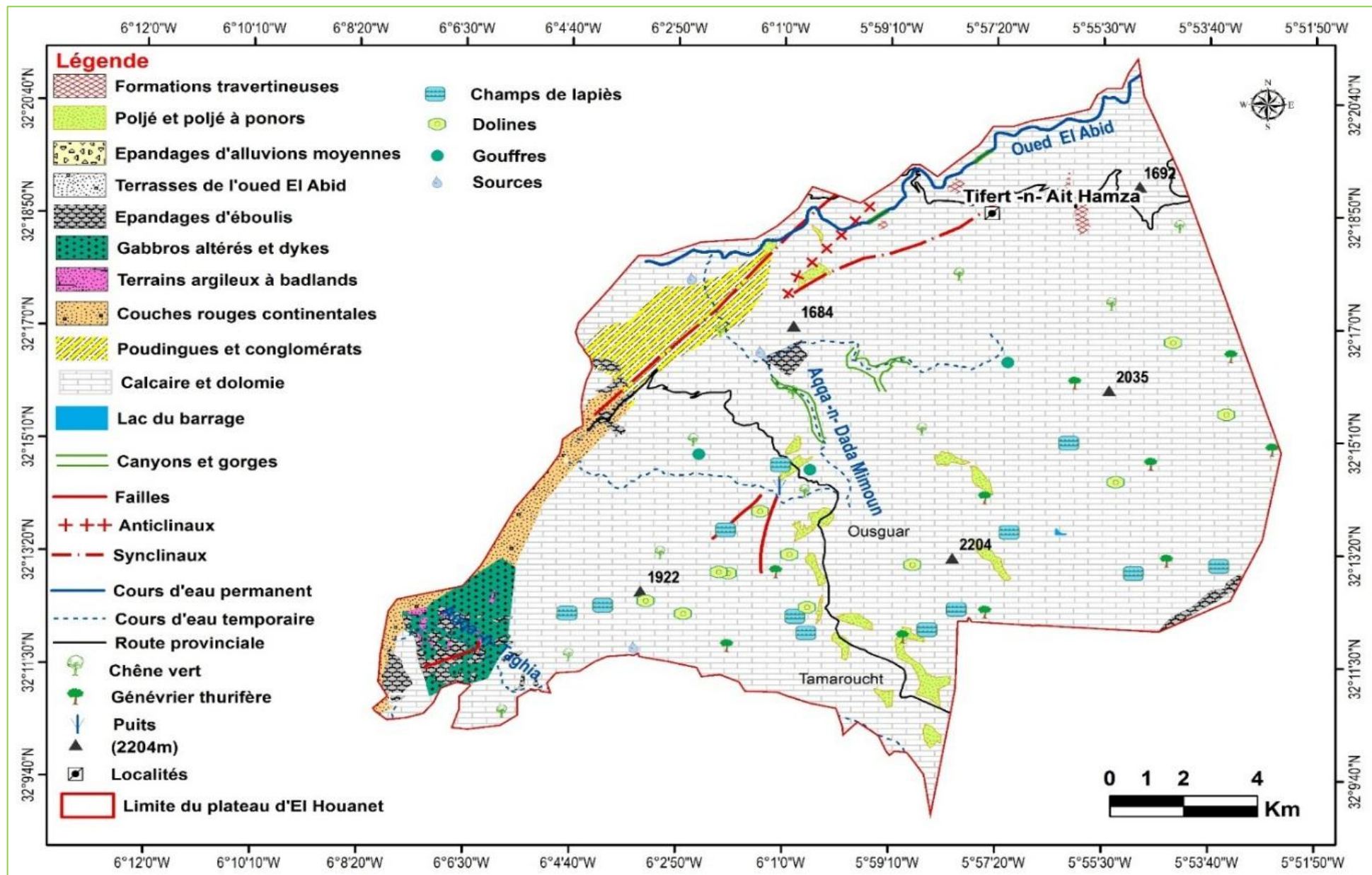
Figure 23: Carte géomorphologique simplifiée (Carte géologique d'Imilchil, 1/100000, carte topographique Imilchil, 1/100000 et images de Google Earth, 2020)
