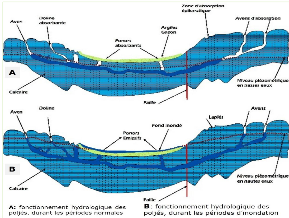
Figure 17: A) fonctionnement hydrologique des poljés durant les périodes normales B) période d'inondation. (Salomon, 2006)
