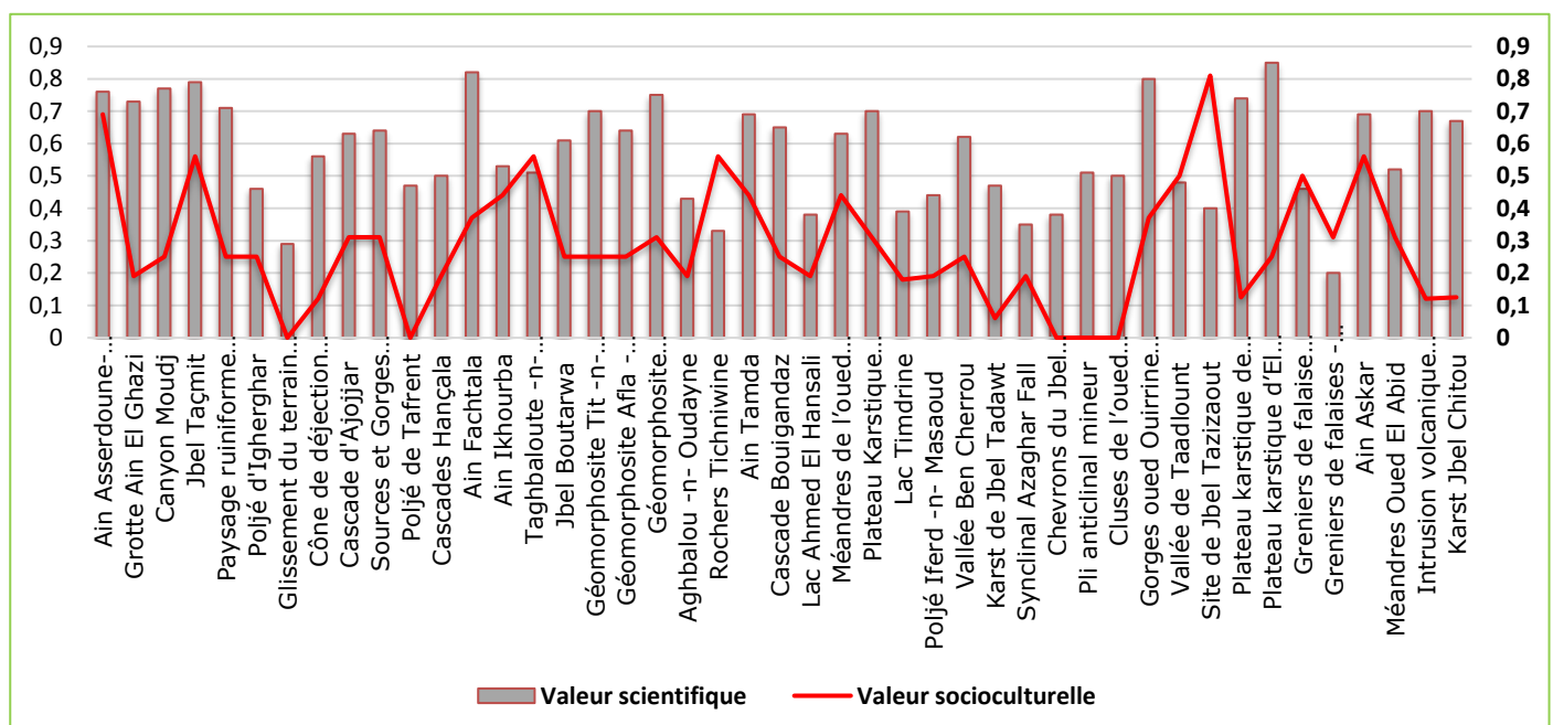
Figure 83: scores de la relation entre la valeur géoscientifique et la valeur scoio-culturelle des géopatrimoines étudiés
