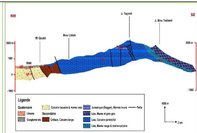
A- Coupe géologique du Jbel Tagmit à Fom El Ancer
