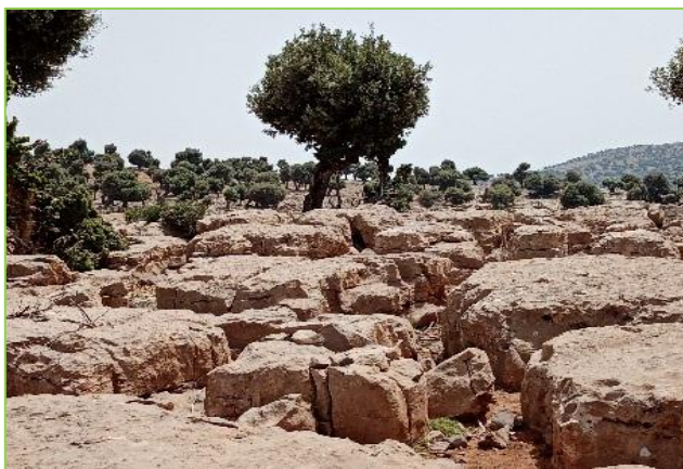
Photo 17: lapiés de dissolution d'Ousguar (Ait Omar, 2020) ; Photo 18: Lapiés de diaclases d'Ousguar (Ait Omar, 2020)
