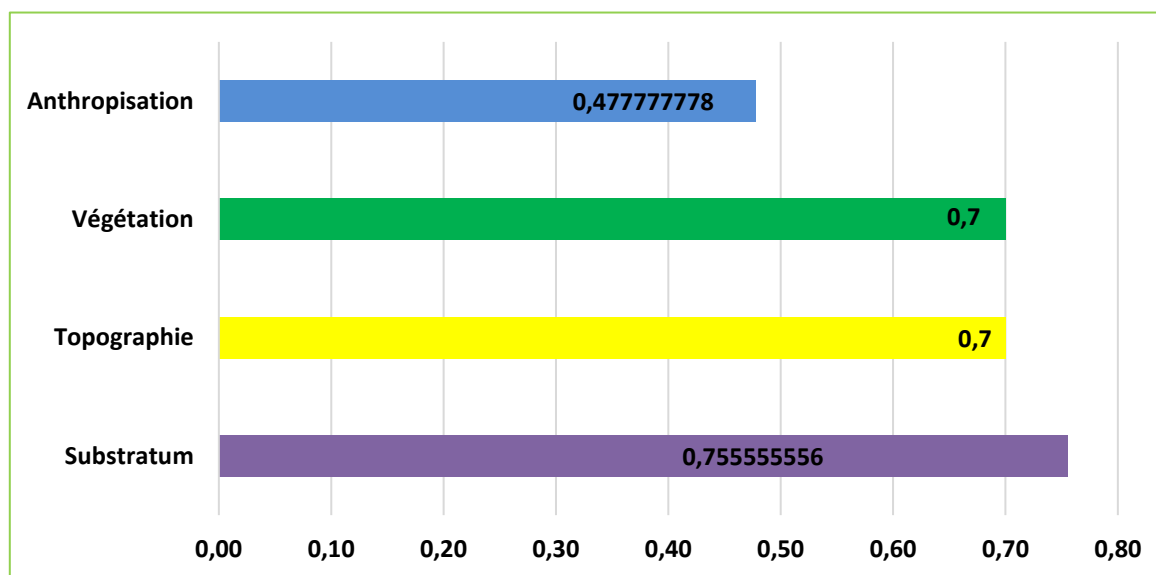
Figure 70: la moyenne de variables composant l'intégrité des géopatrinoines étudiés
