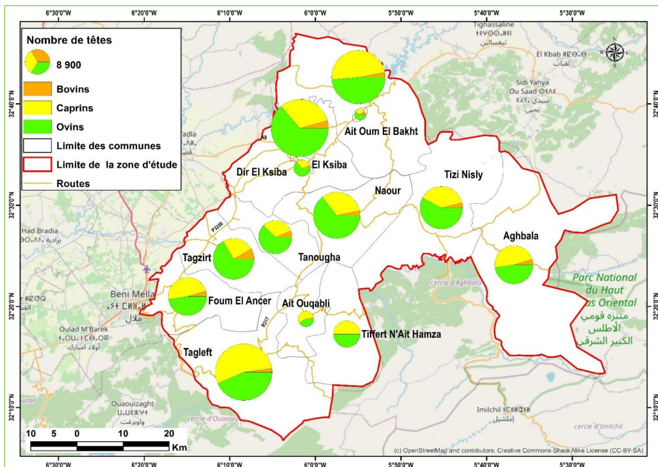
Figure 38: Répartition du nombre de têtes de bovins, caprins et ovins dans la zone d'étude (Taïbi et al., 2015)
