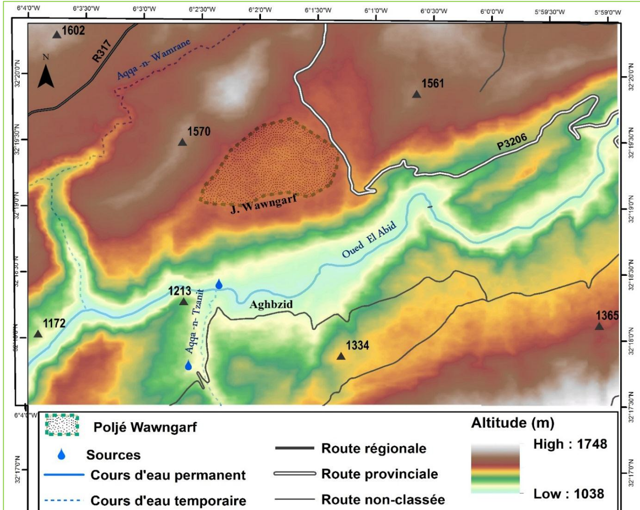
Figure 25: Modèle numérique du terrain du complexe karstique Wawngarf
