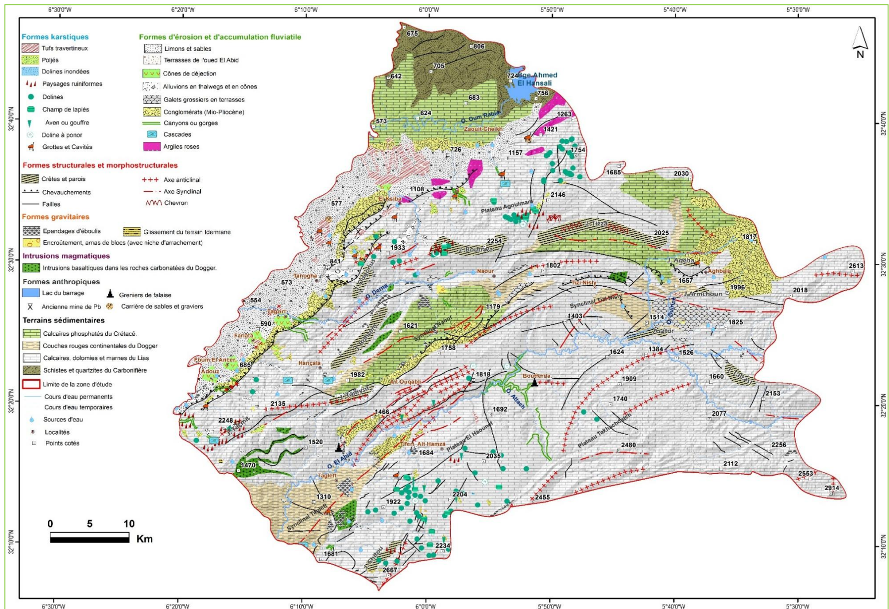
Figure 34: Carte géomorphologique simplifiée de la zone d'étude (Carte géologiques : Béni Mellal, Imilchil 1/100000 et de Rabat, 1/500000 et images Google Earth 2020 et visites du terrain (2018-2021)
