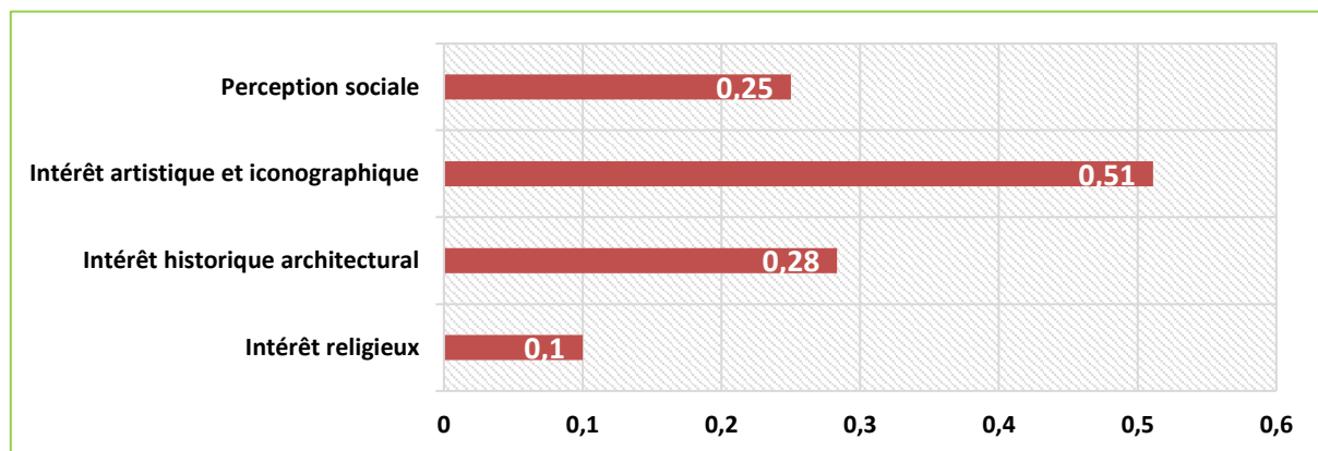
Figure 82: moyenne des critères de la valeur scoio-culturelle
