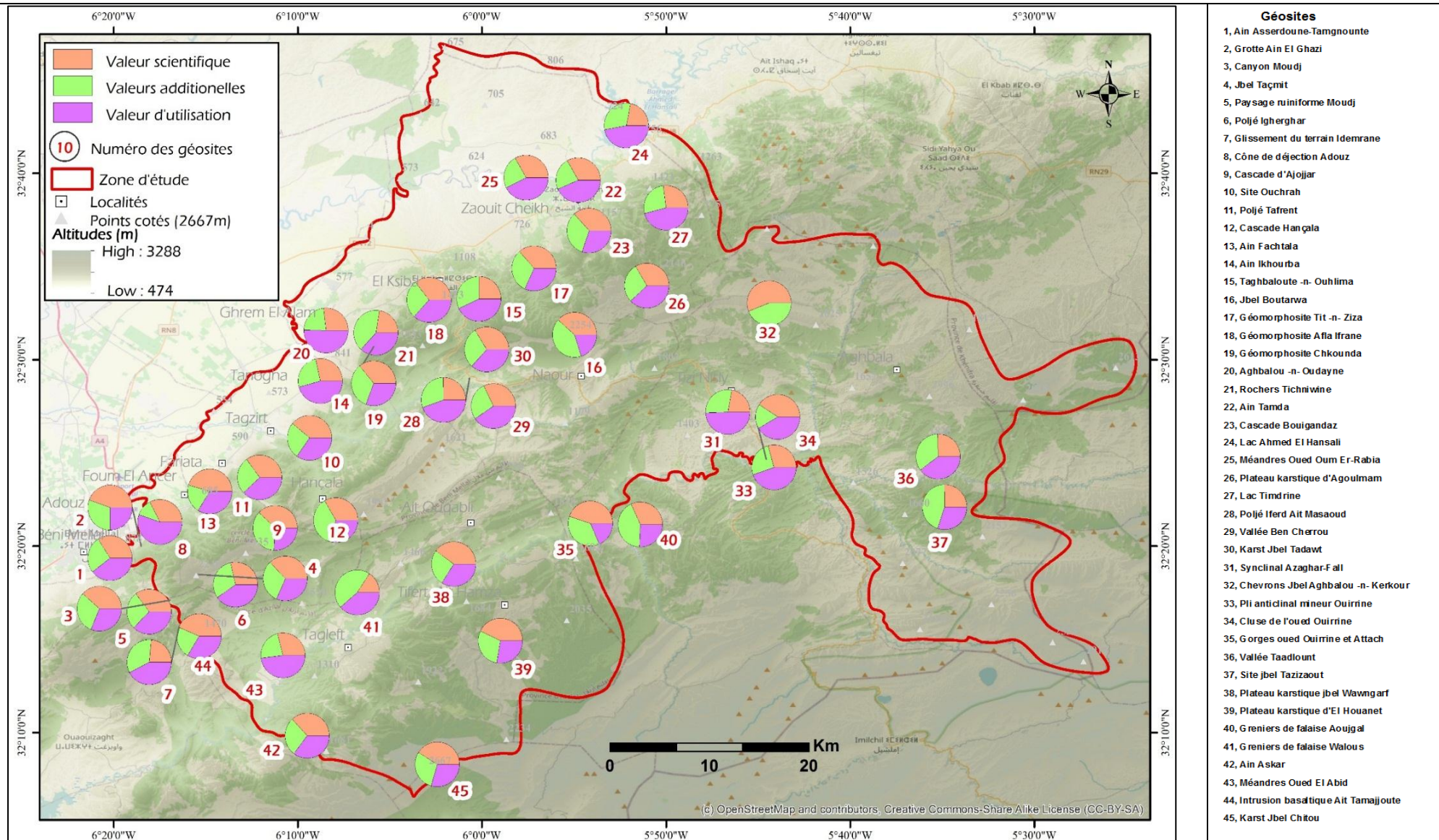
Figure 93: Scores des valeurs scientifique, additionnelle et d'utilisation des géopatrimoines étudiés
