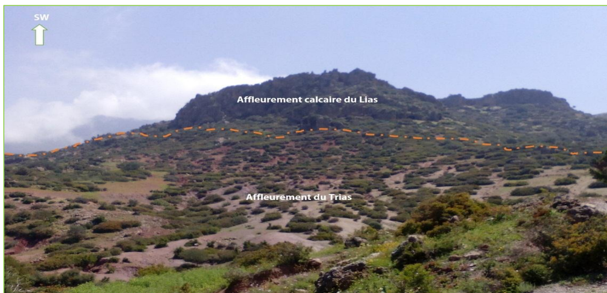
Photo 2: Trias affleure à la surface donnant naissance à l'émergence d'Anoufi (Tanougha) (Ait Omar, 2018)
