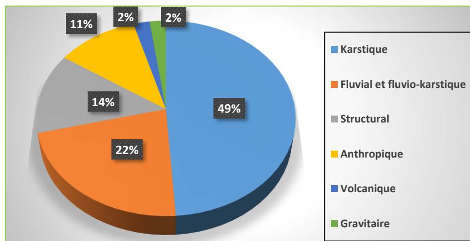
Figure 57: Les géopatrimoines retenus par processus
