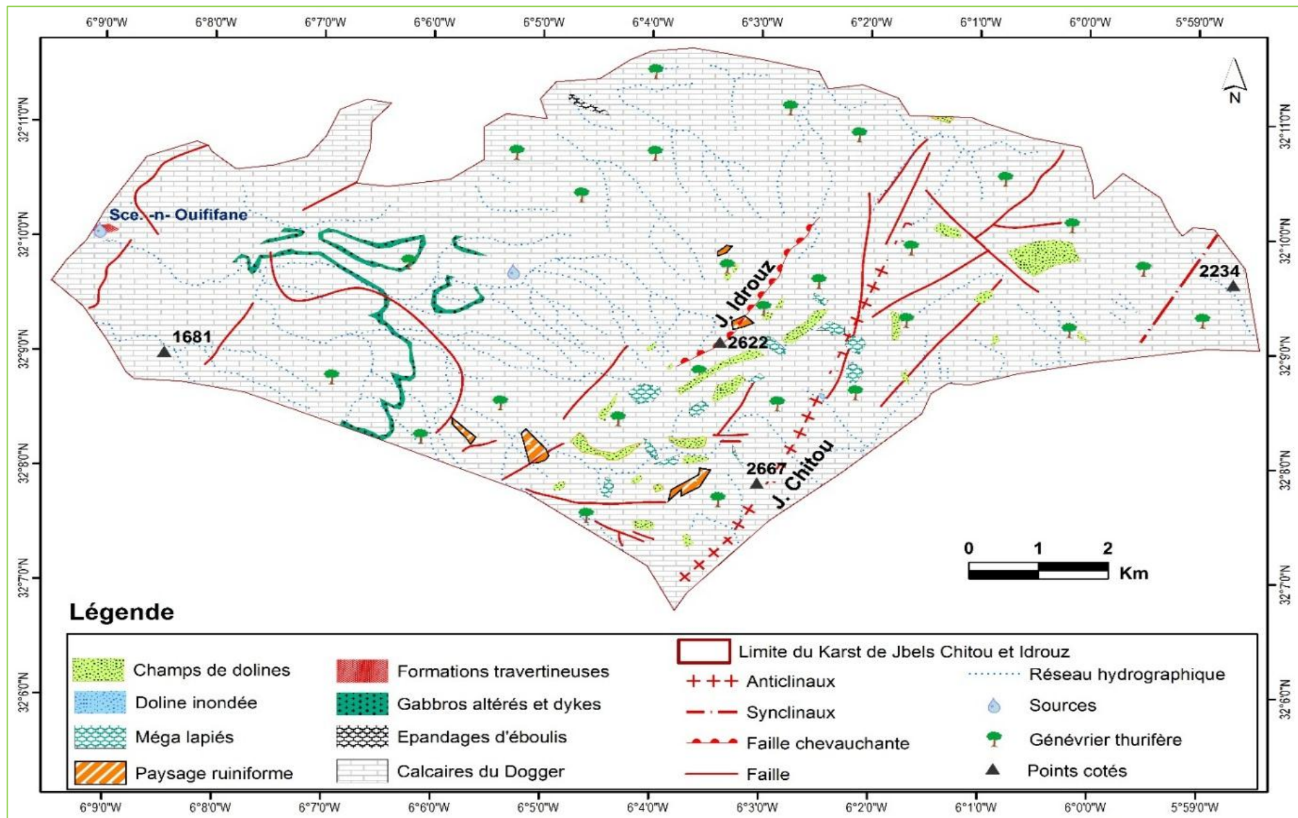
Figure 24: Carte géomorphologique simplifiée du karst de Jbels Chitou et Idrouz (Carte géologique de Béni Mellal, 1/100000, carte topographique de Tilouguite, 1/50000 et image Google Earth, 2020)
