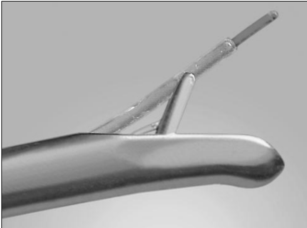
Figure N°87: Gaine protectrice d'un laser endoscopique Karl Storz. Le mécanisme de direction de l'extrémité du laser est visible [32].
