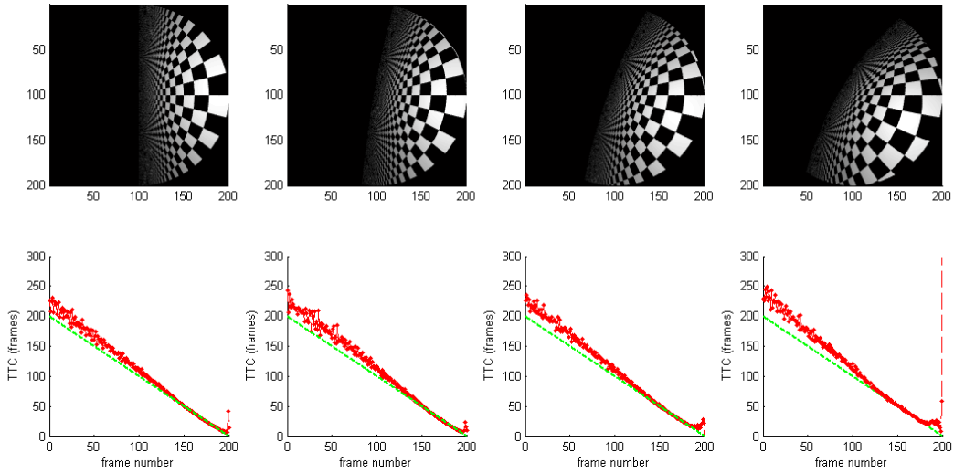
FIGURE 5.4 – Estimation du TAC. La première rangée montre respectivement l'image n^{\circ}1 des séquences seq1, seq2, seq3 et seq4 présentées dans le tableau 5.3. La deuxième ligne montre la courbe du TAC estimé (en rouge) et la vérité terrain (en vert) pour chaque séquence.
