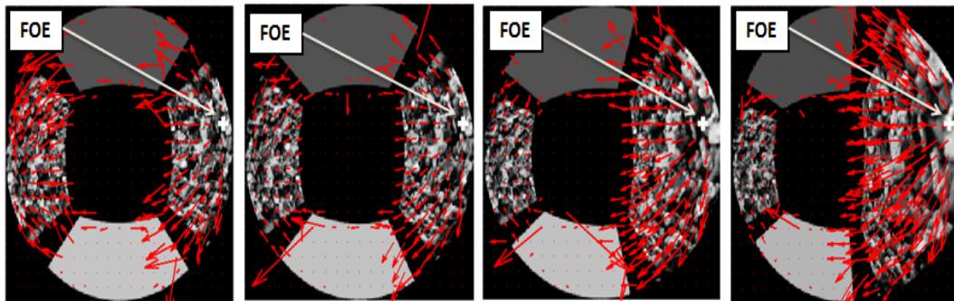
FIGURE 5.29 – Les vecteurs de flot optique estimés et la position du FOE sur les quatre images de la séquence de la figure 5.28.
