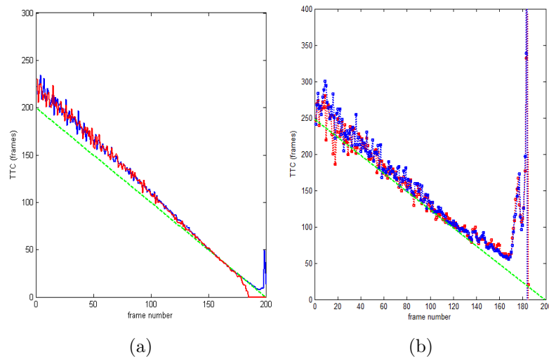
FIGURE 5.35 – Comparaison entre les deux approches locale et globale de calcul du TAC. La Courbe rouge montre l'estimateur du TAC calculé à partir de la MLFO et la courbe bleue l'estimateur du TAC calculé à partir de la MGG. (a) comparaison dans le cas de la séquence de synthèse. (b) Comparaison dans le cas de la séquence réelle.
