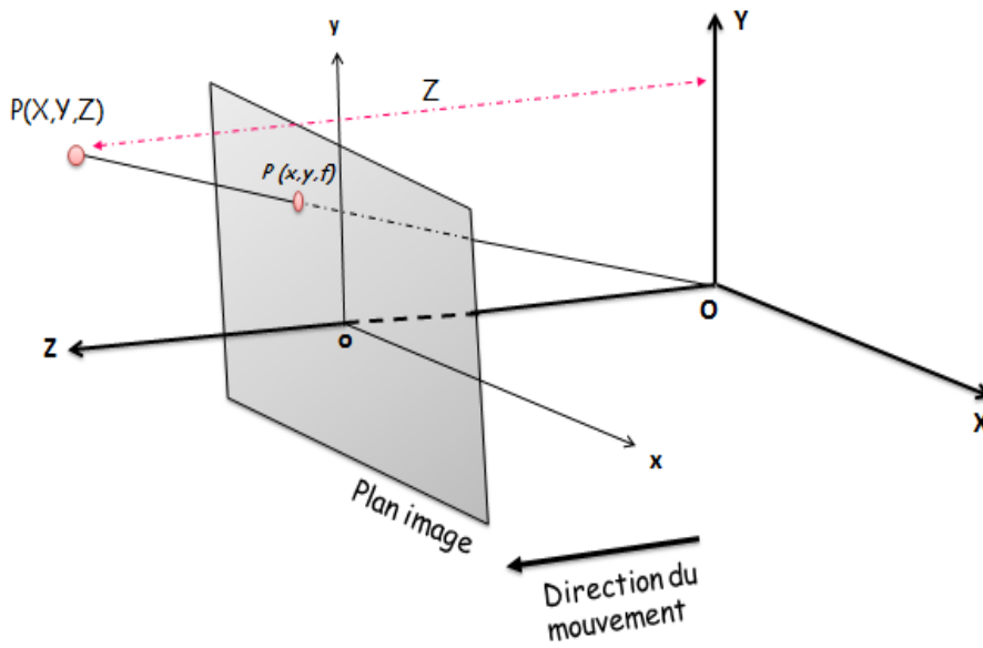
FIGURE 3.9 – Configuration géométrique dans le cas perspectif.
