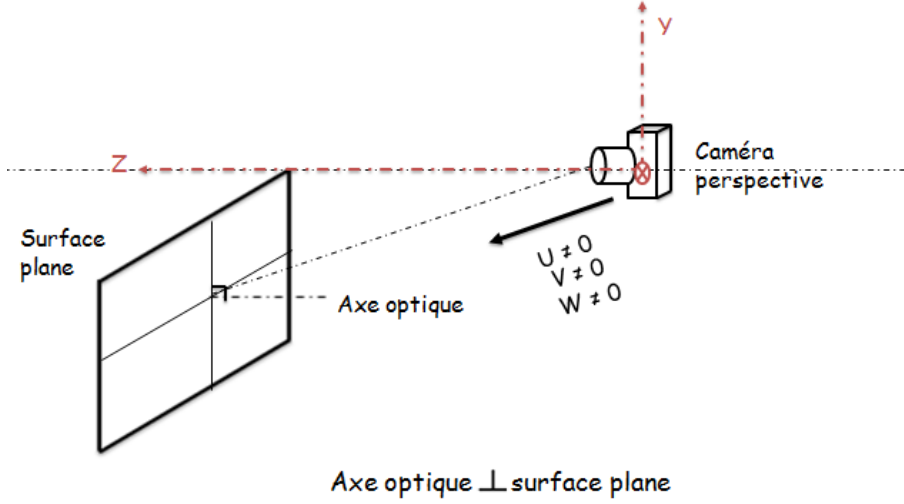
FIGURE 3.15 – Cas 2 : Translation arbitraire de la caméra relativement à une surface plane perpendiculaire.
