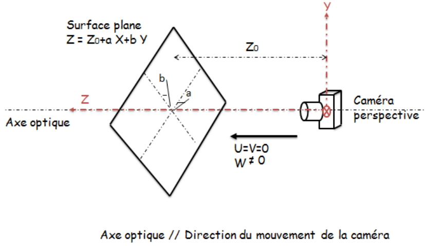
FIGURE 3.16 – Cas 3 : Translation de la caméra suivant l'axe optique relativement à une surface plane d'orientation quelconque.
