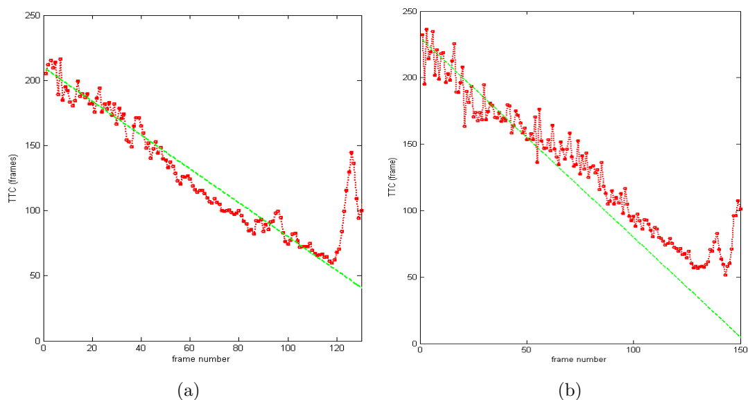
FIGURE 5.10 – Estimation du TAC dans le cas réel pour les séquences décrites dans la table 5.4, la courbe rouge fournit l’estimation du TAC et la courbe verte correspond à la vérité terrain : (a) TAC estimé pour la seq 11, (b) TAC estimé pour la seq 12.
