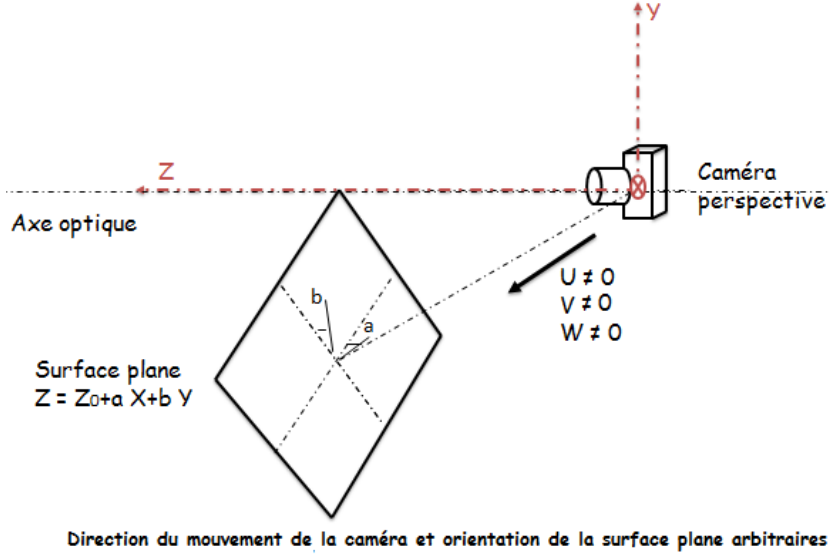
FIGURE 3.17 – Cas 4 : Translation arbitraire de la caméra relativement à une surface d'orientation quelconque
