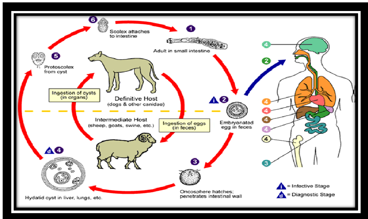
Fig. 14 : Le cycle de vie de l'Echinococcus granulosus.
