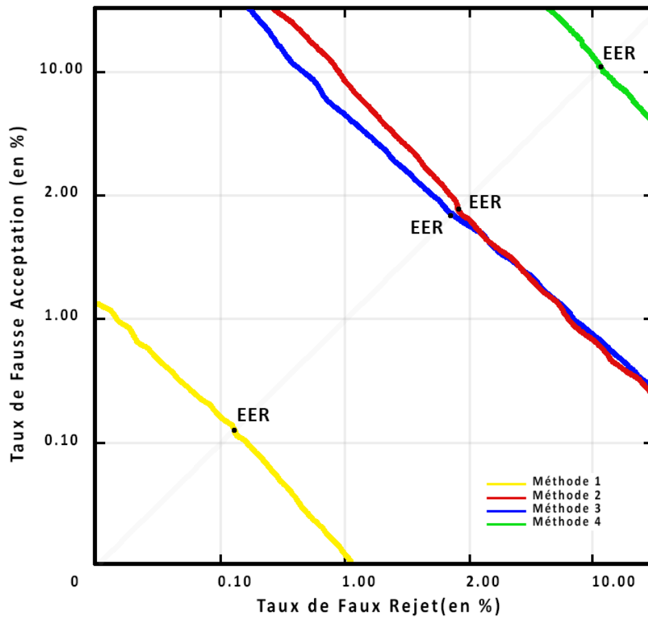
Figure 1.5: Le compromis d'erreur de détection d'échantillon (DET) représentant la performance de quatre techniques de vérification automatique du locuteur.
