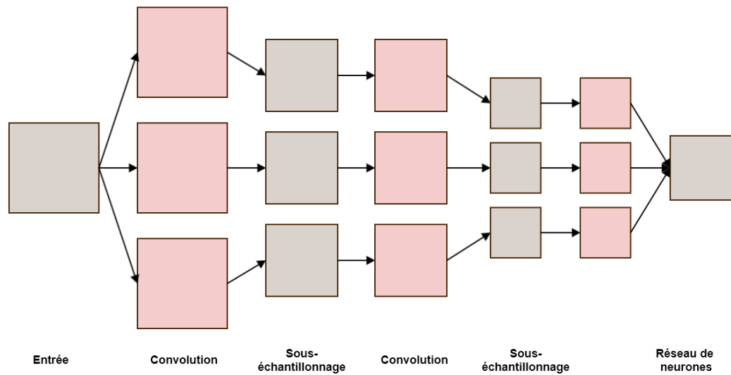
Figure 2.9: Un schéma conceptuelle du réseau de neurones convolutif en utilisant trois filtres.
