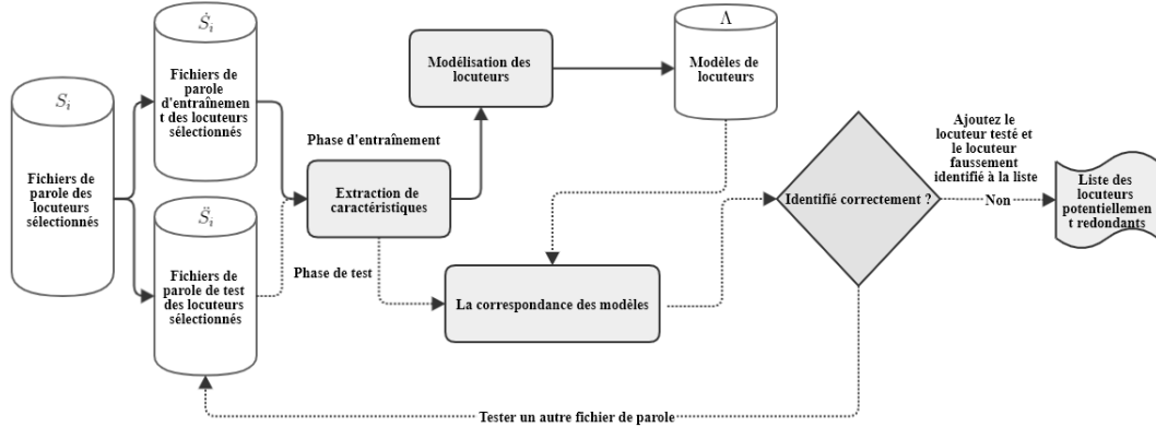
Figure 3.2: Un organigramme du processus d'identification automatique des locuteurs potentiellement redondants.
