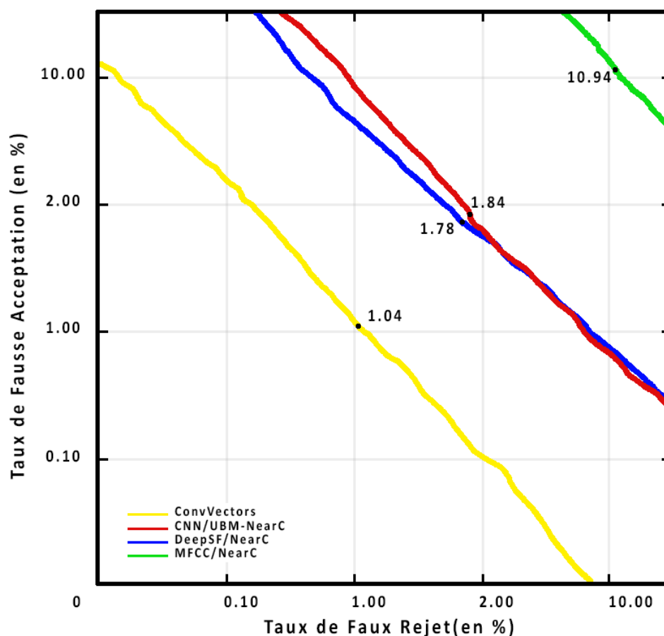
Figure 4.4: Le compromis d'erreur de détection d'échantillon (DET) représentant la performance des méthodes proposées: MFCC/NearC, DeepSF/NearC, CNN/UBM-NearC et ConvVectors.
