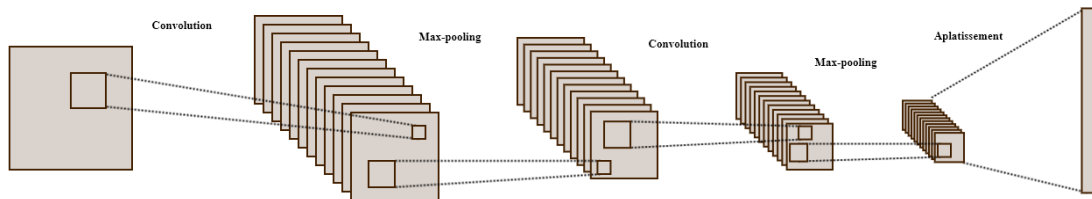
Figure 7.3: Illustration de la structure du réseau de neurones convolutif, elle se compose de : couche d'entrée (à gauche), couches de convolution, couches de sous-échantillonnage, et une couche entièrement connectée (à droite).
