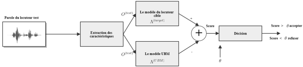
Figure 1.3: La procédure d'évaluation du modèle GMM/UBM pour la tâche de vérification automatique du locuteur.
