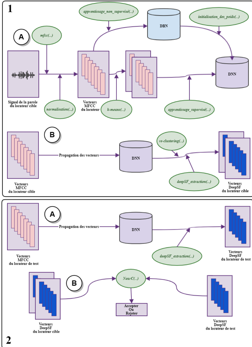
Figure 5.1: Le schéma de la méthode proposée. La phase (1) est la phase d'entraînement, la phase (2) est la phase de test.
