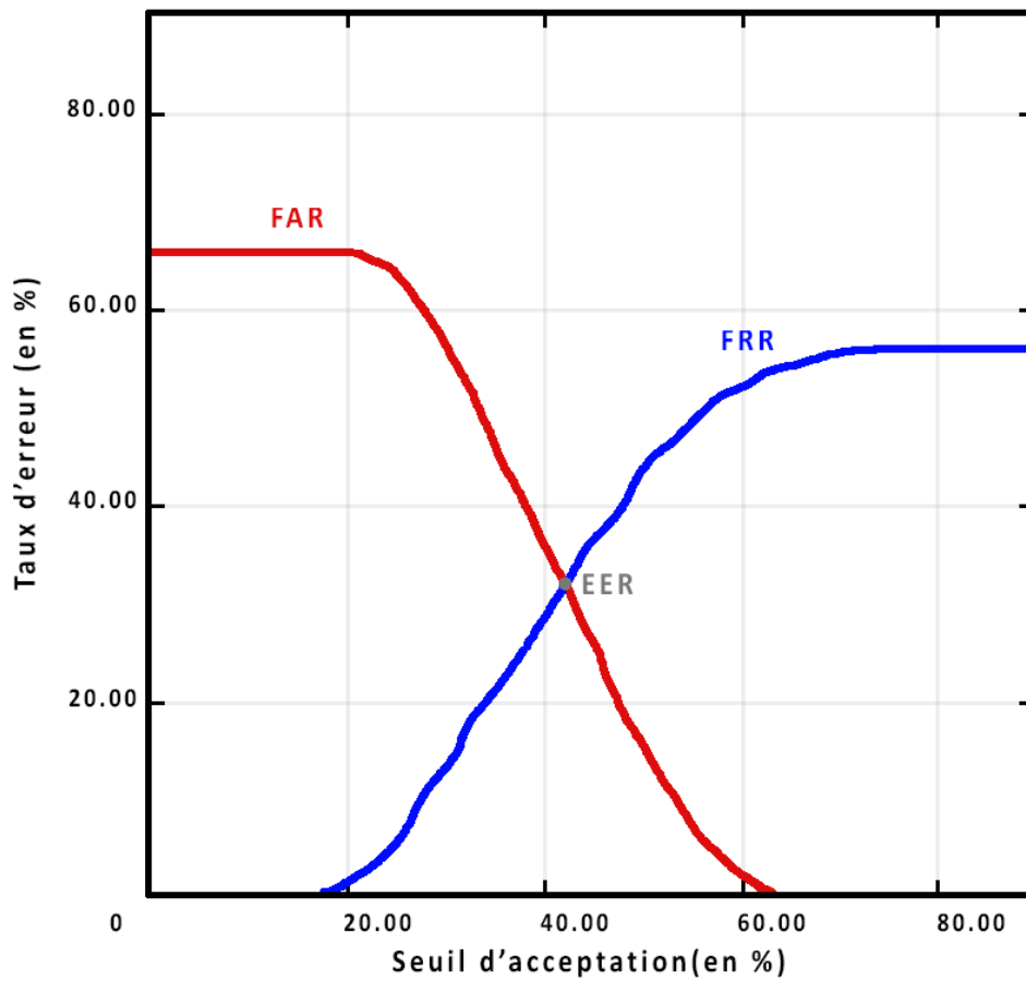
Figure 1.4: Illustration du point d'intersection des courbes FRR et FAR.
