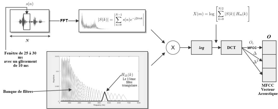
Figure 1.2: Le processus d'extraction d'un vecteur MFCC à partir d'une trame de parole. Voir Eq. 1.1 et Eq. 1.2 pour o_i et o , respectivement.
