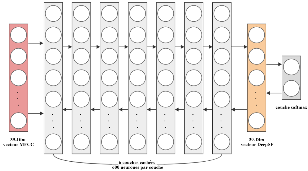
Figure 5.2: L'architecture du réseau de neurone profond (DNN) utilisé dans la méthode proposée.
