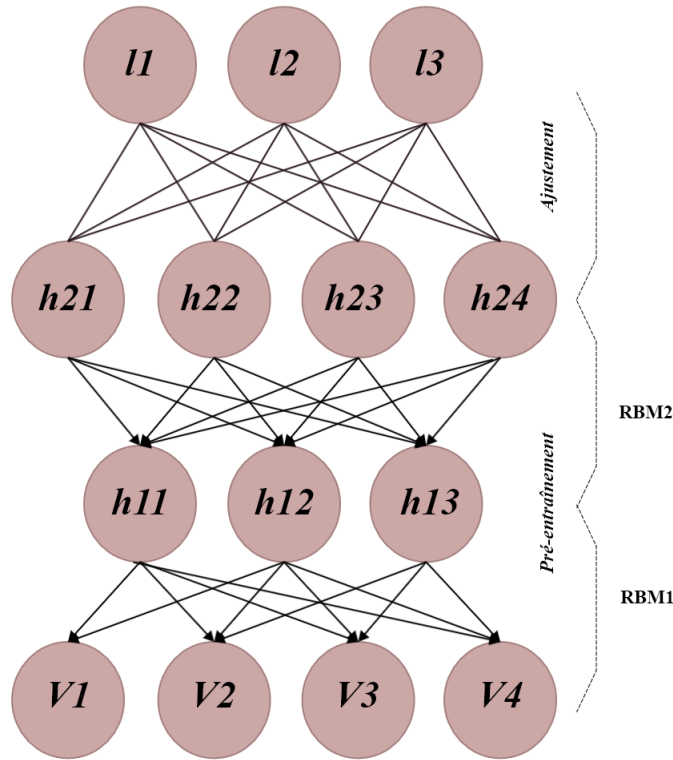
Figure 2.7: Un schéma conceptuelle du réseau de croyance profond.
