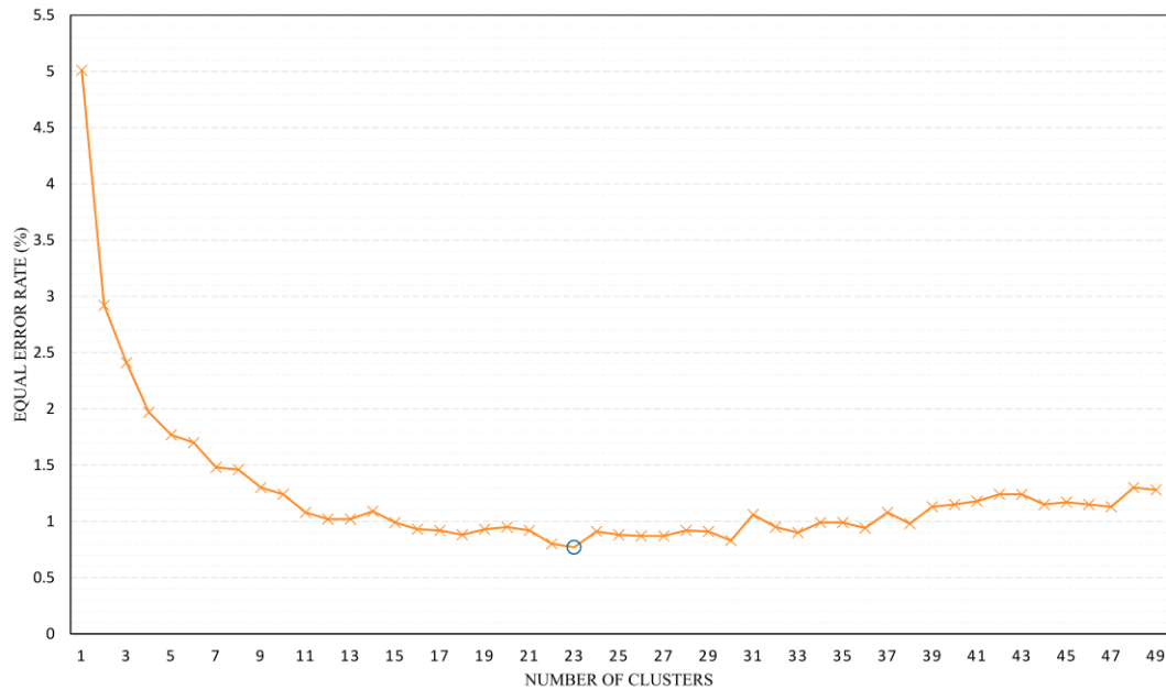
Figure 4.1: Méthode (iii): MFCC/NearC, Le taux d'erreur égal est tracé par rapport au nombre de clusters sur le corpus THUYG / locuteurs féminins, le EER minimal est de 0,77% pour k = 23 (point entouré d'un cercle).
