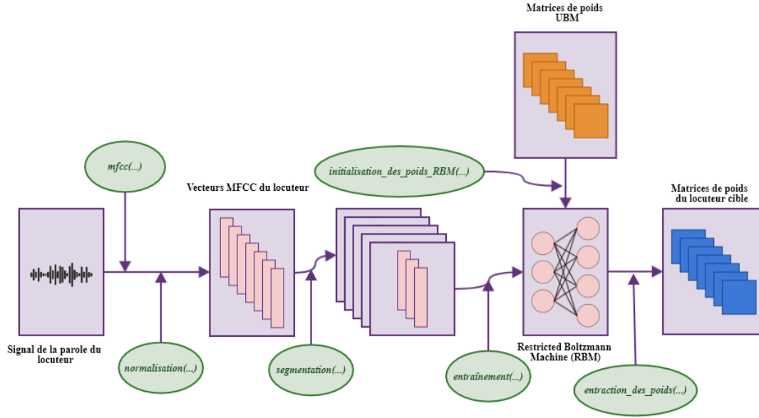
Figure 6.2: Processus de génération des matrices du locuteur cible.
