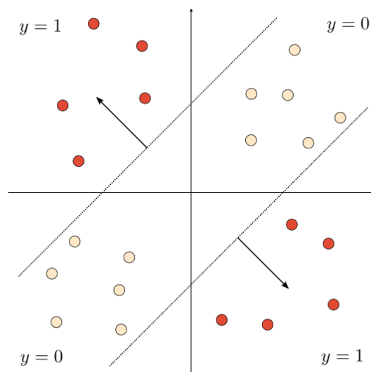
Figure 2.5: Une illustration de l'incapacité d'une seule ligne (c'est-à-dire un perceptron) à classer correctement la fonction XOR. Au lieu de cela, la composition de deux lignes est nécessaire pour séparer correctement ces échantillons, c'est-à-dire plusieurs couches.
