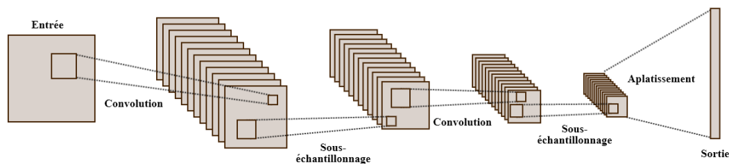
Figure 2.8: Un schéma du réseau de neurones convolutif. (La profondeur des matrices représente le nombre de filtres utilisés. La taille du vecteur de sortie est déterminé après l’aplatissement des matrices de la couche précédente et la concaténations des vecteurs résultants.)
