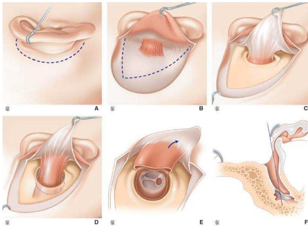
Figure 38 : Voie rétroauriculaire [13]
