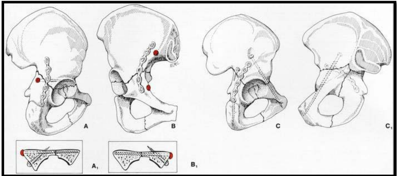
Figure 61 : Différents types d'ostéosynthèse des fractures en T
