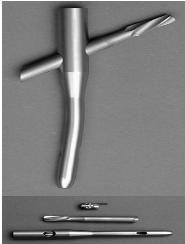
Figure 66 : clou TFN de fixation trochantérienne (170 mm) avec ses composantes à savoir le mécanisme anti rotatif, la lame spiralée et le clou (62).
