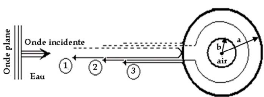
Fig III.2 Mécanisme de la formation des échos (1 : Echo spéculaire, 2 : Ondes circonférentielles, 3 : Onde de Sholte)
