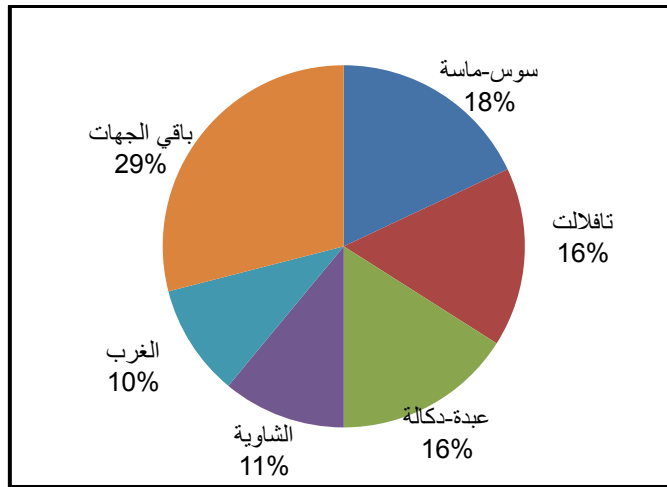
شكل رقم 2: توزيع استهلاك الأسمدة حسب المجالات الفلاحية.
