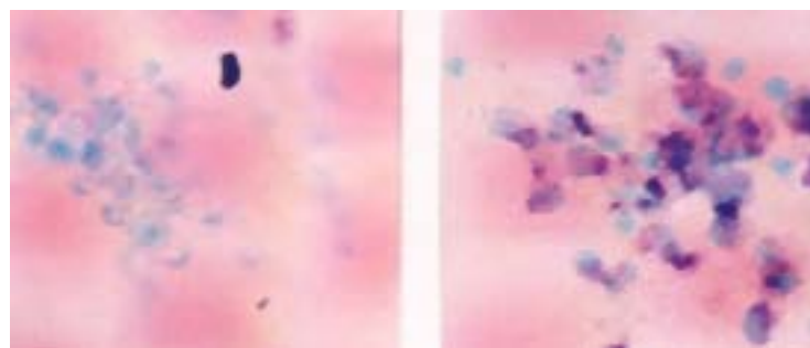
Figure 27: le NBT test: Les PN normaux sont activés et l'O 2- généré réduit le NBT en pigment bleu-violet, le test alors est positif. Lorsque les cellules génèrent peu ou pas d'O 2- elles restent incolores
