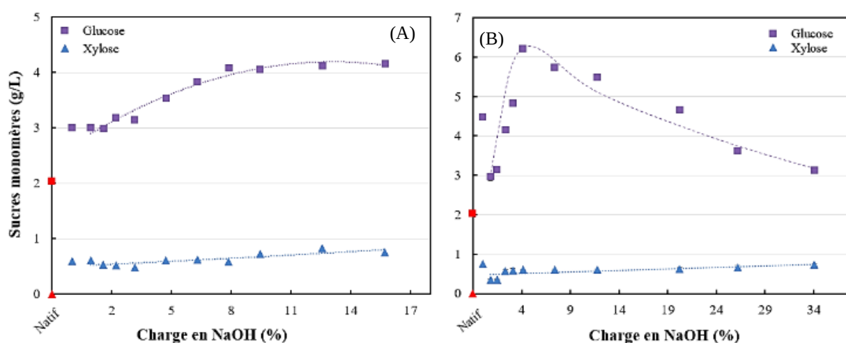
Figure 98 : Concentrations en sucres monomères présents dans l'hydrolysate de la chènevotte prétraitée en conditions alcalines. Imprégnation de l'agent chimique par aspersion (A) ou immersion (B)
