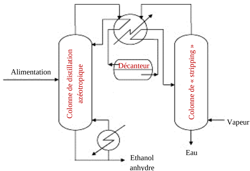
Figure 38 : Schéma du procédé de distillation azéotropique (Kumar et al., 2010)
