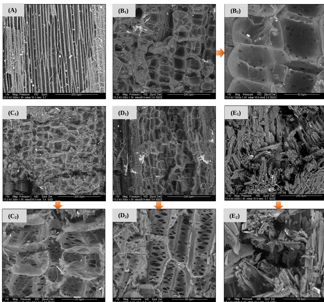
Figure 75 : Images par MEB à deux grossissements de la chènevotte prétraitée ; Imprégnation par immersion à différentes concentrations en acide sulfurique : natif à X300 (A), 0,6% à X300 (B 1 ) et X1000 (B 2 ), 1% à X300 (C 1 ) et X1000 (C 2 ), 2% à X300 (D 1 ) et X1000 (D 2 ), 3% à X300 (E 1 ) et X1000 (E 2 )
