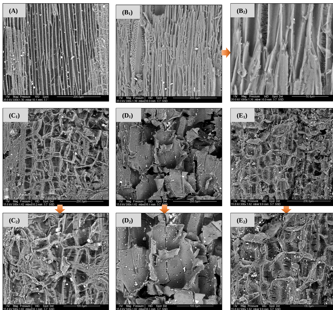
Figure 80: Images par MEB à deux grossissements de la chènevotte prétraitée ; imprégnation par aspersion à différentes concentrations en hydroxyde de sodium : natif à X300 (A), sans agent alcalin (0%) à X300 (B 1 ) et X500 (B 2 ) ; 10% à X300 (C 1 ) et X500 (C 2 ) ; 20% à X300 (D 1 ) et X500 (D 2 ) ; 30% à X300 (E 1 ) et X500 (E 2 )
