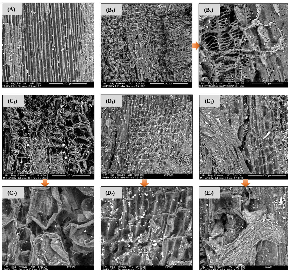
Figure 81: Images par MEB à deux grossissements de la chènevotte prétraitée ; Imprégnation par immersion à différentes concentrations en hydroxyde de sodium : natif à X300(A) ; 0,6% X300 (B1) et X1000 (B2) ; 1% à X300 (C1) et X1000 (C2) ; 2% à X300 (D1) et X1000 (D2) ; 3% à X300 (E1) et X1000 (E2)
