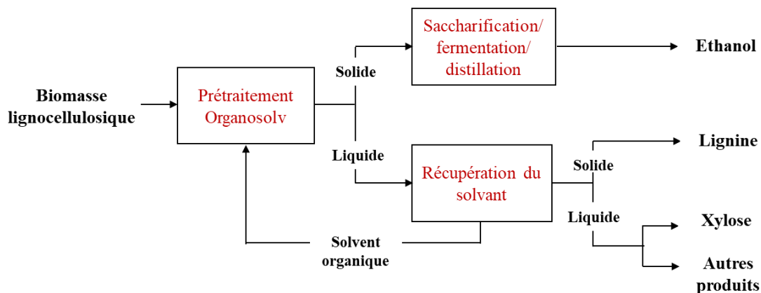
Figure 26 : Schéma du procédé Organosolv (Zhang et al., 2016)
