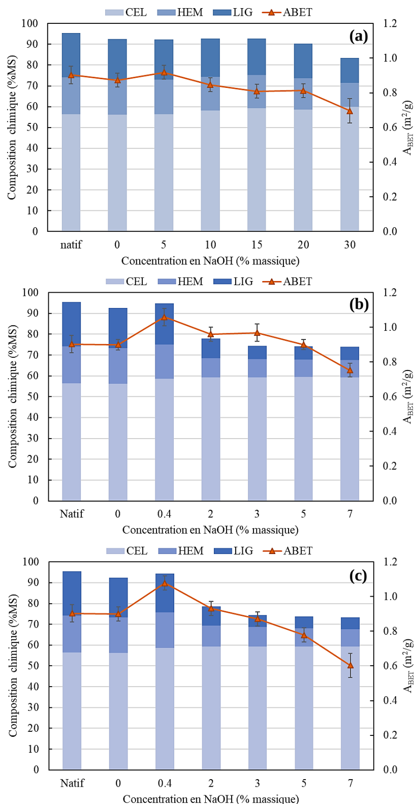
Figure 77 : Variation de la composition chimique et de la surface spécifique de la chènevotte imprégnée par de l'hydroxyde de sodium à différentes concentrations par aspersion (a) et immersion pendant 10 min (b) et 30 min (c) et prétraitée par DIC.
