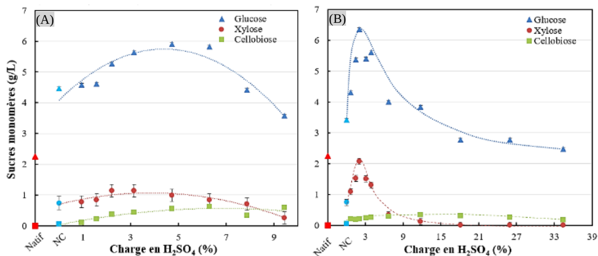
Figure 94 : Concentrations en sucres monomères présents dans l'hydrolysats de la chènevotte prétraitée en conditions acides, après imprégnation par aspersion (A) et immersion (B)
