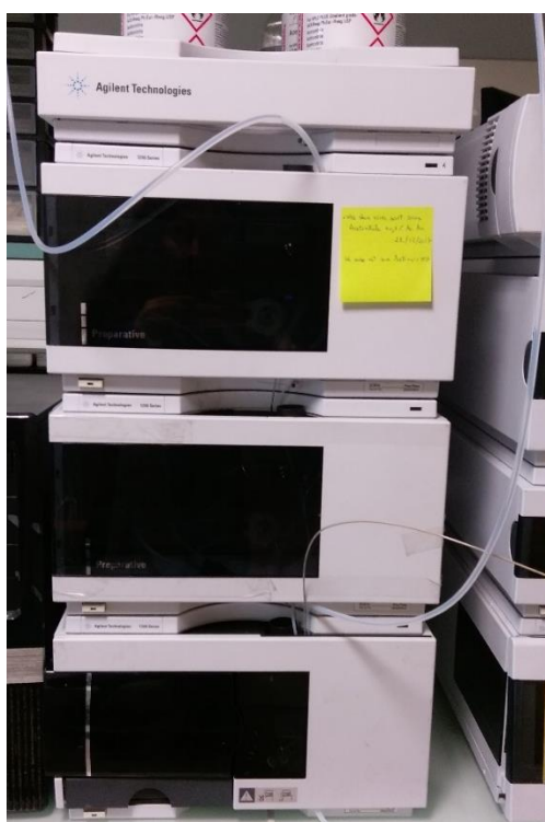
Figure 62 : Système HPLC
