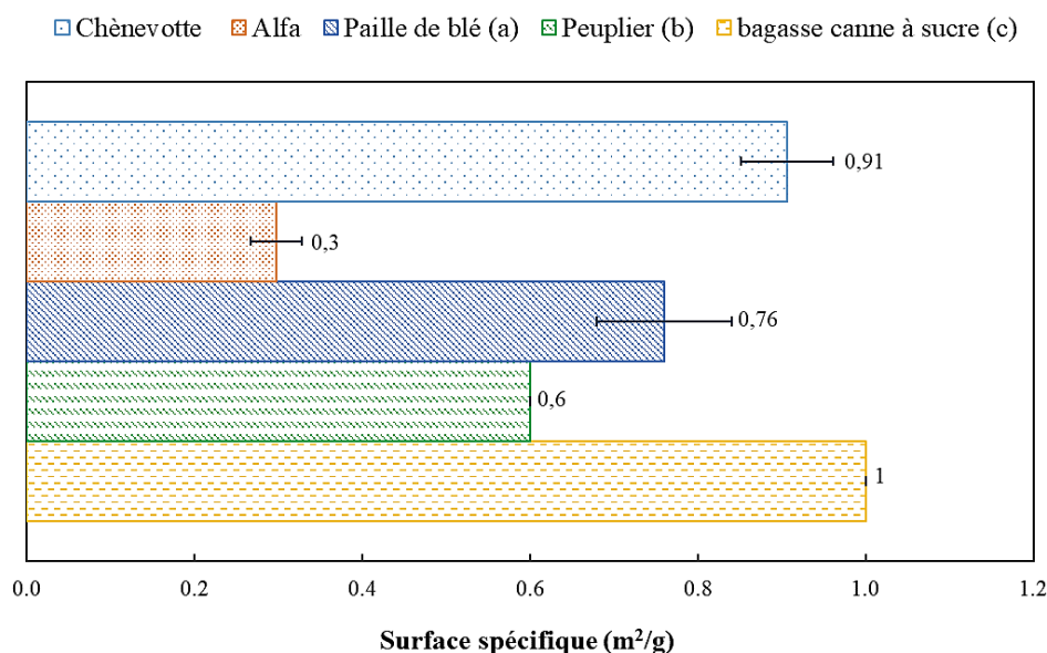
Figure 68 : Surface spécifique des deux substrats étudiés en comparaison avec d'autres matières lignocellulosiques. Intervalle de la taille des particules : (a) : 1-8 mm (Maache-Rezzoug et al., 2015), (b) : 0,15-0,5 (Nitsos et al., 2013) et (c) : \geq 0,42 mm (Wei Hsin Chen et al., 2011).
