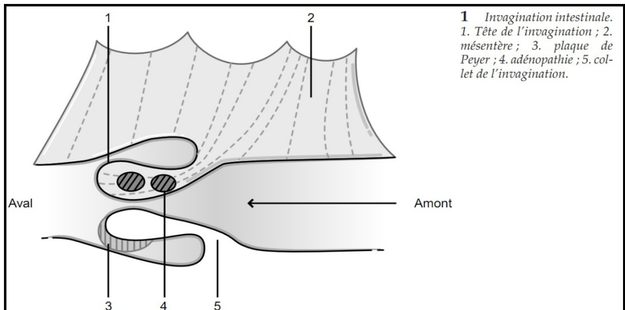
Figure 15: boudin d'invagination [24].
