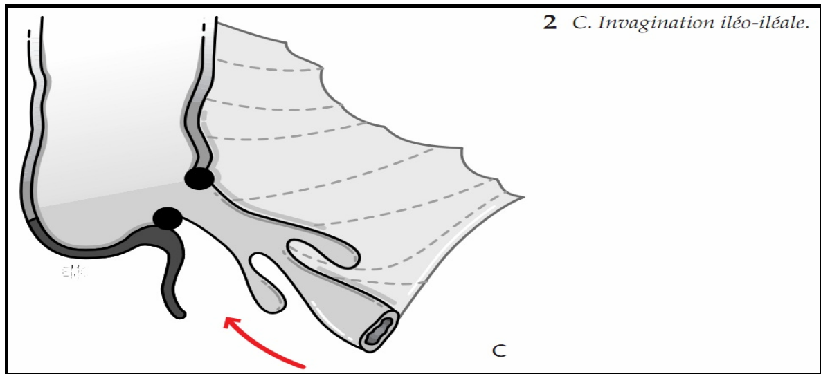
Figure 17:invagination iléo-iléale [24].
