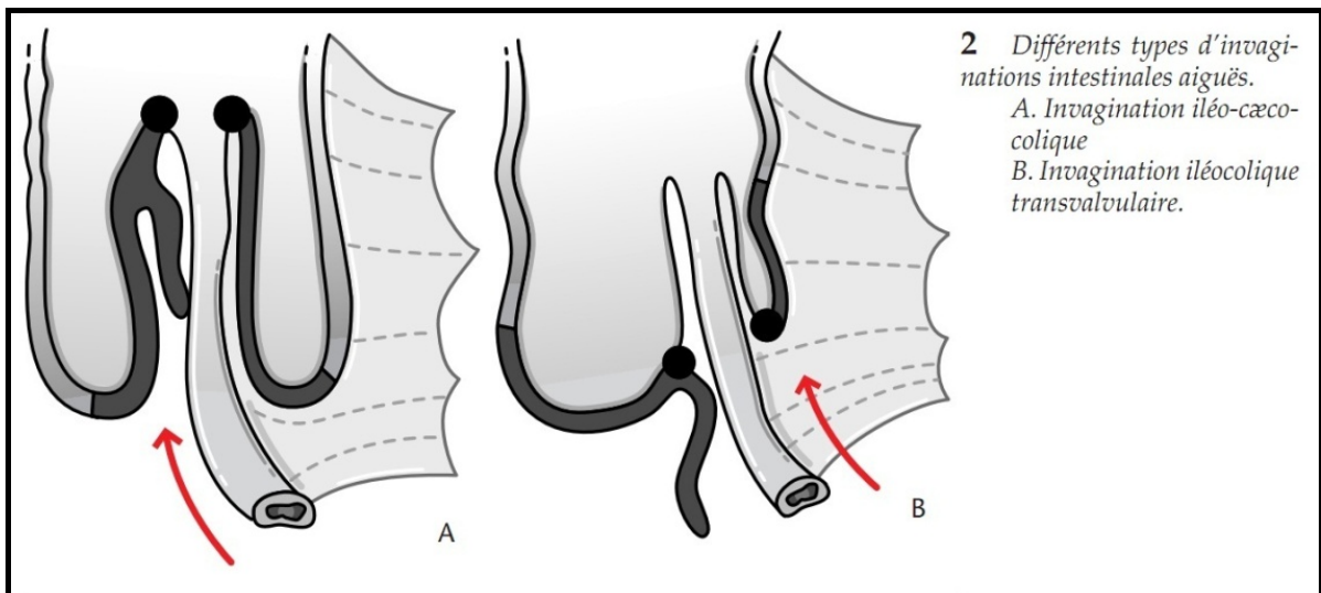
Figure 16 : invagination iléocolique [24].
