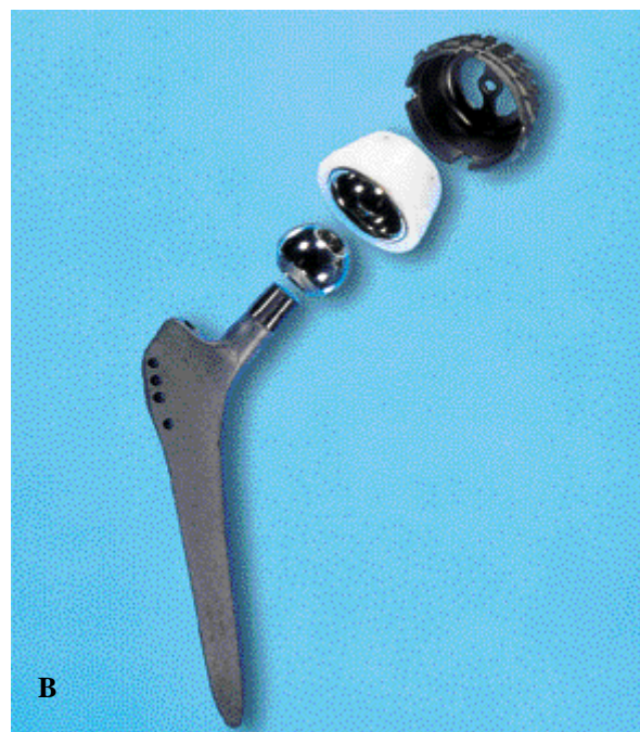
B. Prothèse totale de hanche modulaire à fixation hybride et couples de frottement optionnels
