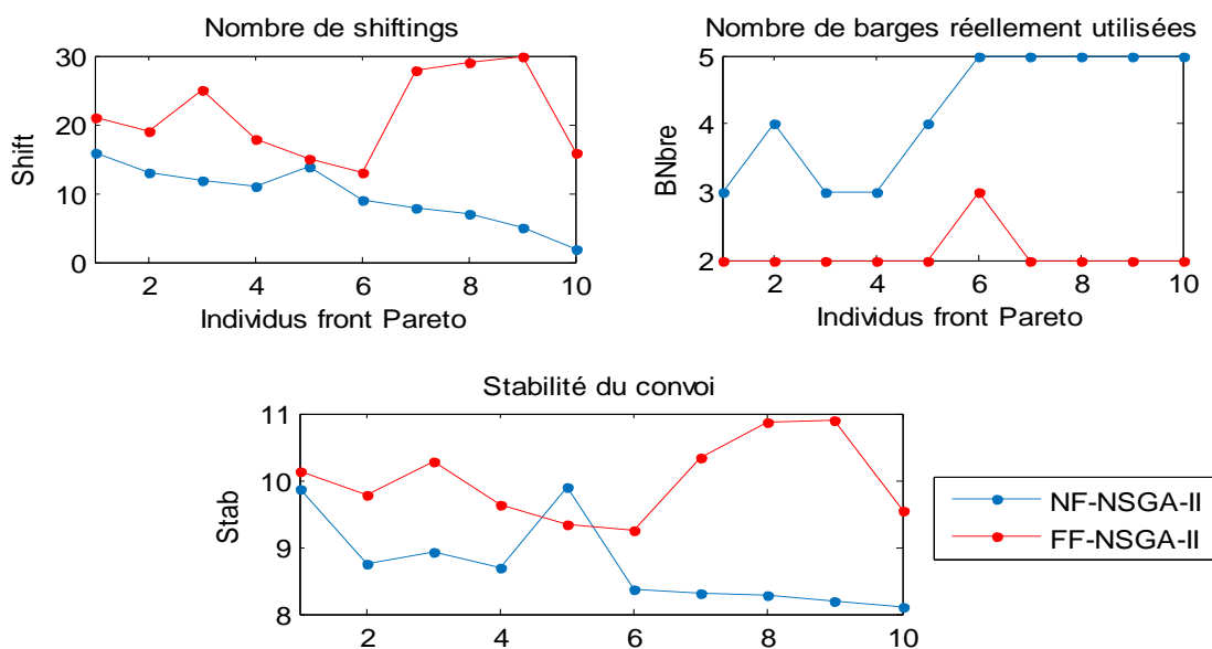
Figure IV-26. Comparaison entre NF-NSGA-II et FF-NSGA-II selon les valeurs de chaque fonction objectif
