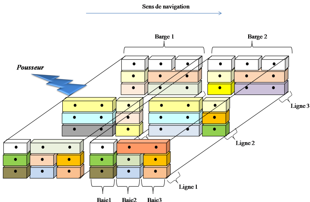
Figure IV-2. Exemple d'un convoi poussé de deux barges homogènes de capacité 27 EVP totalement remplies
